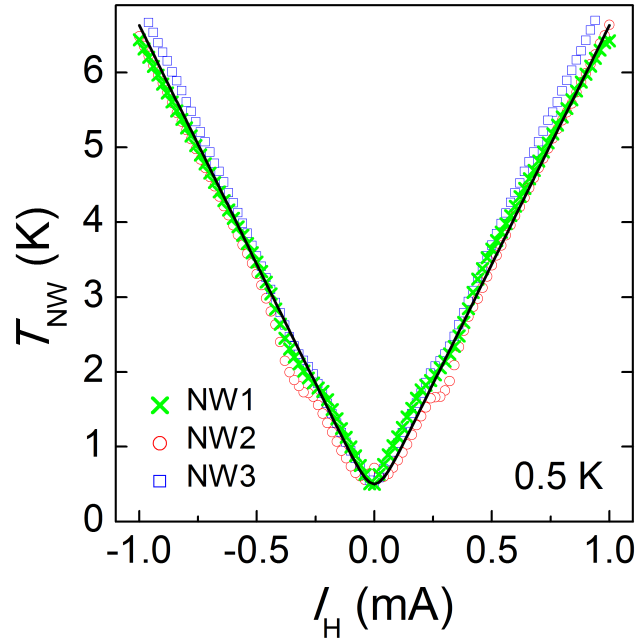
Рис. 6.4: Измерение локального шума при температуре T_0 = 0.5 К. Измеренная шумовая температура нанопровода-сенсора в зависимости от тока I_H через контактную полоску в конфигурации 1 \rightarrow \perp для трех различных образцов (разные символы). Сплошная линия соответствует фермиевской функции распределения в точке «test end» с температурой, определенной в соответствии с (1.17), где V = r_H I_H при r_H = 3.6 Ом.
