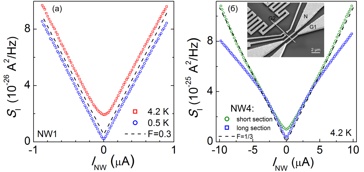
Рис. 6.2: Измерение дробового шума. (а) Спектральная плотность токового шума как функция тока в образце NW1 при двух различных температурах ванны. Различные символы соответствуют различным температурам. Наклон пунктирной прямой соответствует значению фактора Фано F = 0.3 , близкому к универсальному значению для металлических диффузионных проводников. (б) Спектральная плотность токового шума как функция тока в короткой (кружки) и длинной (квадраты) частях образца NW4. Геометрия образца NW4 приведена на вставке.
