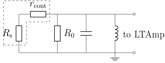
Рис. 2.11: Принципиальная схема измерения токового шума.
