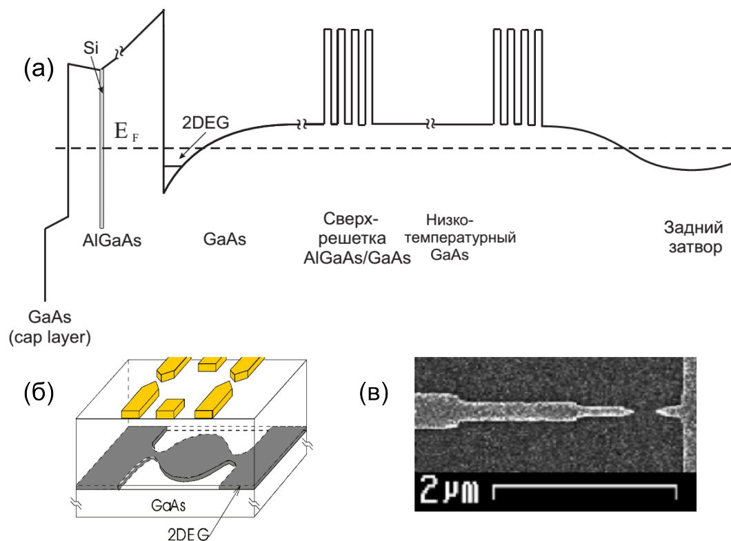
Рис. 2.1: (а) Схематическое изображение гетероструктуры GaAs/AlGaAs. (б) Схематическое изображение сформированной при помощи затворов квантовой точки. (в) Микрофотография одного из изучавшихся образцов (образец I из главы 3).
