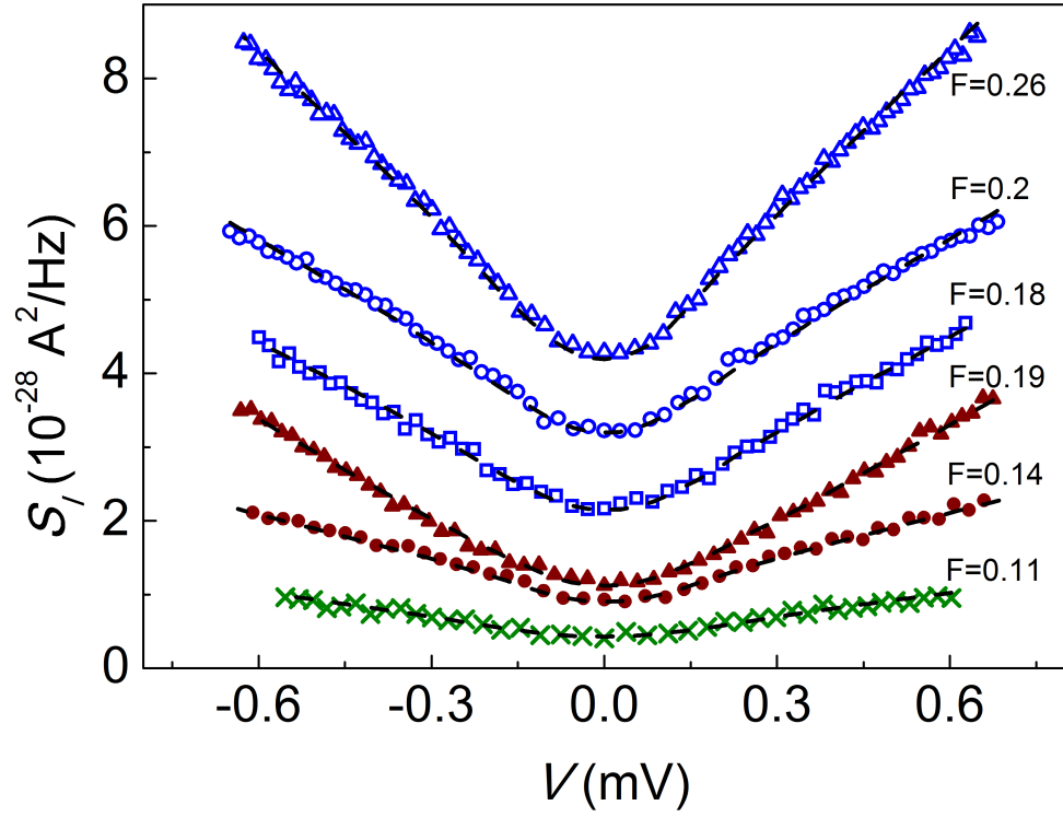
Рис. 5.10: Фактор Фано в режиме краевого транспорта в исследованных образцах. Символы – спектральная плотность дробового шума в области точки нейтральности как функция тянущего напряжения. Пунктирные линии – подгонки с использованием приблизительной формулы для сильно нелинейного режима (см. текст), использовавшиеся при этом значения F даны рядом с соответствующими кривыми. Открытые и закрытые символы отвечают образцам I и II соответственно, а кресты – образцу III. Те же символы отмечают соответствующие затворные напряжения V_g и значения сопротивления в режиме линейного отклика на рис. 5.6. Данные для образца I сдвинуты по вертикали на 3, 2 и 1 в единицах 10^{-28} \text{ A}^2/\text{Гц} (сверху вниз).
