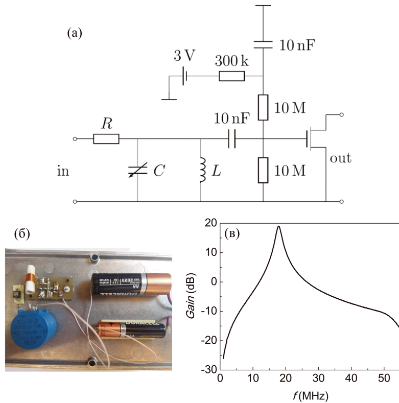
Рис. 2.8: Активный полосовой фильтр. (а) Схема активного фильтра. (б) Фотография фильтра. (в) Амплитудно-частотная характеристика.
