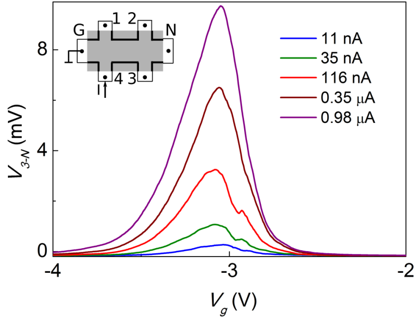
Рис. 5.8: Краевой транспорт в сильно нелинейном режиме.
