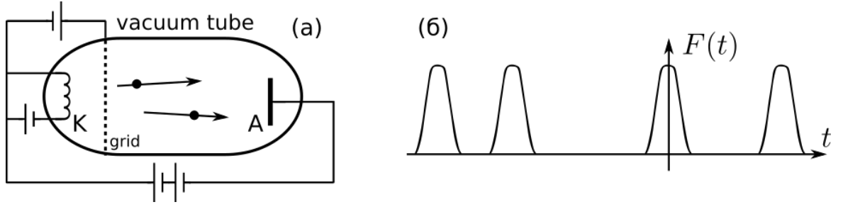
Рис. 1.3: (а) Схематическое изображение электронной лампы. (б) Ток через лампу как сумма единичных актов прилета электронов на анод.
