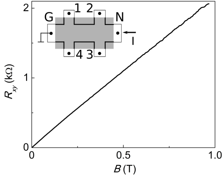
Рис. 5.5: Измерение холловского сопротивления (между контактами 1 и 4 в геометрии, изображенной на вставке) для одного из образцов при нулевом затворном напряжении.
