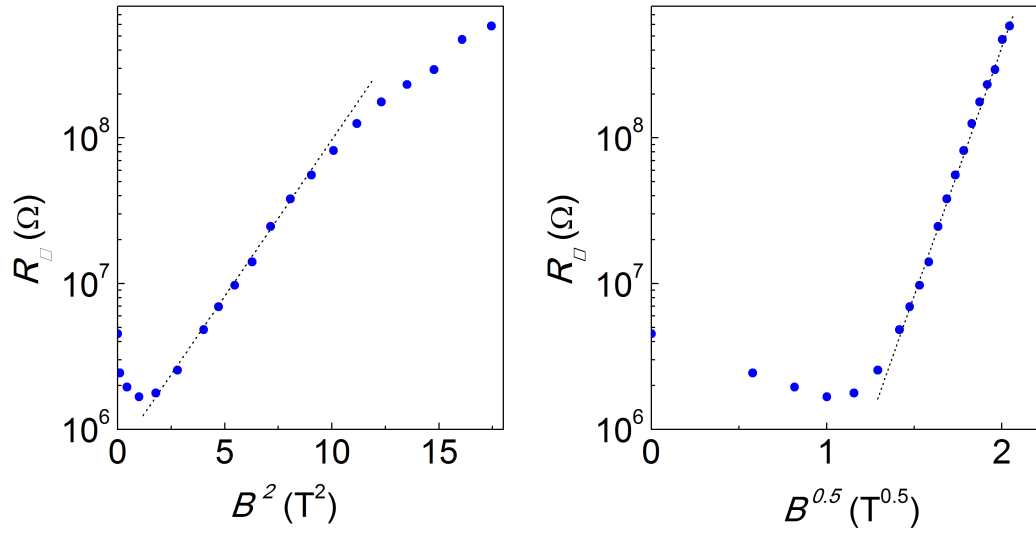
Рис. 4.5: Магнитосопротивление образца в различных координатах.
