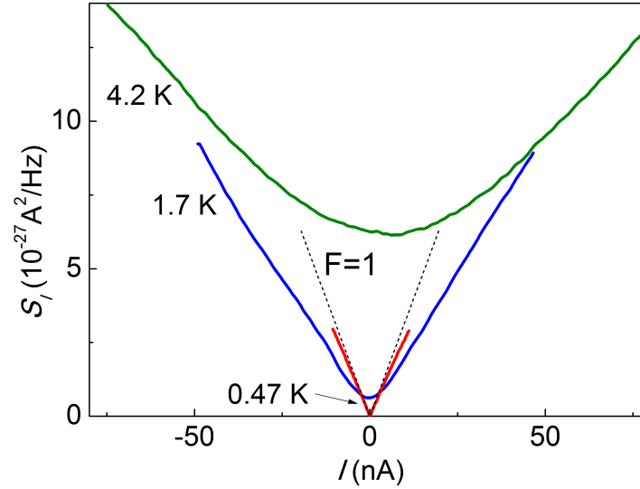
Рис. 4.7: Изменение фактора Фано с температурой. Сопротивление образца R_{\square} = 26 \text{ МОм} ( T = 0.47 \text{ K} ), T_0 \approx 300 \text{ K} . Пунктирная линия соответствует значению F = 1 .
