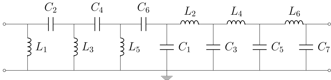
Рис. 2.6: Пассивный полосовой фильтр.
