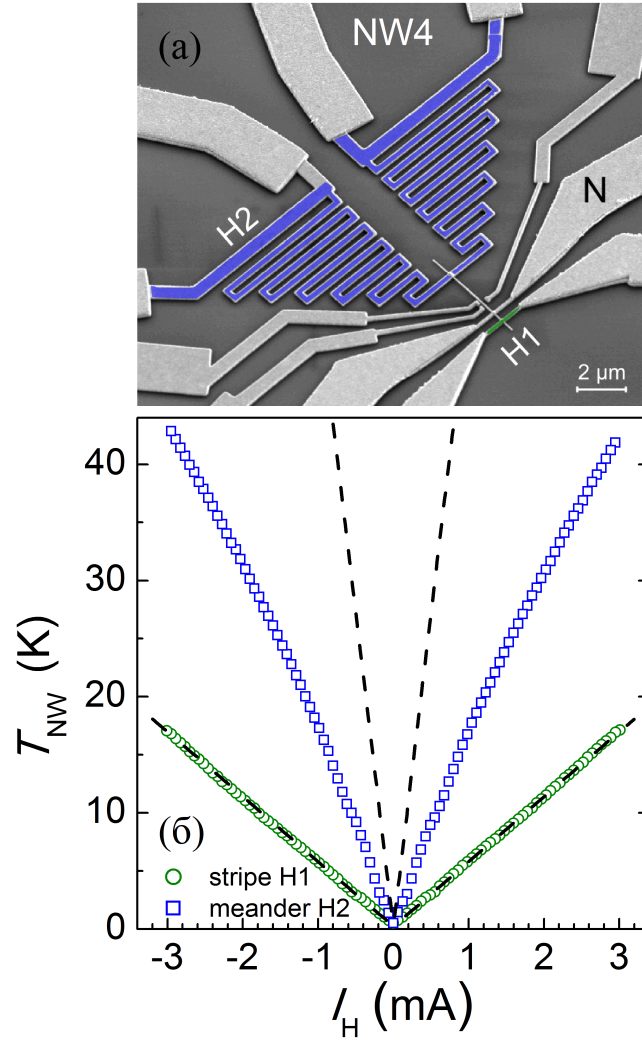
Рис. 6.5: (а) Микрофотография образца NW4. (б) Измерение локального шума при температуре T_0 = 0.5 К. Измеренная шумовая температура нанопровода-сенсора в зависимости от тока I_N через короткую контактную полосу Н1 (кружки) и меандр Н2 (квадраты) для образца NW4. Пунктирные линии соответствуют фермиевским функциям распределения в точке «test end» с температурами, определенными в соответствии с (1.17) при r_H = 3.1 Ом и r_H = 30 Ом соответственно.
