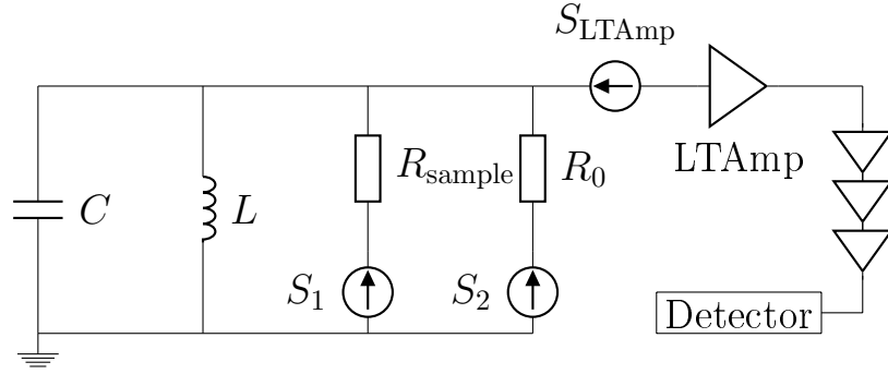
Рис. 2.9: Эквивалентный контур измерения токового шума в схеме с резонансным контуром. Образец R_{\text{sample}} , нагрузочное сопротивление R_0 = 3.3 \text{ кОм} , катушка L = 7 \text{ мкГн} и емкость кабеля C = 22 \text{ пФ} соединены в параллель на входе низкотемпературного усилителя. S_1, S_2, S_{\text{LTamp}} – токовые флуктуации образца, нагрузочного сопротивления и токовый шум усилителя, соответственно.
