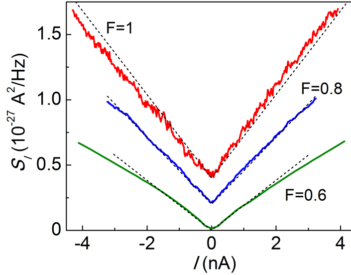
Рис. 4.6: Спектральная плотность дробового шума как функция тока при T = 0.56 К. Удельное сопротивление образца (температура Мотта) сверху вниз: R_{\square} = 58 МОм ( T_0 \approx 300 К), R_{\square} = 8.8 МОм ( T_0 \approx 140 К), R_{\square} = 1 МОм ( T_0 \approx 40 К). Пунктирные линии соответствуют наклону экспериментальных кривых в области линейной зависимости от тока. Масштаб по обеим осям уменьшен в 50(5) раз для нижней(средней) кривой. Две верхних кривых сдвинуты по вертикали на 2 и 4 \cdot 10^{-28} \text{ A}^2/\text{Гц} .
