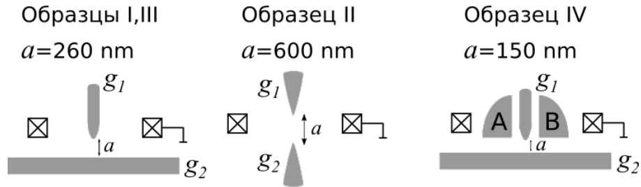
Рис. 3.9: Схематическое изображение изучавшихся образцов.
