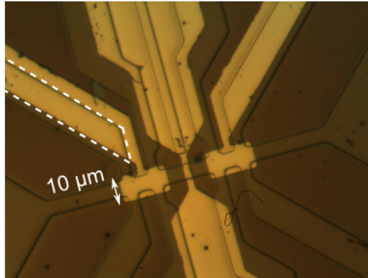
Рис. 5.4: Микрофотография одного из изучавшихся образцов. Пунктиром отмечена часть затвора над подводящей к рабочей части образца частью мезы, которая существенно увеличивает паразитную емкость образца.
