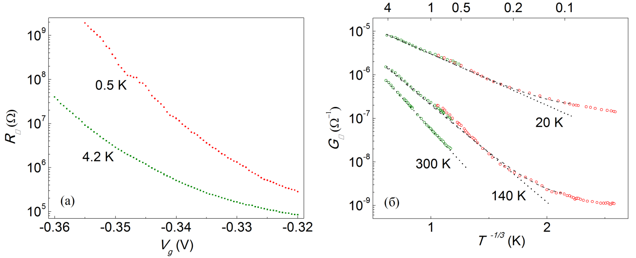
Рис. 4.3: Проводимость/сопротивление образца в линейном режиме. (а) Сопротивление образца как функция величины затворного напряжения V_g для двух различных температур. (б) Температурная зависимость проводимости по мере обеднения образца. Точками проведены линии, соответствующие моттовским температурным зависимостям. Подгонка температурных зависимостей с учетом низкотемпературных отклонений показана пунктирными линиями для указанных значений T_p (см. текст).
