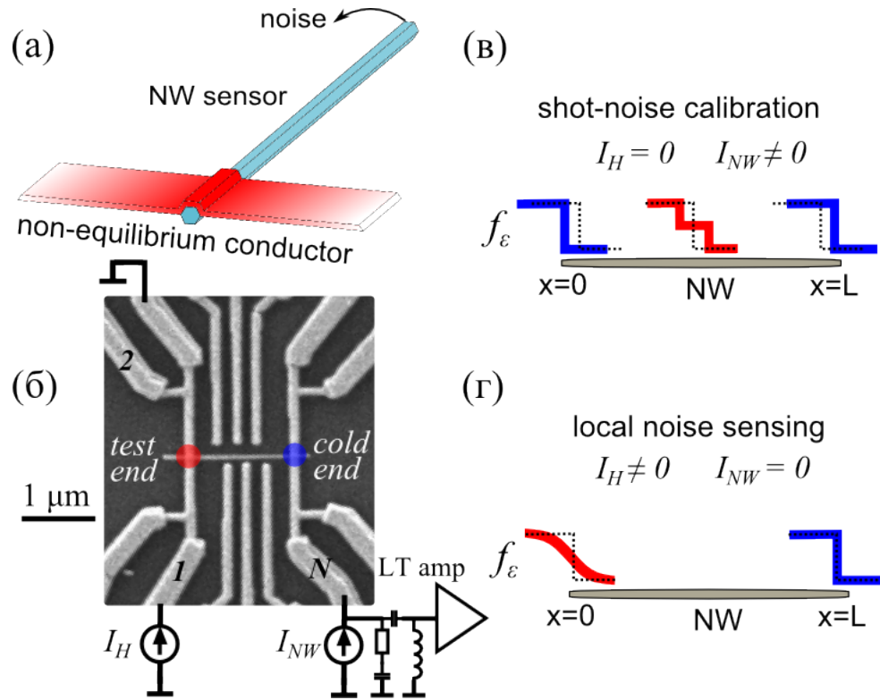
Рис. 6.1: Принцип локальной шумовой термометрии. (а) Локальный шумовой сенсор из нанопровода в контакте с исследуемым неравновесным проводником. Градиент цвета обозначает пространственную неоднородность электронной функции распределения в проводнике. (б) СЭМ-изображение одного из исследовавшихся образцов. Нанопровод и металлические части наноструктуры изображены светло-серым цветом. Красной и синей точками отмечены тестовый и противоположный холодный концы нанопровода. Показана также часть схемы на входе низкотемпературного усилителя и контур постоянного тока для создания неравновесной ситуации в левой контактной полоске. (в) и (г) Электронная функция распределения f_\epsilon в различных точках внутри нанопровода, соответствующая процедуре калибровки по дробовому шуму и локальному измерению шума (сплошные линии). Тонкие линии из точек соответствуют f_\epsilon в состоянии теплового равновесия. Для простоты тепловое размытие не отображено.
