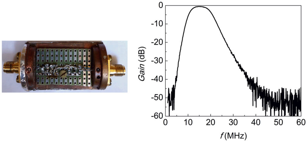
Рис. 2.7: Пассивный фильтр (слева) и его амплитудно-частотная характеристика (справа).
