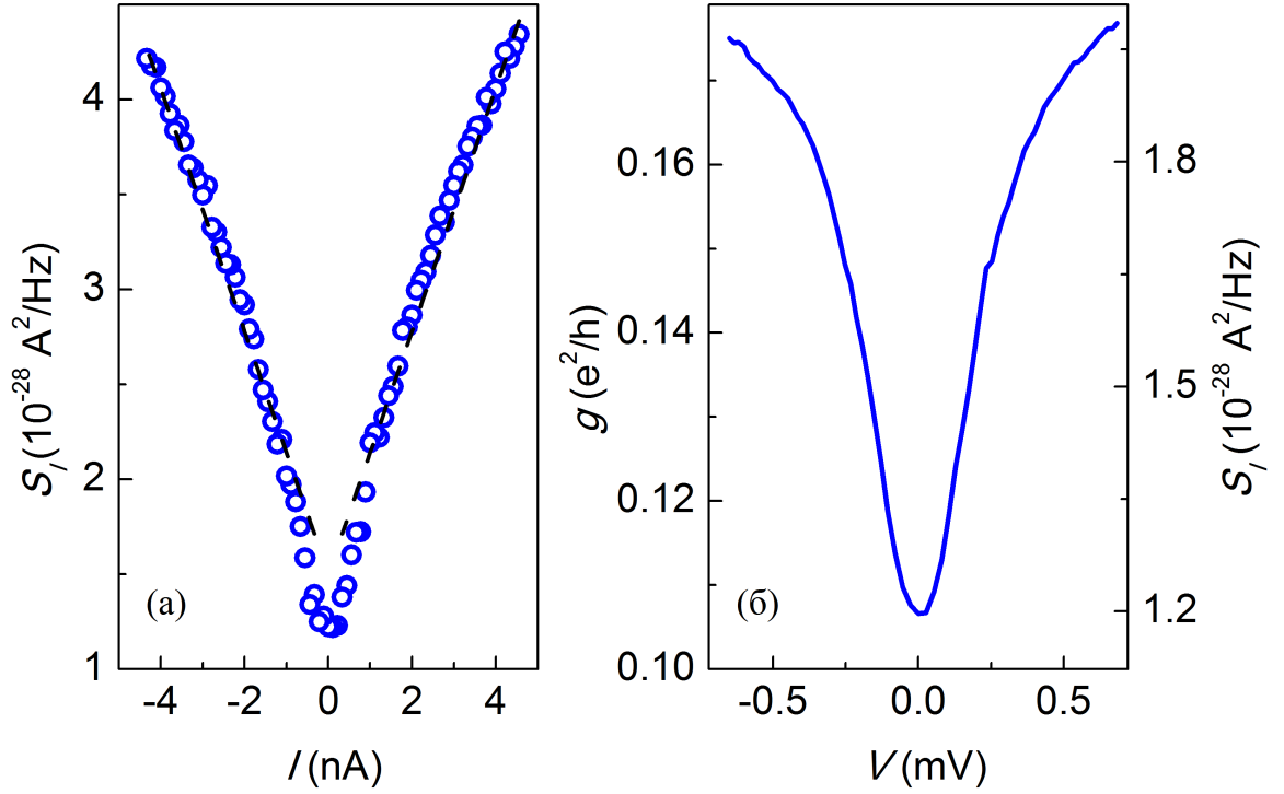
Рис. 5.9: Дробовой шум и дифференциальный кондактанс в режиме краевого транспорта в образце I. (а) Спектральная плотность дробового шума как функция тока при V_g = -3.2 В (символы). Наклон пунктирной линии соответствует величине фактора Фано F = 0.2 . (б) Дифференциальный кондактанс как функция тянущего напряжения (левая вертикальная ось) и соответствующий вклад теплового шума Джонсона-Найквиста S_I = 4k_B Tg (правая вертикальная ось). Учтен вклад конечного сопротивления контактов в проводимость.
