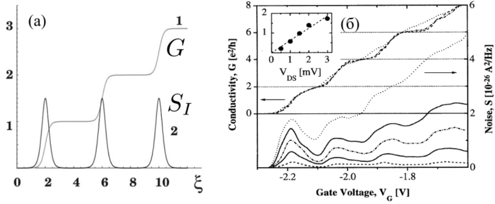
Рис. 3.2: (а) Кондактанс в единицах e^2/2\pi\hbar (кривая 1) и спектральная плотность токового шума на нулевой частоте в единицах e^3|V|/6\pi\hbar (кривая 2) точечного контакта как функция обезразмеренного затворного напряжения. Изображение из работы [2]. (б) Спектральная плотность шума и нормированный кондактанс квантового точечного контакта как функции затворного напряжения V_g при T = 1.5 К. Шум измерялся при тянущих напряжениях V_{sd} = 0.5, 1, 1.5, 2 и 3 мВ. На вставке: высота первого пика в шуме при различных V_{sd} . Экспериментальные данные из работы [48].
