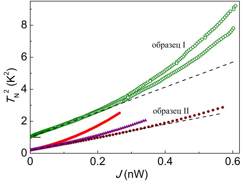
Рис. 3.15: Квадрат шумовой температуры как функция джоулевой мощности для двух образцов. Открытые символы соответствуют образцу I при R_0 \approx 2.1 кОм, заштрихованные - образцу II при R_0 \approx 0.5 кОм (кружки), 1.5 кОм (треугольники) и 3.4 кОм (квадраты). Для образца I верхняя (нижняя) ветвь соответствует V < 0 ( V > 0 ), в то время как в образце I кривые симметричны в обеих полярностях. Пунктирные линии построены по экстраполяции линейной зависимости T_N^2 - T_0^2 \propto J из малых значений J . Температура ванны T_0 = 0.1 К для образца I и T_0 = 0.5 К для образца II. Для удобства данные для образца I смещены по вертикали.
