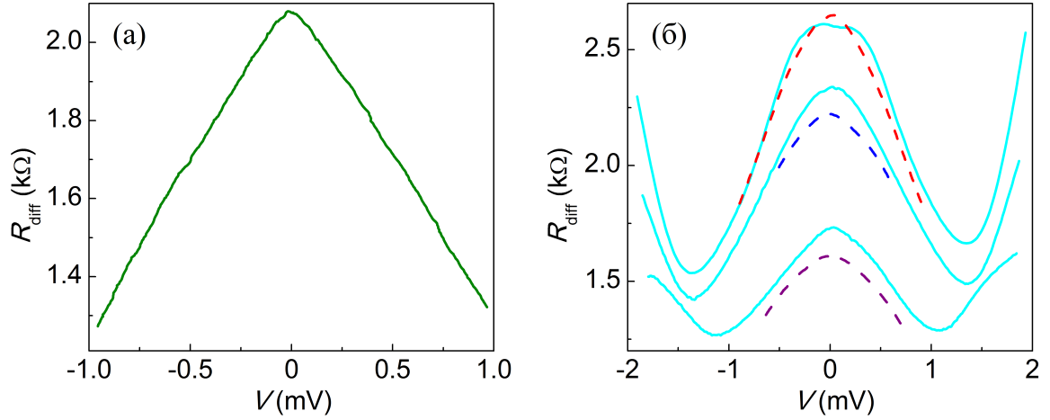
Рис. 3.12: (а) Дифференциальное сопротивление образца I как функция тянущего напряжения ( T = 0.1 K). (б) Дифференциальное сопротивление образца II (пунктирные линии, T = 0.5 K, R_0 = 1.5, 2 и 3.4 кОм) и образца III (сплошные линии, T = 0.1 K, R_0 = 1.2, 2.3 и 3.3 кОм) в зависимости от тянущего напряжения. Данные сдвинуты по вертикали для наглядности.
