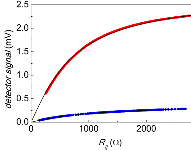
Рис. 2.10: Калибровка установки при помощи измерения теплового шума. Красные и синие символы соответствуют измерениям при температурах ванны 4.2 К и 0.43 К, сплошные линии – подгонки с параметрами R_0 = 3.3 кОм, L = 7 мкГн, C = 22 пФ.
