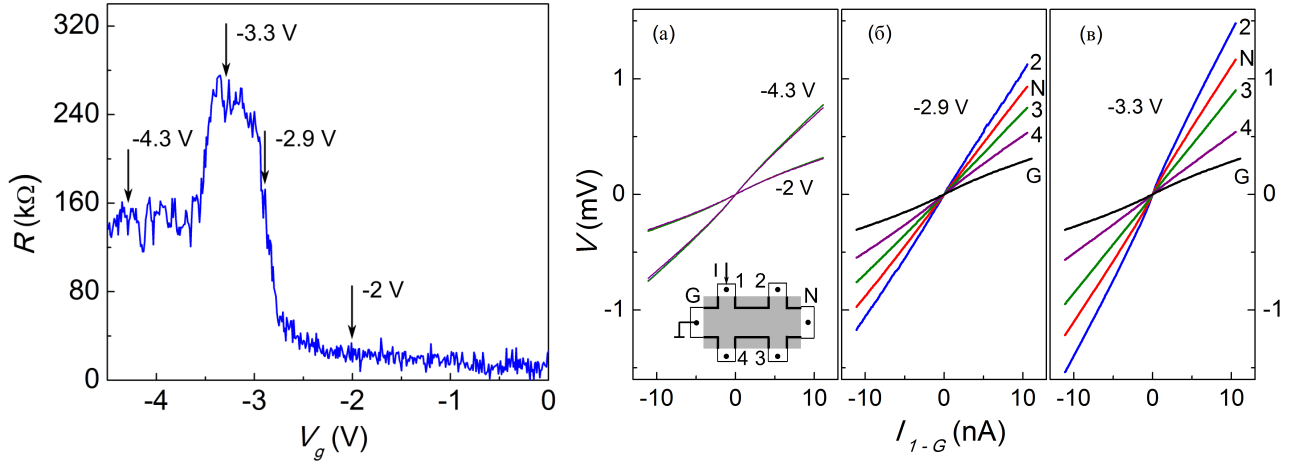
Рис. 5.7: Слева: двухтерминальное сопротивление в режиме линейного отклика. Справа: Краевой транспорт в режиме нелинейного отклика. (а) Объемный транспорт в области проводимости p -типа ( V_g = -4.3 В) и n -типа ( V_g = -2 В) вдали от точки нейтральности. В обоих случаях напряжение на контактах 2, N , 3 и 4 совпадает с экспериментальной точностью. Вставка: схема трехтерминального измерения нелокального сигнала в образце I с заданием тока через контакт 1 и заземленным контактом G . (б,в) Краевой транспорт в области точки нейтральности при V_g = -2.9 В и V_g = -3.3 В. Помимо сигналов с контактов 2, N , 3 и 4 здесь также построен вклад последовательного сопротивления контакта G и соответствующей части мезы. Вертикальная шкала общая для трех графиков.
