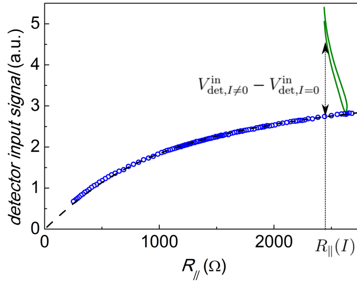
Рис. 2.12: Сигнал на детекторе как функция сопротивления R_{||} . Синие символы соответствуют измеренному тепловому шуму при температуре T = 0.44 К, зеленая кривая – неравновесному шуму. Две ветви на зеленой кривой соответствуют положительным и отрицательным токам. Пунктирная линия - ожидаемое значение сигнала теплового шума для значений R_0 = 3.3 кОм, L = 6 мкГн, C_{\text{par}} = 18 пФ.
