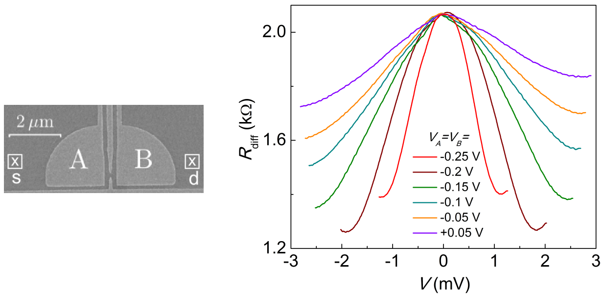
Рис. 3.13: Слева: Микрофотография образца IV. Справа: Дифференциальное сопротивление образца IV как функция тянущего напряжения ( T = 0.5 K, R_0 = 2.07 кОм). Электронная концентрация вблизи сужения контролировалась приложением напряжения V_{A,B} к затворам A и B , а напряжение на расщепленном затворе подбиралось таким образом, чтобы сопротивление точечного контакта в режиме линейного отклика оставалось равным R_0 .
