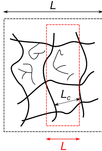
Рис. 4.1: Критический кластер (жирные линии) в сильно неоднородной системе, отражающий картину токонесущих состояний. Масштаб картины определяется температурой и плотностью состояний на уровне Ферми. Пунктирные черный и красный прямоугольники демонстрируют два возможных случая: L \gg L_c и L \sim L_c соответственно, где L – размер образца в направлении протекания тока. Контакты подключены к вертикальным сторонам пунктирных прямоугольников.
