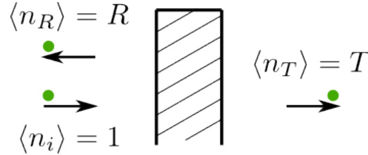
Рис. 5.3: Схематическое изображение барьера в когерентном одноканальном проводнике.
