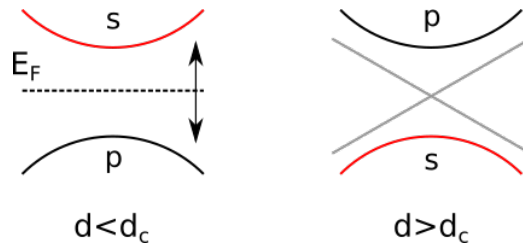
Рис. 5.1: Энергетический спектр квантовой ямы: краевые состояния в щели широкой квантовой ямы (справа).
