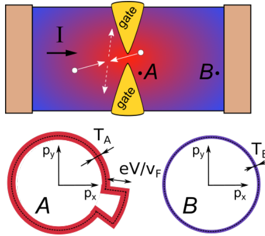
Рис. 3.10: Идея эксперимента. Ток I течет через точечный контакт, и электронная функция распределения становится неравновесной. Помимо простого разогрева двумерного электронного газа, отраженного градиентом цвета, мы изучаем влияние электрон-электронного рассеяния во встречных электронных пучках на сопротивление и на шум точечного контакта. В нижней половине рисунка показаны электронные функции распределения в импульсном пространстве для точек A и B . В точке A функция распределения анизотропна с выпуклостью eV/v_F и высокой локальной температурой T_A , в точке B функция распределения локально равновесная с более низкой температурой T_B .
