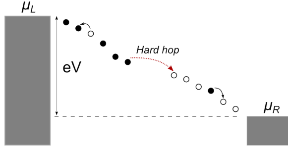
Рис. 4.8: Прыжки вдоль одномерной цепочки локализованных состояний с тяжелым прыжком посередине. Закрашенные/пустые кружки – занятые/свободные состояния.
