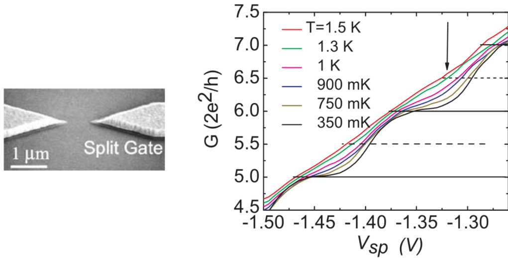
Рис. 3.3: Из работы [52]. Слева: СЭМ изображение одного из исследовавшихся точечных контактов. Справа: Кондактанс, измеренный в режиме линейного отклика, как функция затворного напряжения при различных температурах.
