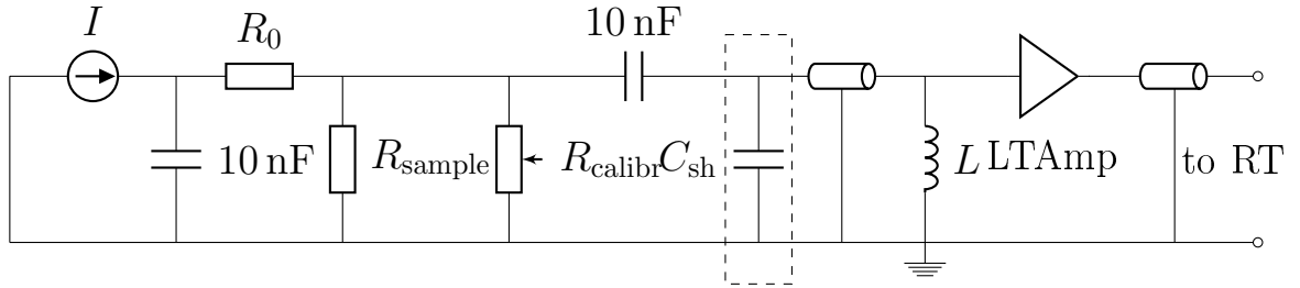
Рис. 2.3: Принципиальная схема измерений при низкой температуре.
