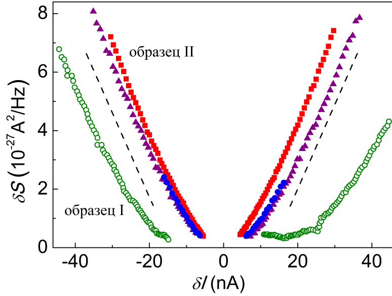
Рис. 3.16: Спектральная плотность \delta S «избыточного» шума как функция нелинейной добавки в ток. Открытые символы соответствуют образцу I при R_0 \approx 2.1 \text{ кОм} ( 0.5 \text{ мВ} \leq |V| \leq 1 \text{ мВ} ), заштрихованные - образцу II при R_0 \approx 1.5 \text{ кОм} (треугольники, 0.4 \text{ мВ} \leq |V| \leq 0.7 \text{ мВ} ), 2 \text{ кОм} (кружки, 0.4 \text{ мВ} \leq |V| \leq 0.6 \text{ мВ} ) и 3.4 \text{ кОм} (квадраты, 0.5 \text{ мВ} \leq |V| \leq 0.9 \text{ мВ} ). Пунктирные линии построены с наклоном F^* = 0.9 . Для образца I масштаб по обеим осям уменьшен в 2 раза.
