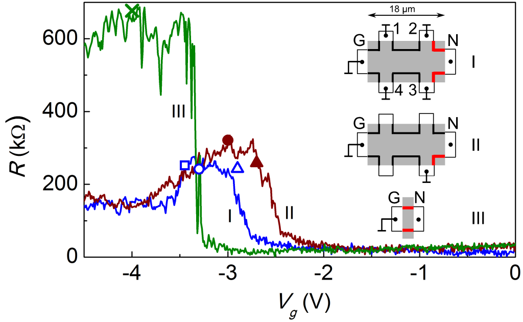
Рис. 5.6: Двухтерминальное сопротивление в режиме линейного отклика для трех образцов как функция затворного напряжения при температуре T = 0.52 K. Символами обозначены координаты (R_{2p}, V_g) , для которых в дальнейшем будет обсуждаться дробовой шум. Непоявление некоторых символов на соответствующую кривую связано с небольшим дрейфом во времени состояния образца.
