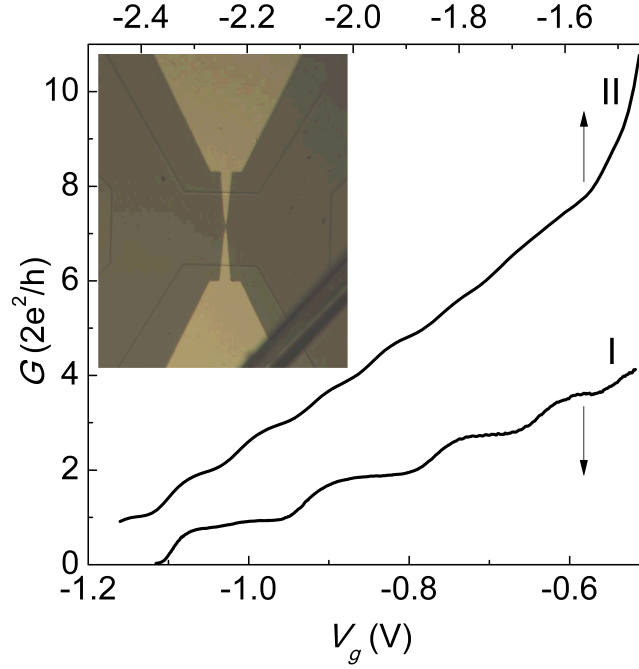
Рис. 3.11: Кондактанс точечных контактов I и II как функция затворного напряжения при температурах T = 0.1\text{ К} и T = 0.5\text{ К} соответственно. На вставке: микрофотография сужения II.
