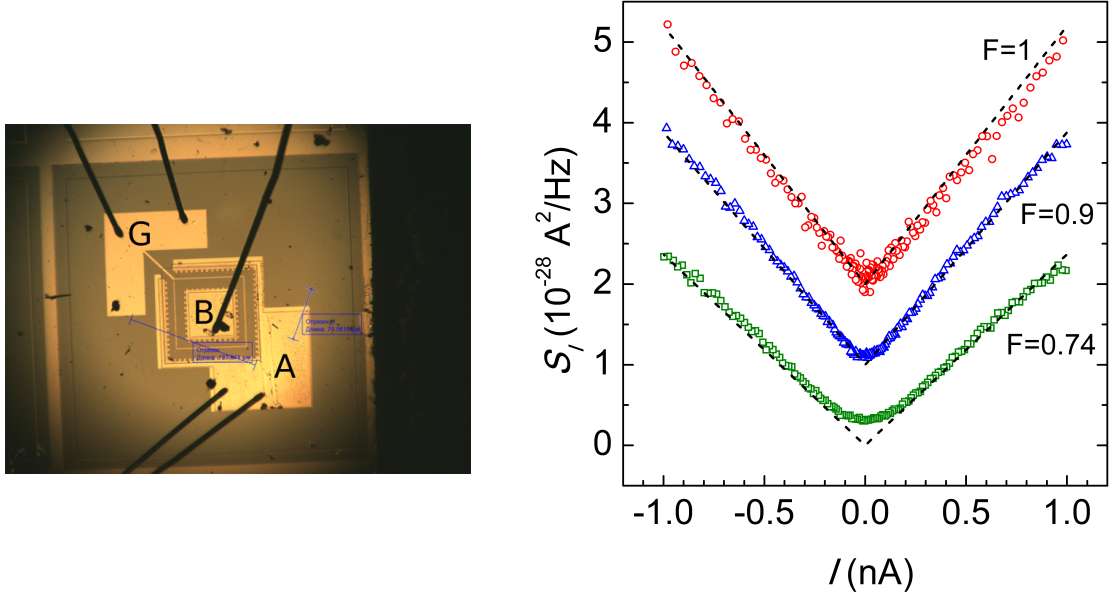
Рис. 4.9: Слева: Фотография исследованного образца (см. текст). Справа: Спектральная плотность дробового шума как функция тока при T = 0.5 \text{ К} . Удельное сопротивление образца сверху вниз: R_{\square} \approx 5 \text{ ГОм} , R_{\square} = 380 \text{ МОм} , R_{\square} = 75 \text{ МОм} . Пунктирные линии соответствуют наклону экспериментальных кривых в области линейной зависимости от тока. Масштаб по обеим осям уменьшен в 10(5) раз для нижнего(среднего) набора данных. Два верхних набора данных сдвинуты по вертикали на 1 и 2 \cdot 10^{-28} \text{ А}^2/\text{Гц} .
