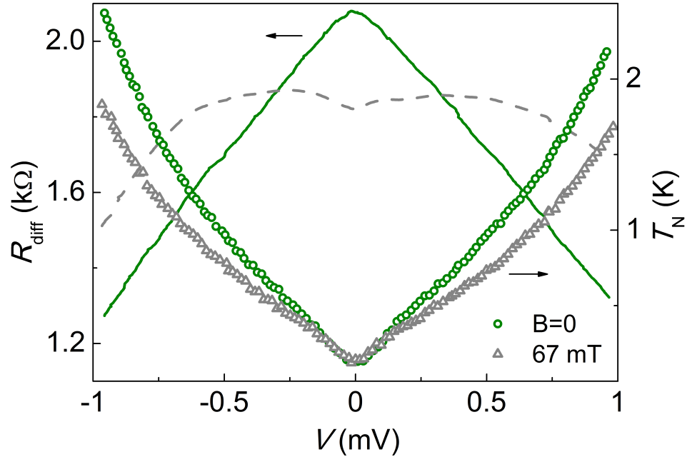
Рис. 3.17: Влияние магнитного поля на дифференциальное сопротивление и шум в образце I.
