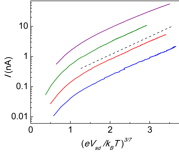
Рис. 4.4: Нелинейные вольт-амперные характеристики при T = 0.47 К. Кривые соответствуют сопротивлениям R_{\square} = 0.5, 1.6, 6, 19 МОм. Пунктирная линия проведена для L_c = 11 мкм.
