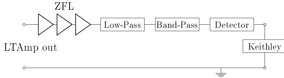
Рис. 2.5: Схема измерений при комнатной температуре.
