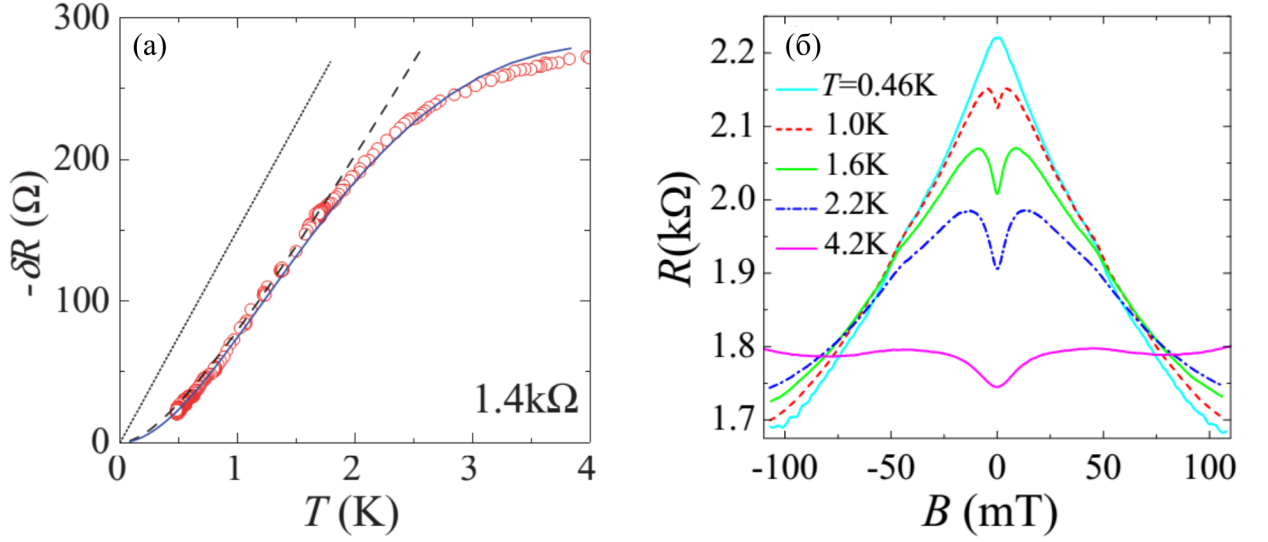
Рис. 3.7: (а) Экспериментальная температурная зависимость добавки в сопротивление точечного контакта, представленной в виде -\delta R \equiv -(R(T) - R_0) , где R(T) - измеренное при данной температуре сопротивление, а величина R_0 определяется из данных магнитосопротивления. В данном случае R_0 = 1.4 кОм. Точки в соответствии с [55], пунктир - численный расчет в духе [53] для демонстрации отклонений от линейной зависимости при низких температурах. (б) Эволюция магнитосопротивления точечного контакта для R_0 = 2.2 кОм с температурой. Экспериментальные данные из работы [58].
