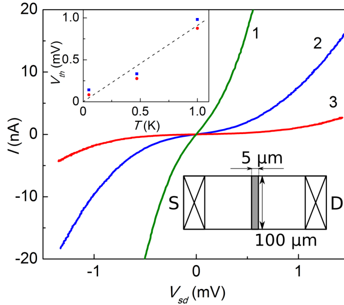
Рис. 4.2: Вольт-амперные характеристики образца при T = 0.56 \text{ К} для различных затворных напряжений: (1) V_g = -0.302 \text{ В} , (2) V_g = -0.308 \text{ В} , (3) V_g = -0.339 \text{ В} .
