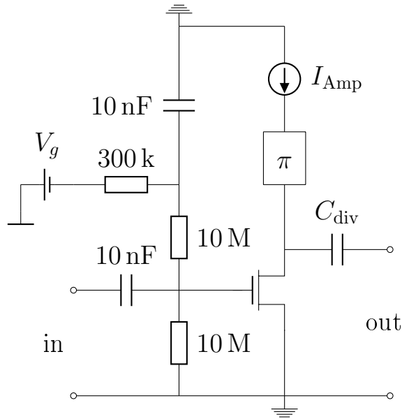
Рис. 2.4: Схема низкотемпературного усилителя LTamp.
