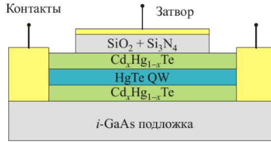
Рис. 2.2: Схематическая структура изучаемых квантовых ям. Рисунок из работы [42].
