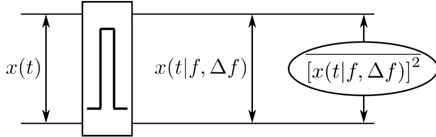
Рис. 1.2: Принципиальная схема измерения спектральной плотности сигнала x(t) . Здесь x(t) – флуктуации сигнала, x(t|f, \Delta f) – флуктуации сигнала, прошедшие через фильтр, [x(t|f, \Delta f)]^2 – мощность флуктуаций, прошедших через фильтр.
