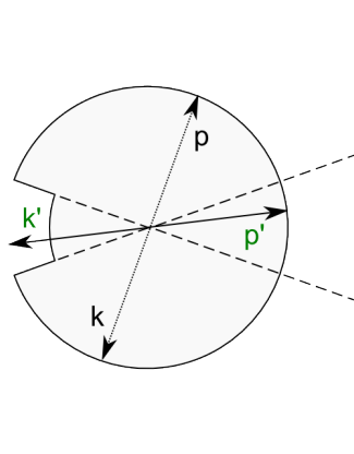
Рис. 3.5: Акты e - e рассеяния, дающие вклад в кондактанс точечного контакта.
