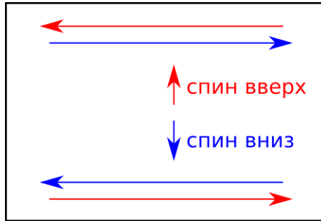
Рис. 5.2: Токонесущие краевые состояния в режиме квантового спинового эффекта Холла.
