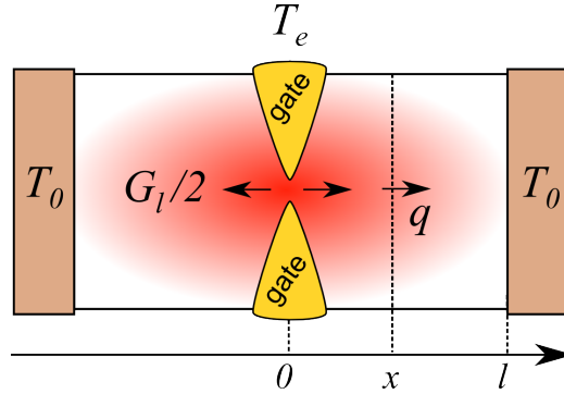
Рис. 3.8: Учет нагрева электронной системы при eV \gg k_B T .
