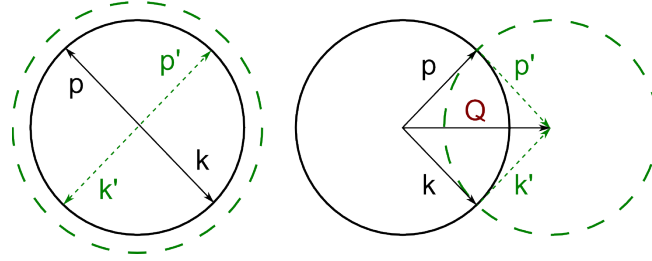
Рис. 3.6: Электрон-электронное рассеяние в импульсном пространстве для случая нулевой температуры T = 0 . (а) Электроны с \mathbf{Q} = \mathbf{p} + \mathbf{k} = 0 могут рассеяться в любую пару электронов \mathbf{p}' и \mathbf{k}' такую, что \mathbf{p}' + \mathbf{k}' = 0 . (б) Пара электронов с \mathbf{Q} \neq 0 при рассеянии могут либо обменяться, либо сохранить свои импульсы.
