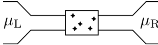
Рис. 1.4: Сечение двухконтактного проводника, соединенного с двумя резервуарами.
