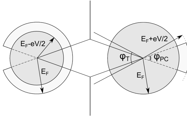
Рис. 3.4: Поверхность Ферми слева и справа от точечного контакта при отсутствии e - e рассеяния
