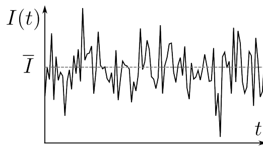
Рис. 1.1: Флуктуации тока через мезоскопический проводник.
