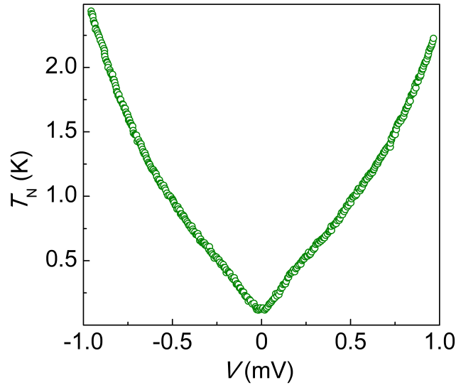
Рис. 3.14: Шумовая температура T_N точечного контакта I как функция тянущего напряжения.
