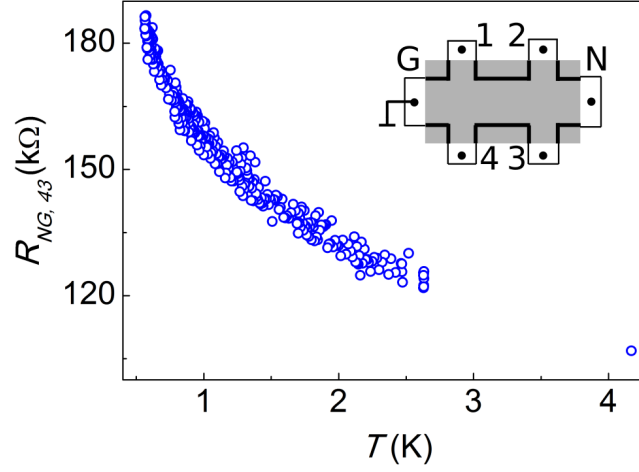
Рис. 5.11: Температурная зависимость четырехточечного сопротивления R_{NG,43} , измеренного в режиме линейного отклика, в образце I в области точки нейтральности при V_g = -3.2 В.
