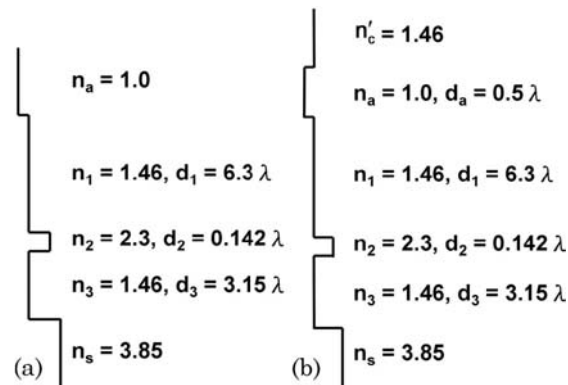
Рис. 2. (а) Структура ARROW. (б) Структура ARROW с добавленным слоем с высоким показателем
