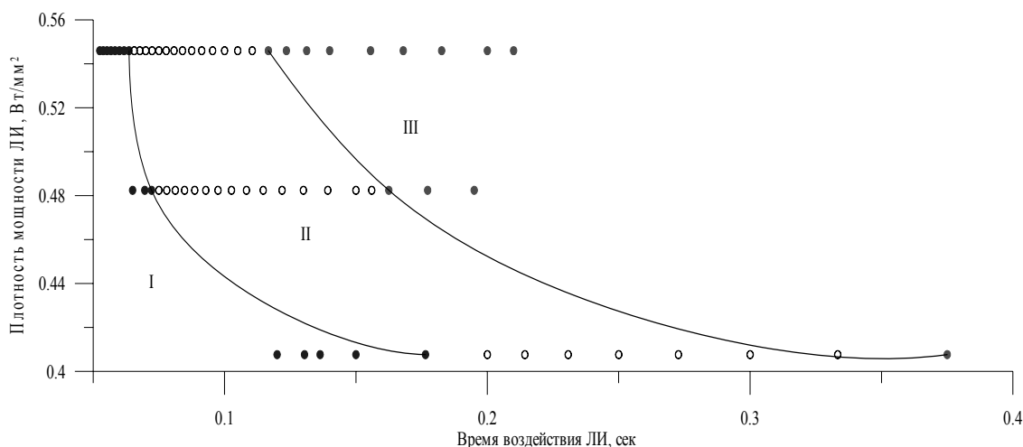
Рис. 1. Область технологических режимов спекания КПК на \text{CO}_2 -лазере: I – область, где образцы не спекаются; II – область спекания; III – область деструкции полимера
