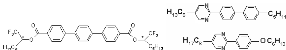
Рис.2. Химическая формула хиральной структуры (S,S)-bis-(1,1,1-трифтороокт-2-ил)-4,4'-терфенилдикарбоксилата (FOTDA) (слева) и бинарной матрицы (справа)
