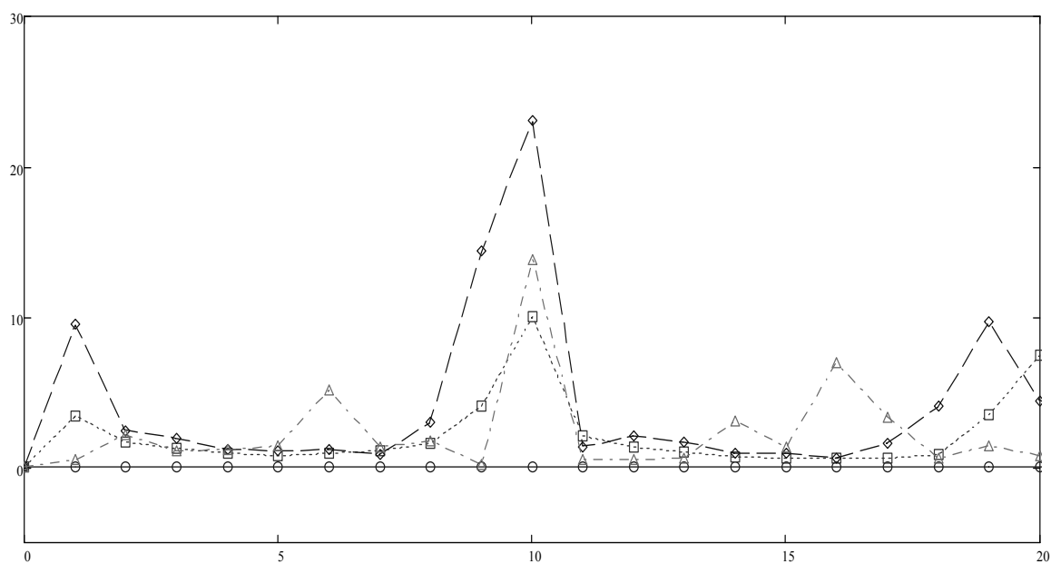
Рис. 4. Спектр распределения интенсивности вдоль оси x_0 ( \circ – H=0 , \square – H=0.02 , \Delta – H=0.05 , \diamond – H=0.15 )
