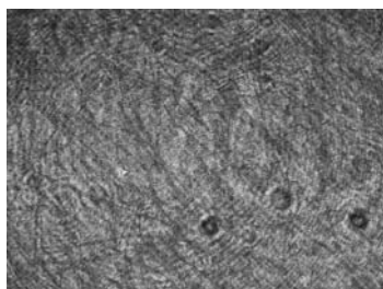
Рис.4. Цифровая голограмма
