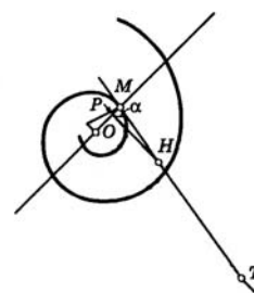
Рис. 2. Логарифмическая спираль
