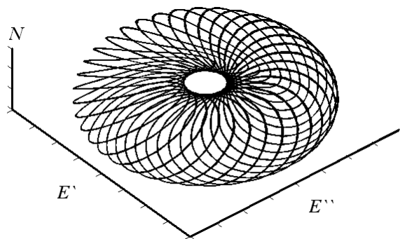
Рис.3. Аттрактор в виде устойчивого двумерного тора при v = 9.5
