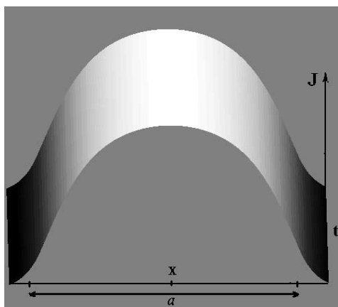
Рис.1. Пространственно-временная динамика при v = 5
