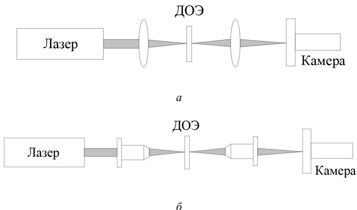
Рис. 2. Общий вид оптических схем с использованием линз(а) и с использованием микрообъективов(б)
