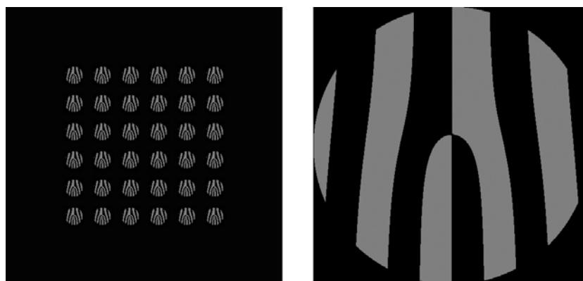
Рис. 1. Слева группа ДОЭ формирующих оптический «вихрь» третьего порядка с разрешением 32х32 точек, справа ДОЭ формирующий оптический «вихрь» первого порядка с разрешением 512х512 точек
