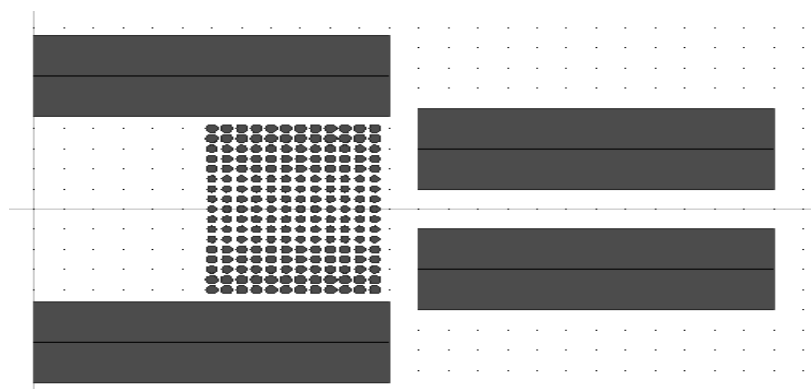
Рис. 1. Изображение \Phi K -линзы вместе с волноводами
