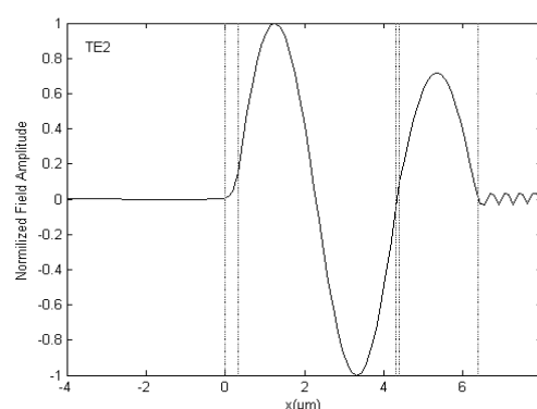
Рис. 4. Профиль моды TE_2 из табл. 1 структуры ARROW, представленной на рис. 2 (b)
