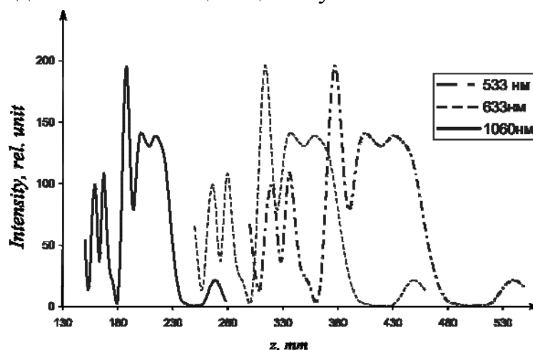
Рис. 1. Распределение интенсивности вдоль оптической оси
