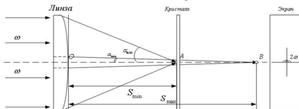
Рис.2. Схема хода лучей из разных кольцевых зон линзы (пояснение в тексте)
