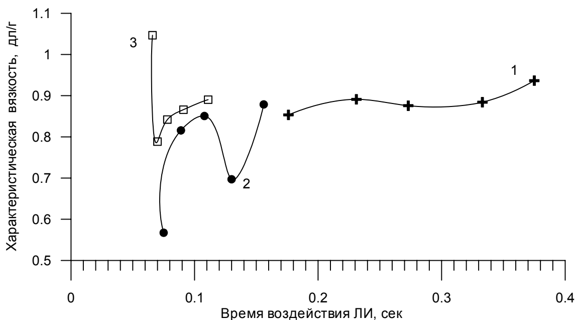
Рис. 5. Изменение характеристической вязкости образцов в зависимости от времени воздействия ЛИ при мощности 8 Вт (1), 16 Вт (2), 21 Вт (3)
