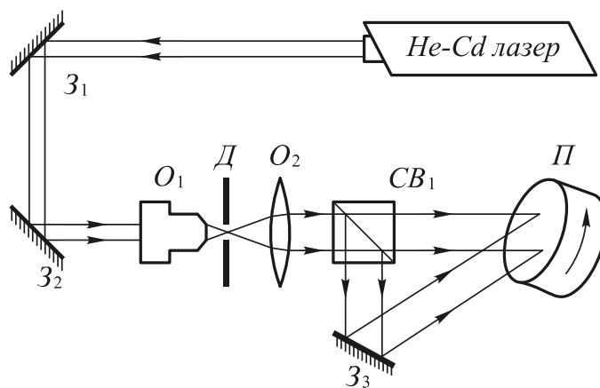
Рис.1. Буквами обозначены: Z_1, Z_2, Z_3 , – зеркала, O_1, O_2 – объективы, D – диафрагма, CB_1 – делительный кубит, \Pi – подложка из стекла с нанесенным на нее фоторезистом.
