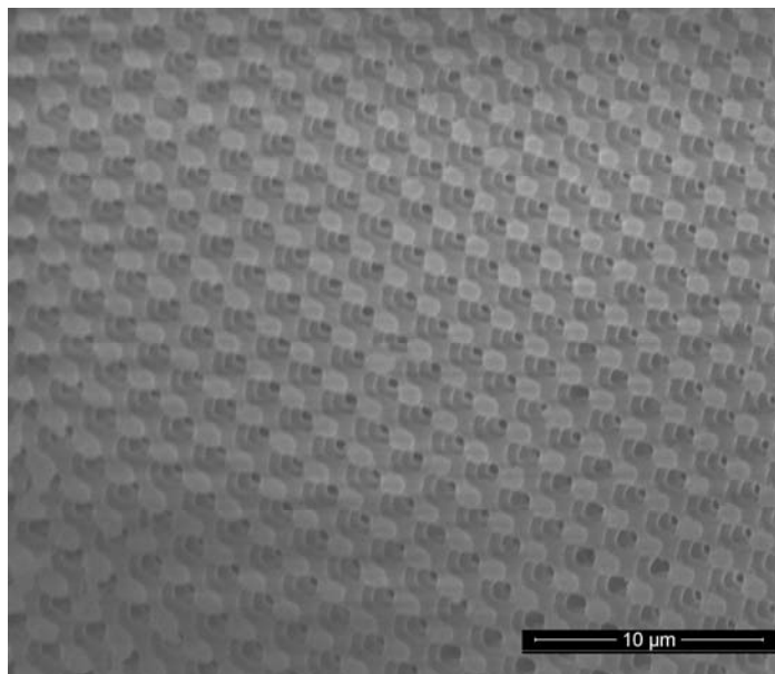
Рис. 2. Электронная фотография трехмерного фотонного кристалла
