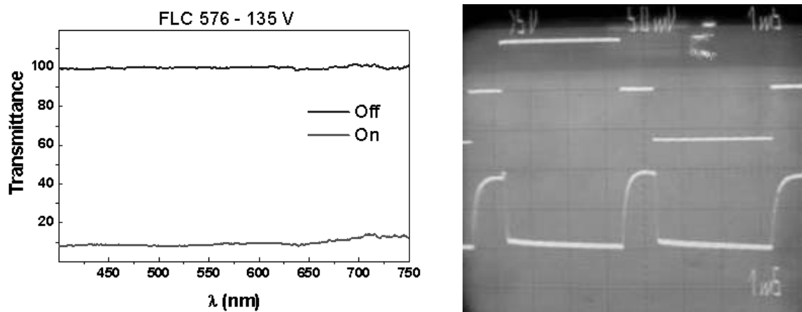
Рис. 8. Слева – спектры пропускания модулятора светорассеяния на основе смектической наноструктуры СЖК-576, толщина слоя СЖК – 21 \mu\text{м} , шаг спирали p_0=165 нм. Справа – фотография экрана осциллографа светорассеивающей моды
