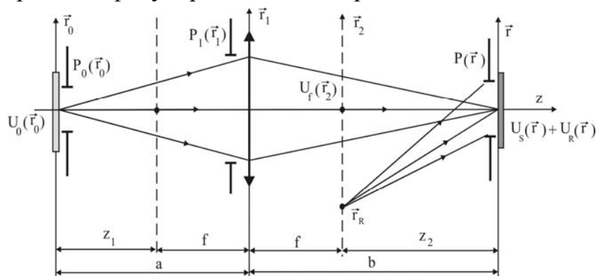
Рис. 1. К расчету комплексных амплитуд полей при записи безлинзовой фурье-голограммы сфокусированных изображений
