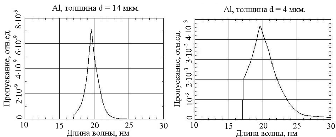
Рис. 2. Коэффициент пропускания алюминиевого фильтра, плотностью \rho = 2,6989 \text{ г/см}^3 для различных толщин
