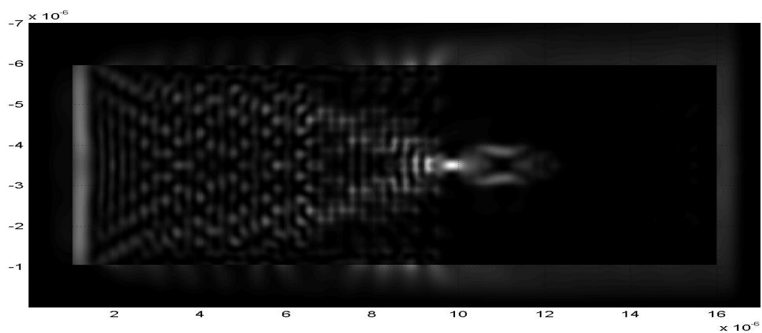
Рис. 6. 2D-распределение интенсивности |E_x|^2
