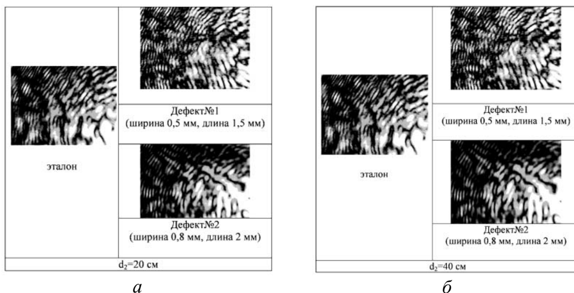
Рис.4. Результирующие спекл-картины, полученные при контроле поверхности фонаря кабины самолета с использованием спирального волнового фронта: а) d_2=20 см, б) d_2=40 см
