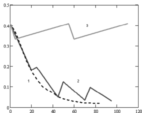
Рис. 6 График зависимости оптической плотности от времени для транс-цис перехода в зависимости от времени 1 — ПНТИ 10^{-4} ; 2 — t_{кр}=20 мин и t_{син}=5 мин; 3 — t_{кр}=5 мин и t_{син}=50 мин.
