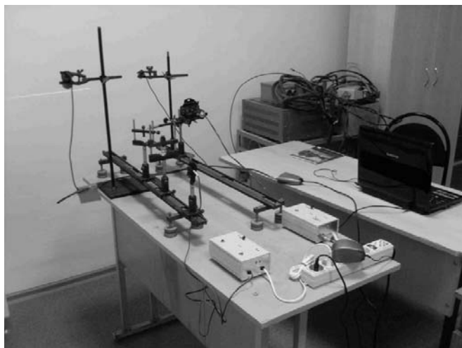
Рис. 3. Тест-установка
