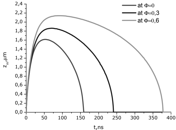
Рис. 3. Зависимость глубины проплавления от пористости
