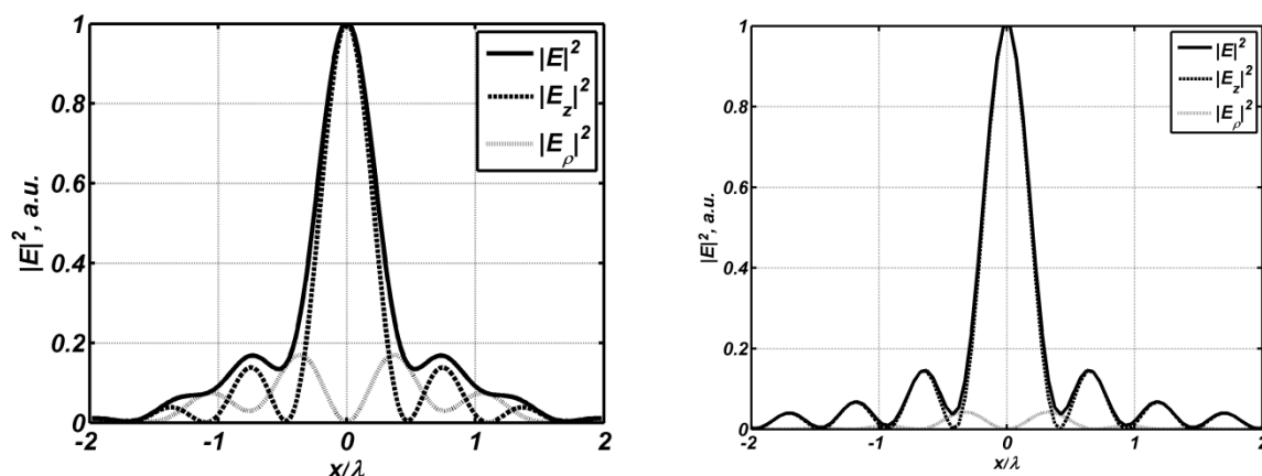
Рис. 5. Распределение интенсивности в фокусе при моделировании (а) методом FDTD, (б) с помощью формул Ричардса-Вольфа прохождения моды R-TEM 01 через зонную пластинку с фокусным расстоянием f=5\lambda
