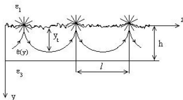
Рис.1. Схема распространения волны в плоском градиентном волноводу
