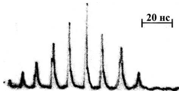
Рис. 5. Характерная осциллограмма генерации задающего лазера в режиме КРМП
