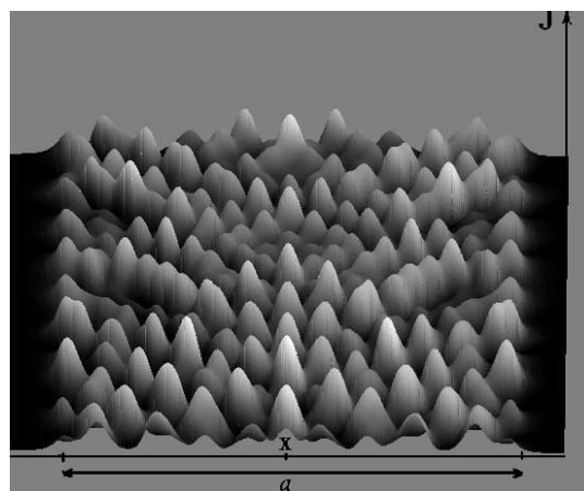
Рис.4. Пространственно-временная динамика при v = 15
