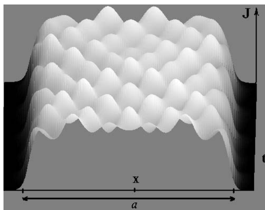
Рис.2. Пространственно-временная динамика при v = 9.5
