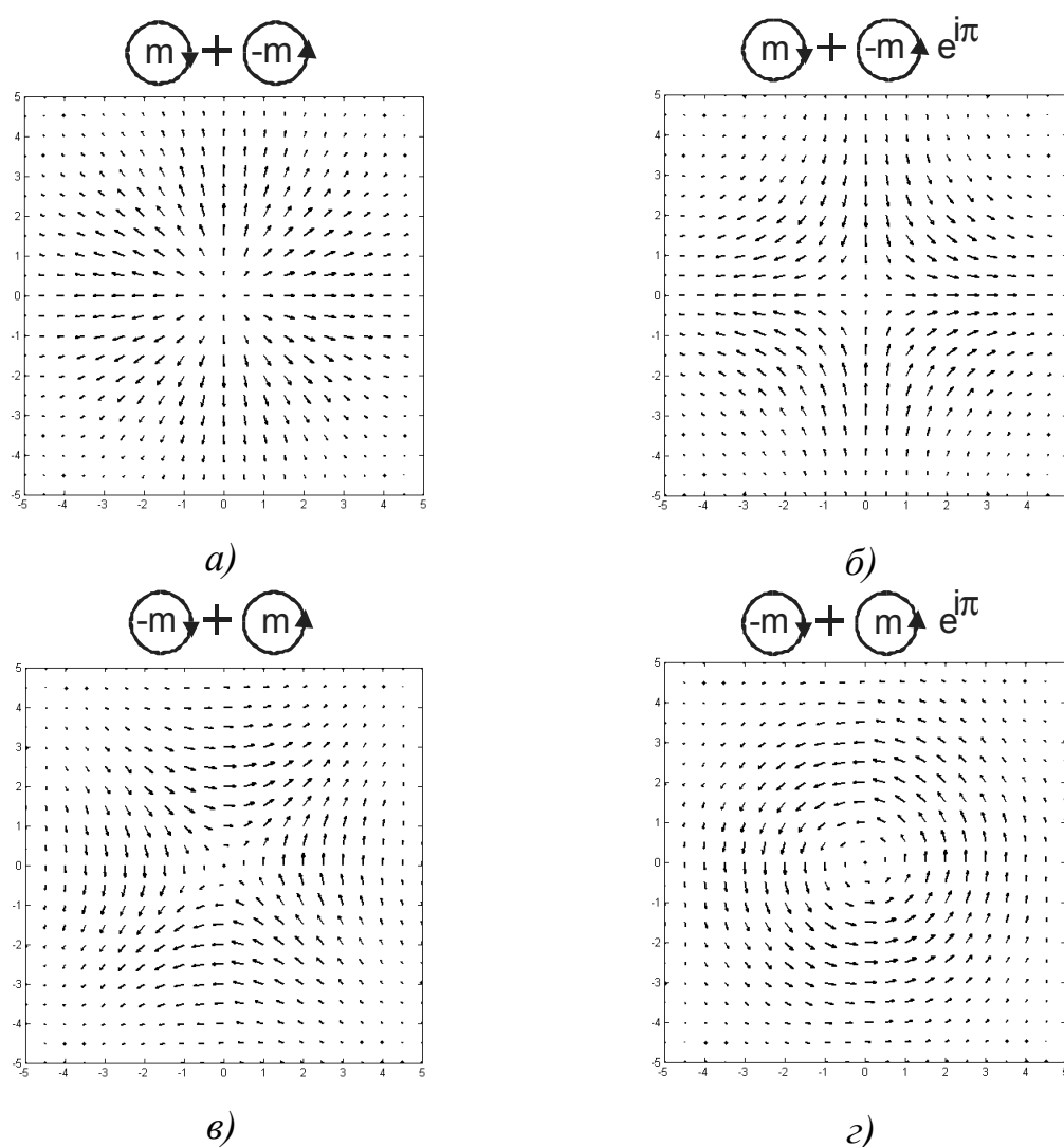
Рис. 1. Структура поляризации при сложении пучков Лагерра-Гаусса с топологическими зарядами |m|=1 (направление стрелок у кружков соответствуют правой и левой круговой поляризации)
