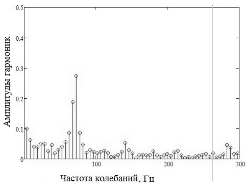
Рис. 4. Спектр частот
