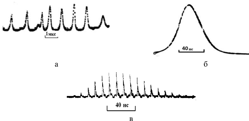
Рис. 1. Характерные осциллограммы, иллюстрирующие форму и временную структуру импульсов \text{YAP:Nd}^{3+} -лазера: а) – режим свободной генерации, б) – режим гигантского импульса, в) – режим кратковременной резонансной модуляции потерь
