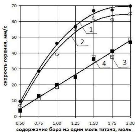
Рис.2 Зависимость скорости горения в среде азота от состава смесей, для различных условий проведения эксперимента.
