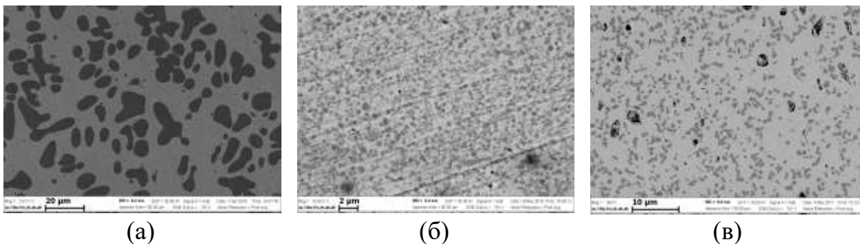
Рис. 2 – Микроструктура полученных образцов сплава 70Cu/30Fe: (а)- СВС-металлургия, (б) – торец ленты с установки Melt-spinnig CS, (в) – ВИП при 1200°C.
