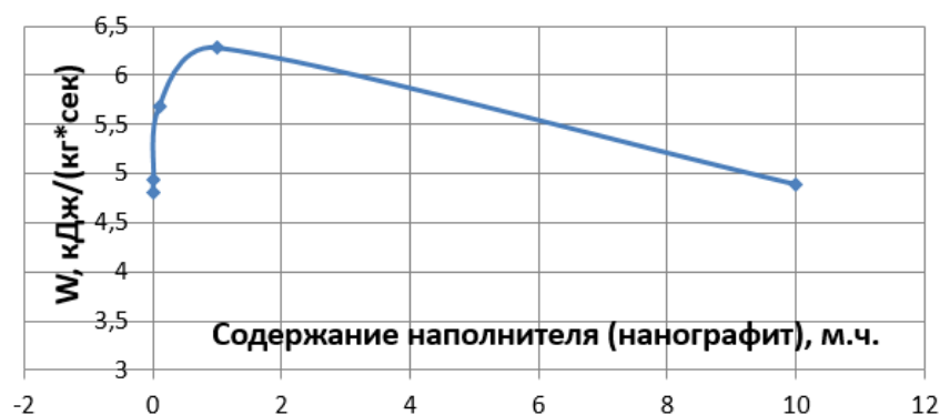
Рис. 1. Концентрационные зависимости удельной скорости поглощения энергии образцов СВМПЭ + графит от содержания наполнителя
