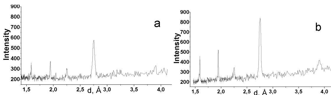
Рис.1. Рентгенограммы образцов манганита лантана \text{La}_{0,7}\text{Mn}_{1,3}\text{O}_{3\pm\Delta} , не подвергнутого прессованию (а) и спрессованного при P=0,8 ГПа (б). Температура синтеза -850^\circ\text{C} .
