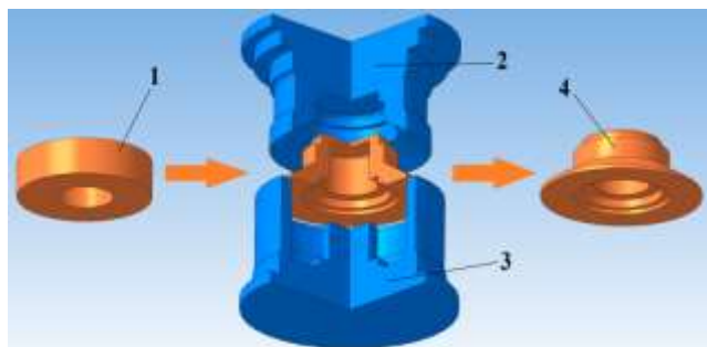
Рис 2. Схема объемной штамповки опорного изолятора из СВМПЭ-нанокомпозита: 1 – заготовка; 2 - пуансон; 3- матрица; 4 – готовое изделие.
