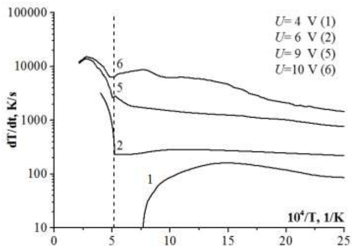
Рис. 2. Зависимости скорости нагрева образца от обратной температуры, полученные в ходе ЭТВ смеси титана и графита при давлении сжатия 48 МПа и электрических напряжениях: 1) 4; 2) 6; 5) 9; 6) 10 В.
