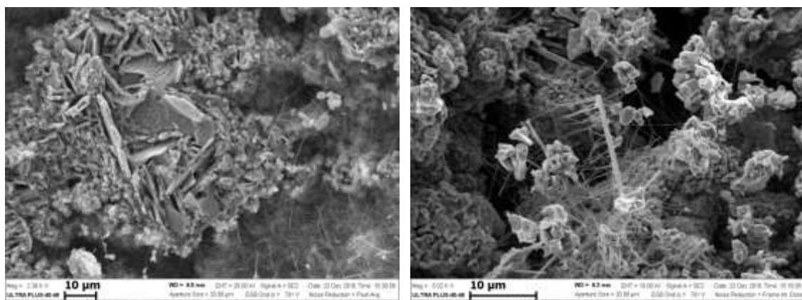
Рис.2. Микрофотографии распавшейся МАХ-фазы на TiN и AlN .
