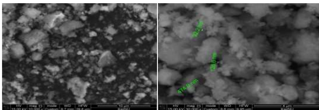
Рис.3. Микроструктура продуктов СВС (SEM) системы \text{Cr}_2\text{O}_3 - \text{V}_2\text{O}_5(\text{руда}) - \text{Mg} (МА 5 мин).
