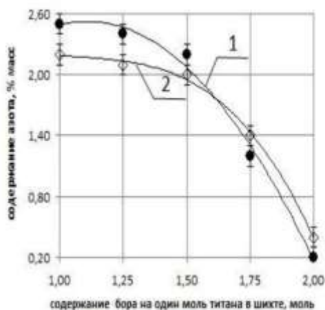
Рис.3 Зависимость содержания азота в продуктах реакции, для различных условий проведения эксперимента.
