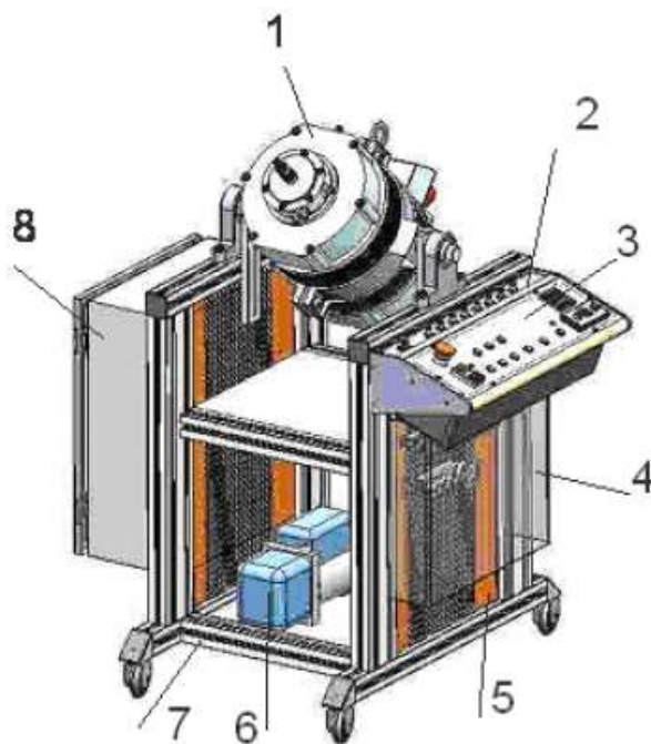
Рис.2. Внешний вид лабораторной установки ВЭГ.
