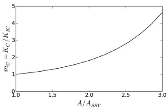
Рис. 1. Зависимость вязкости разрушения K_C от параметра стеснения деформации A .
