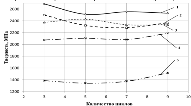
Рис. 2 Изменение твердости покрытия никеля в зависимости от времени и температуры напыления: 1 – 180°C; 2 – 360°C; 3 – 540°C; 4 – 540°C с последующей термической обработкой в печи при температуре 530°C и выдержке 2 часа; 5 – 540°C с последующей термической обработкой в печи при температуре 830°C и выдержке 4 часа.
