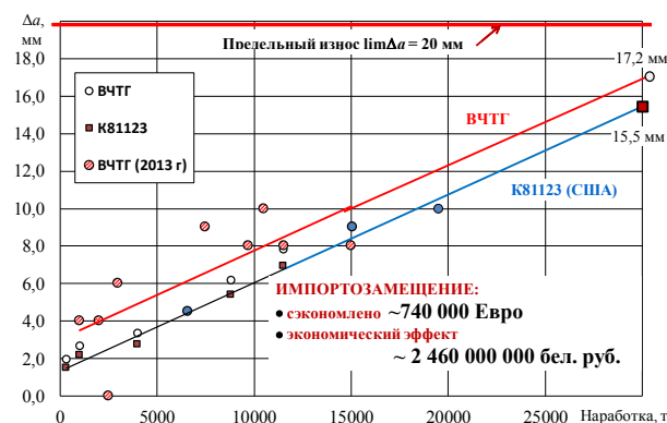
Рис. 3. Эксплуатационная стойкость чугунных и стальных ножей
