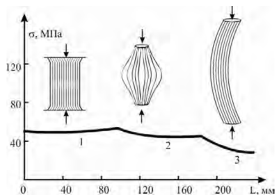
Рис. 1. Зависимости критических сжимающих напряжений \sigma от длины L композитных труб для трех видов разрушения
