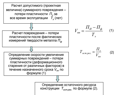
Рис. 1. Схема расчета остаточного ресурса металлоконструкции
