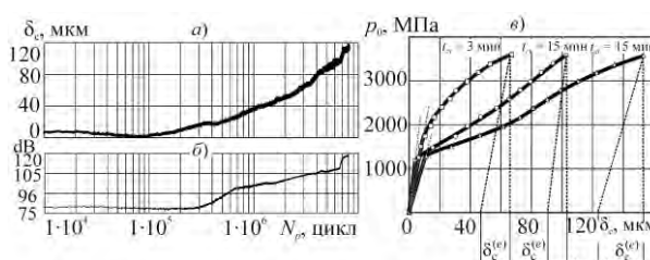
Рис.2 Регистрируемое в процессе испытаний на контактную усталость (регулярное динамическое нагружение) изменение сближения осей (а) и уровня шума (б); диаграмма контактного взаимодействия ( p_0 - \delta_c ) при ступенчатом динамическом нагружении контактной пары (в)
