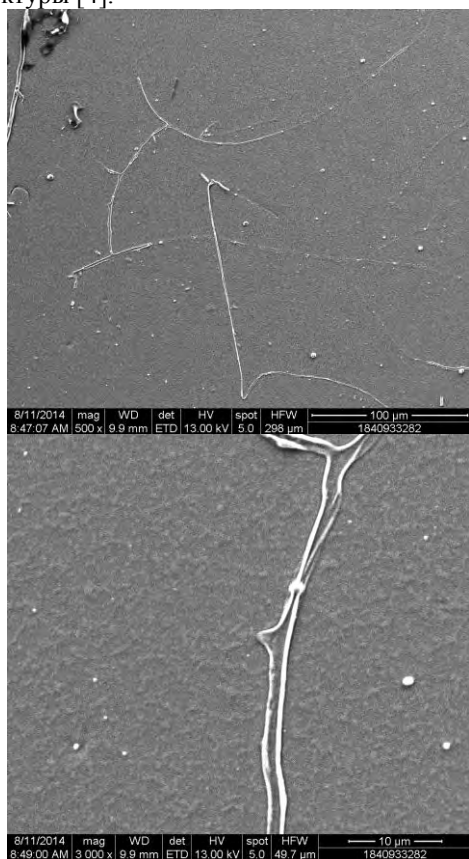
Рис.1. Фрактальные нити Ti
