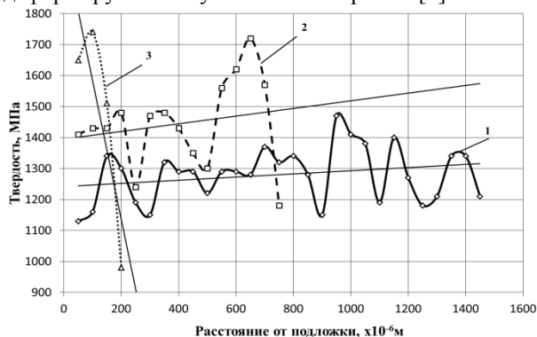
Рис. 1 Распределение твердости по глубине слоя меди, нанесённого при пяти циклах воздействия с температурой: 1-540°C, 2-360°C, 3-180°C.
