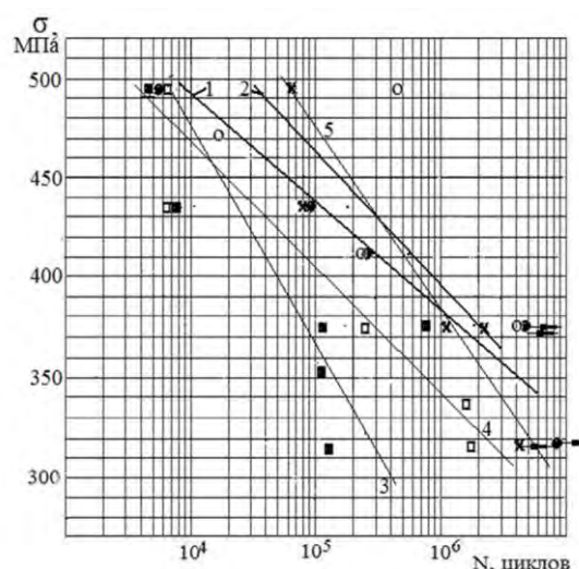
Рис.2 Кривые усталости образцов
