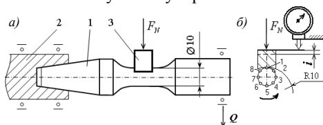
1 – образец; 2 – шпиндель; 3 – контроль-образец Рис. 1. Схема испытания на ФУ (при Q = 0 ) и ФМУ (при Q > 0 )
