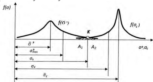
Рис. 1. Кривые плотности распределения нагрузки f(\sigma^p) и несущей способности f(\sigma_c)
