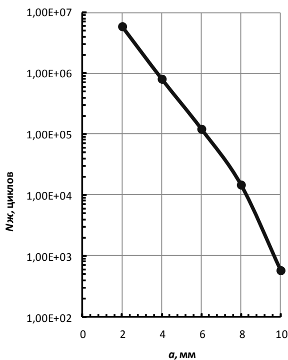
Рис. 1. График зависимости живучести N_{ж} элементов труб из основного металла от длины a полуоси поверхностной полуэллиптической трещины в осевом направлении
