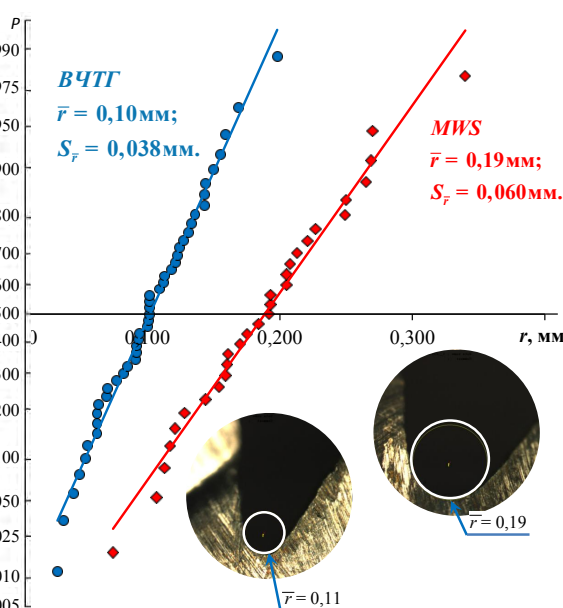
Рис. 2. Эмпирические функции распределения радиуса режущей кромки ножей MWS (сталь) и Гомсельмаш (чугун ВЧТГ) при наработке 1000 т.
