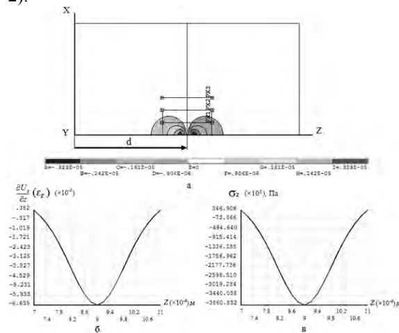
Рис. 2. Траектории PATH X_i в плоскости XZ образца из стекла на фоне изолиний компоненты U_x (м) вектора перемещений (а). Графики изменения \partial U_x / \partial z ( \varepsilon_z ) (б) и \sigma_z (в) для траектории PATH X_2 ( X=2 \times 10^{-4} м).
