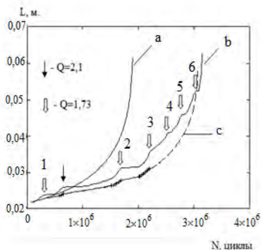
Рис. 1 Зависимость длины трещины L от числа циклов нагружения N ; а- расчётная, по КДУР без учёта влияния перегрузок; б - экспериментальная; с- расчётная, с учётом стадий развития;
