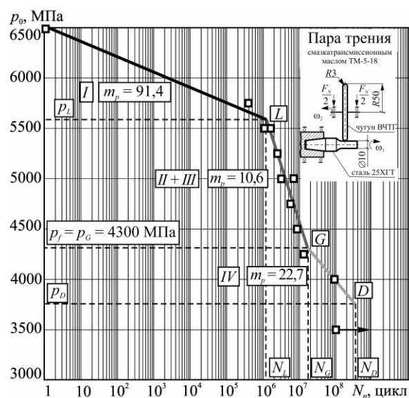
Рис. 3. Полная кривая контактной усталости
