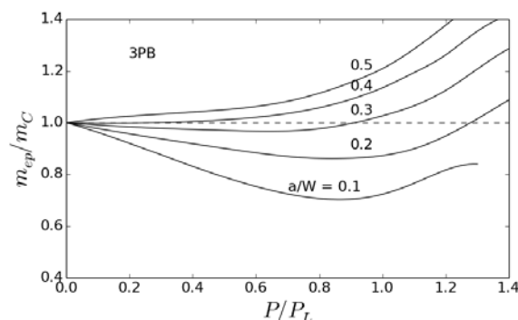
Рис. 2. Консервативность упругого подхода m_{ep}/m_e как функция нагрузки для образца на трехточечный изгиб.
