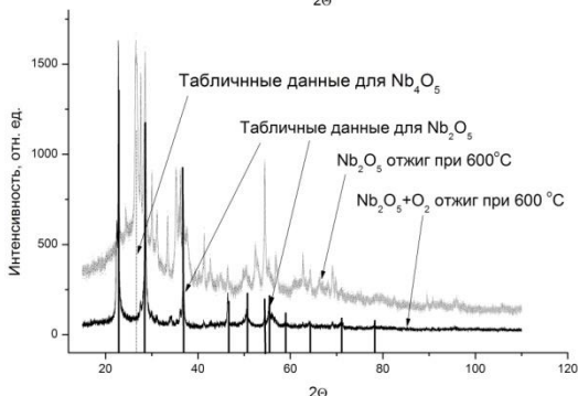
Рис. 2. – Дифрактограммы отожженных пленок \text{Nb}_2\text{O}_5
