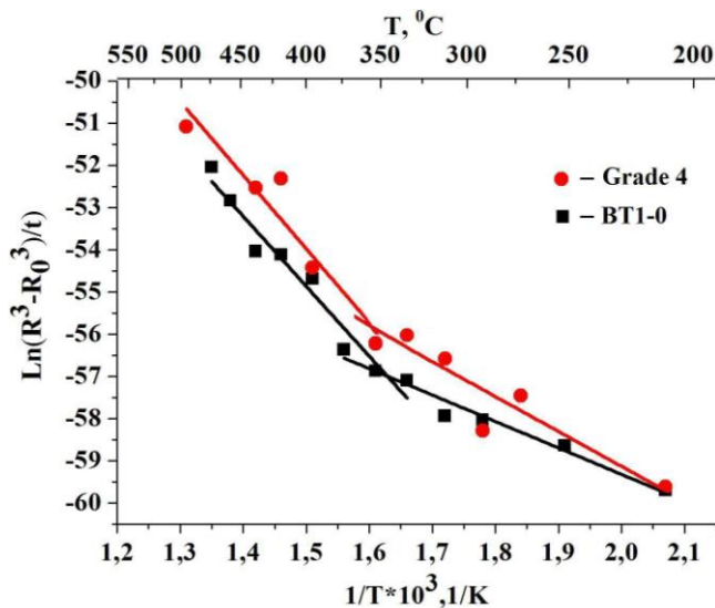
Рис. 1. Температурная зависимость скорости роста зерен в НС титане Grade4 и BT1-0 при n=3 .
