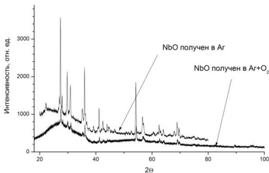
Рис. 1. Дифрактограммы исходных пленок \text{Nb}_2\text{O}_5 . Все пики на дифрактограммах принадлежат ситалловой подложке.
