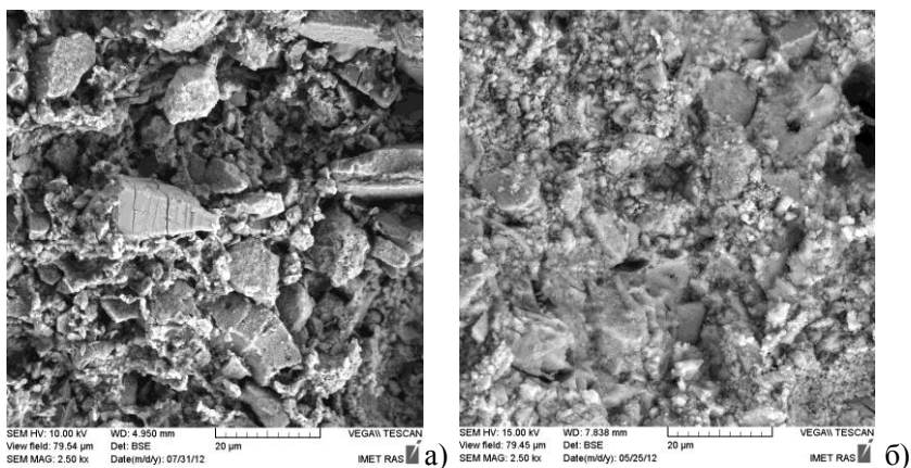
Рис. 1. СЭМ изображения композиционных цемента на 14 сутки: а - твердение на воздухе, б - . твердение в SBF.
