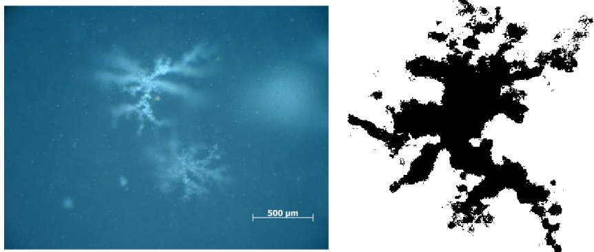
Рис. 1. Микроструктура композита на основе ПММА с 0,1 % ZrO_2 , черно-белое изображение трехмерной кластерообразной фрактальной структуры в виде дендритов для расчета фрактальной размерности
