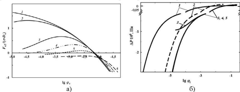
Рисунок - Составляющая капиллярной силы F_{k2} (а) и капиллярное давление \Delta P (б) в жидкой прослойке, (а) - h/D_{\text{ч}} : 1 - 4 \cdot 10^{-4} ; 2 - 1 \cdot 10^{-3} ; 3 - 0,01; 4 - 0,025; 5 - 0,05; 6 - 0,1; D_{\text{ч}} = 5 мкм, \theta = 50^\circ ; (б) - D_{\text{ч}} , мкм: 1 - 100; 2-5 - 10; h , мкм: 1, 2, 4 - 0,01; 3 - 0,1; 5 - 0,2 нм; \theta , ( ^\circ ): 1, 3-5 - 0; 2 - 50.
