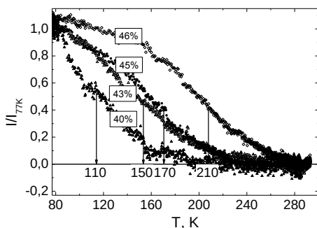
Рис. Зависимости намагниченности от температуры композитов \text{Ni}_x(\text{MgO})_{100-x} . Цифры под осью абсцисс соответствуют температуре Кюри каждого образца
