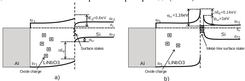
Рис. 1. Зонные диаграммы гетероструктур Si-LiNbO 3 сформированных методом высокочастотного магнетронного распыления в атмосфере Ar (a) и Ar+O 2 (b).
