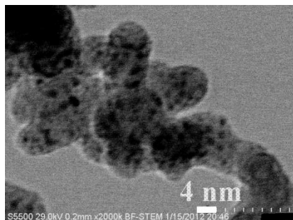
Наночастицы фторида алюминия в нанопибрилле. ПЭМ данные (светлое поле).
