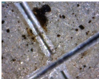
фото 1. Покрытие с наночастицами оксида железа без ПАВ с разрезом от решетки определения адгезии.
