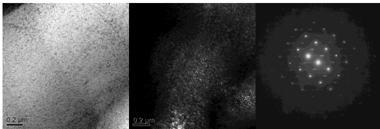
Рис.2. Микроструктура и микродифракция сплава Mg-4,35%Sm-11,5%Tb после старения 200°C, 8 ч.
