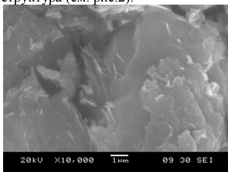
Рис 1. Поверхность разрушения вдоль слоев, ×10000
