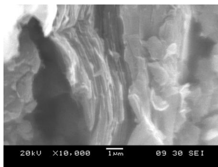
Рис 2. Поверхность разрушения поперек слоев, ×10000
