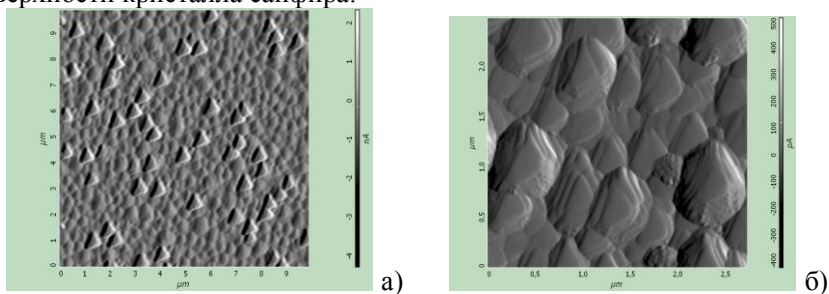
Рис.1. АСМ-изображения поверхности пленок (0001)ZnO/(0001) Al 2 O 3 на различных этапах роста.
