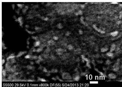
Наночастицы оксифторида титана на нанопибрилле. ПЭМ данные (темное поле).
