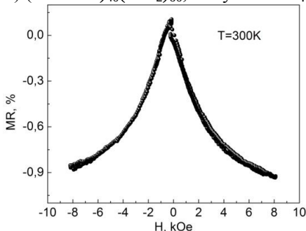
в) (\text{CoNbTa})_{60}(\text{SiO}_2)_{40} , получен при периодическом добавлении \text{O}_2 в Ar.
