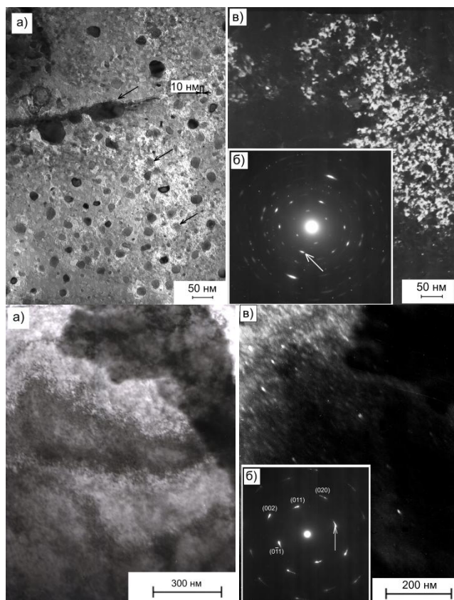
Рис. 5. а – светлопольное изображение структуры в зоне нерастворенного \text{Cr}_2\text{O}_3 ; б – электронограмма шпинели \text{FeO} \cdot \text{Cr}_2\text{O}_3 ; в – темнопольное изображение в рефлексе (210) \text{FeO} \cdot \text{Cr}_2\text{O}_3 ; а' (справа) – светлопольное изображение структуры в зоне полностью растворенного \text{Cr}_2\text{O}_3 ; б' – электронограмма \text{Cr}(\text{мет}) ; в' – темнопольное изображение в рефлексе (011) \text{Cr}(\text{мет})
