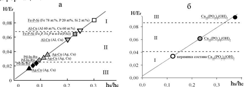
Рис. 1 - Диаграмма зависимости H/E_r от h_s/h_c для а – двух- и трехкомпонентных металлических систем; б – керамики состава \text{Ca}_{10}(\text{PO}_4)_6(\text{OH})_2 с аморфной (I), нанокристаллической (II) и субмикроструктурной (III) структурой
