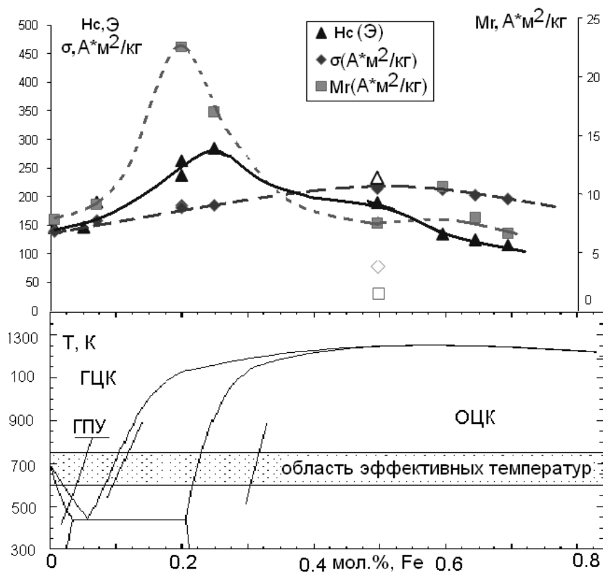
Рис. Фазовый портрет наноразмерной системы FeCo в области T_{эфф} и значения намагниченности насыщения, коэрцитивной силы и остаточной намагниченности ( \sigma , H_s , M_r ) при 5K (НБС-1 – закрашенные маркеры, НБС-2 – незакрашенные маркеры)
