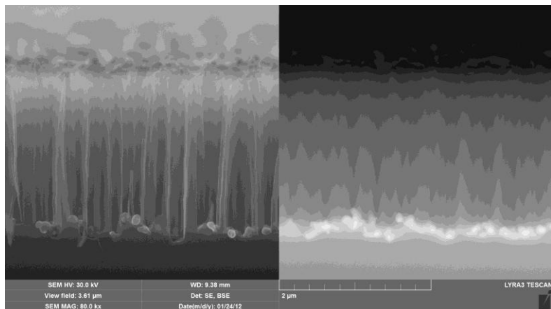
Рис. 1. Изображение в сканирующем электронном микроскопе бокового скло образца кремниевых нанонитей без удаления серебра. Слева изображение от вторичных электронов. Справа изображение от обратно рассеянных электронов.
