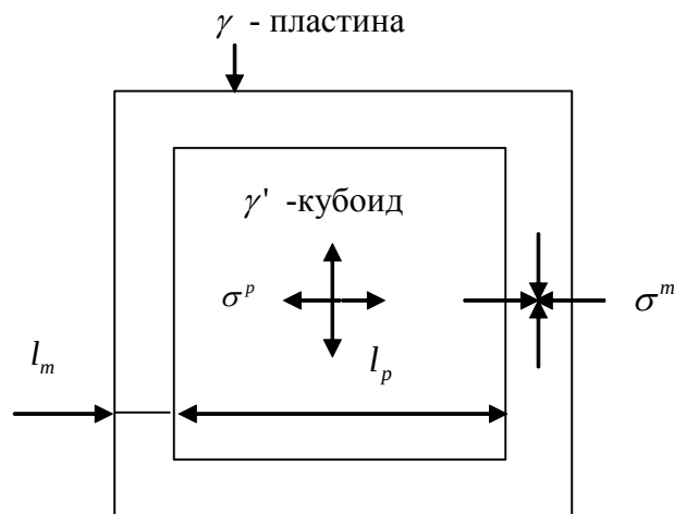
Рис.1. Периодическая ячейка \gamma'/\gamma -микроструктуры, и напряженное состояние ее элементов.
