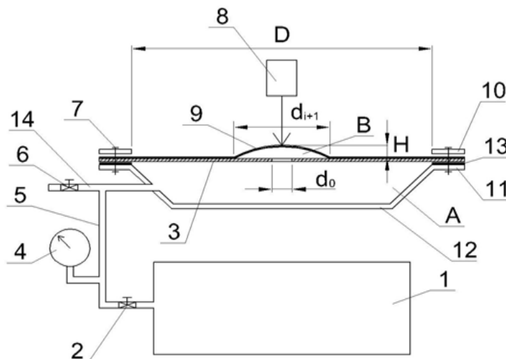
Рис.4. Схема установки.
