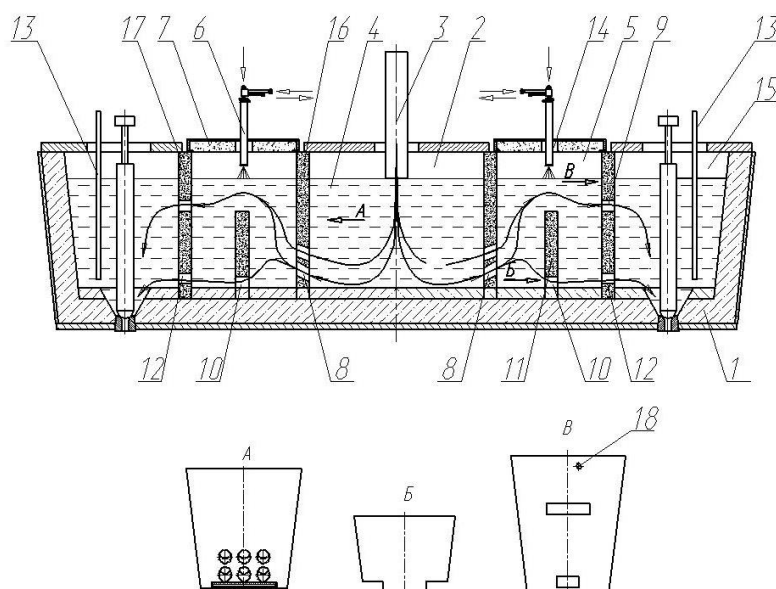
Рис.2. Плазменный подогрев стали в промковше по схеме «плазмотрон-плазмотрон».
