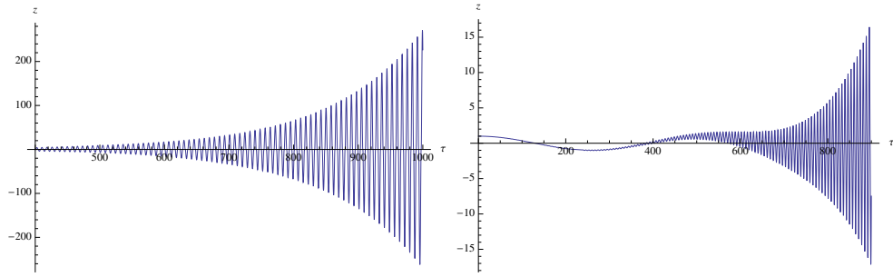
Рис. 3.12: Эффект антитрения в эволюции z(\tau) для осцилляций кривизны с пиками при y_0 = 1280 , \Omega_2/\Omega = 0.8 (слева) и y_0 = 372 , \Omega_2/\Omega = 0.9 (справа).
