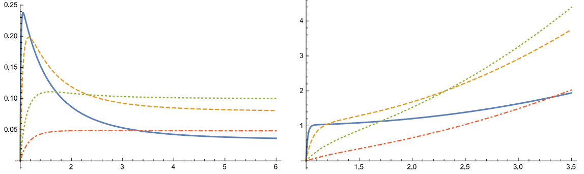
Рис. 4.1: Слева: Эволюция \xi_B(\eta) согласно уравнению (4.64), в котором C_B T_{in}^2 / (5f^2) = 0.1 , для K = N = 20 (сплошная), 5 (штриховая), 1 (пунктирная) и 0.3 (штрих-пунктирная линия). Справа: Отношение \xi_B(\eta) к его равновесному значению \xi_B^{eq}(\eta) , определенному в Ур. (4.65), для тех же значений параметров.
