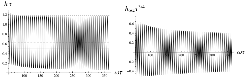
Рис. 2.15: Численное решение для безразмерного параметра Хаббла h с начальными условиями (2.117). На левом рисунке колебания имеют почти постоянную амплитуду, в то время как на правом рисунке амплитуда явно уменьшается.
