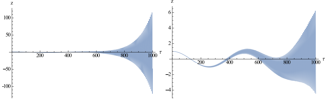
Рис. 3.4: Возбуждение параметрического резонанса z(\tau) для осцилляций кривизны с пиками при y_0 = 30 и \Omega_2/\Omega = 1/2 (слева) и \Omega_2/\Omega = 0.496 (справа).
