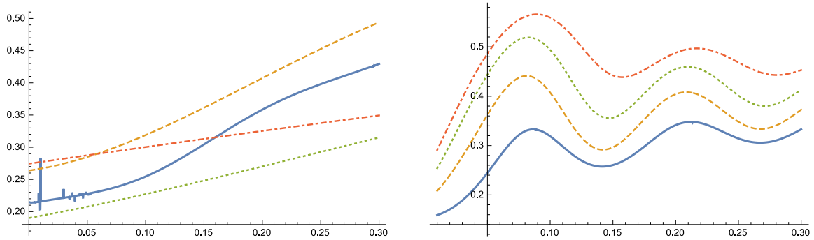
Рис. 4.4: Слева: Относительная разность \zeta = \Xi/(\dot{\theta}/T) - 1 как функция \dot{\theta}/T при фиксированном \ddot{\theta}/T^2 = 0.1 для следующих обрезаний интеграла по времени: \tau = 30 (сплошная линия), 10 (штриховая), 5 (пунктирная), 3 (штрихпунктирная). Справа: Та же разность как функция \ddot{\theta}/T^2 для фиксированного интегрирования по времени до \tau = 10 и различных \dot{\theta}/T : 0.1 (сплошная линия), 0.2 (штриховая), 0.3 (пунктирная), 0.4 (штрихпунктирная).
