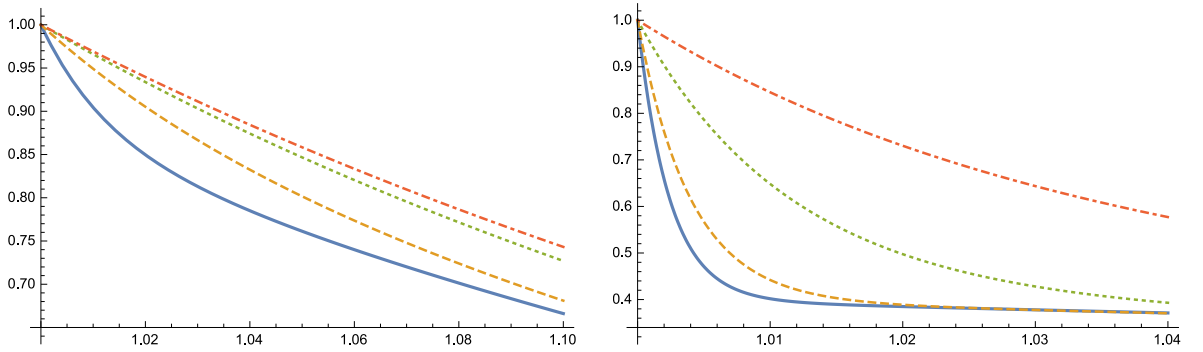
Рис. 4.2: Слева: Эволюция \dot{\theta}(\eta) , нормированного на его начальное значение \dot{\theta}_{in} , для C_B T_{in}^2 / (5f^2) = 0.1 и K = N = 20 (сплошная), 5 (штриховая), 1 (пунктирная) и 0.3 (штрих-пунктирная линия). Справа: То же для C_B T_{in}^2 / (5f^2) = 1 и K = N = 50 (сплошная), 30 (штриховая), 10 (пунктирная) и 3 (штрих-пунктирная линия).
