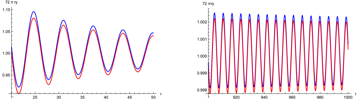
Рис. 2.9: Сравнение решений дифференциального уравнения (2.52) при w = 0 : интегральное решение (2.53) (синим) и асимптотическое решение (2.54) (красным). Безразмерная плотность энергии 72\pi\tau y(\tau) представлена для умеренно больших \tau (слева) и для очень больших \tau (справа). Согласие очень хорошее.
