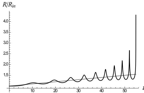
Рис. 1.2: Безразмерный скаляр кривизны R/R_{in} при n = 3 , \kappa = 0.01 , \rho_m/\rho_c = 10^5 .
