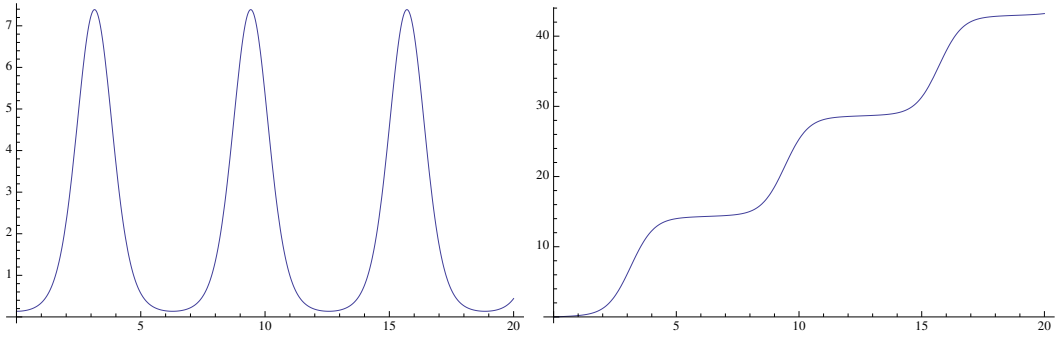
Рис. 3.7: Функция z(\tau) (справа) и ее производная z'(\tau) (слева) из Ур. (3.140) при C_0 = 1 , C_1 = C_2 = 0 , y(\tau) = y_0 \cos(\tau) и \alpha y_0 = 2 .
