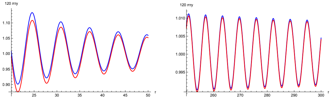
Рис. 2.8: Сравнение численного решения для безразмерной плотности энергии 120\pi y(\tau) (синим) для w = 1/3 с асимптотическим выражением (2.49) (красным) для умеренно больших \tau (слева) и для очень больших \tau (справа).
