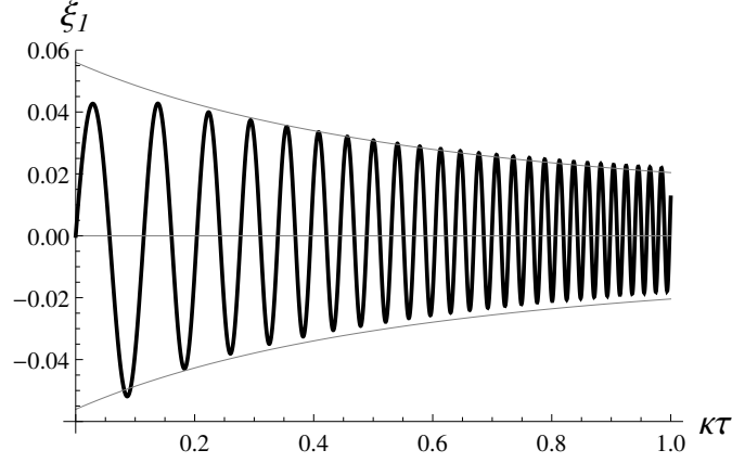
Рис. 1.4: Осцилляции \xi_1(\tau) в случае n = 2 , \kappa = 0.01 , g = 0.01 при начальных условиях y_0 = 1 , y'_0 = \kappa/2 . Амплитуда осцилляций находится в очень хорошем согласии с аналитической оценкой (1.28).
