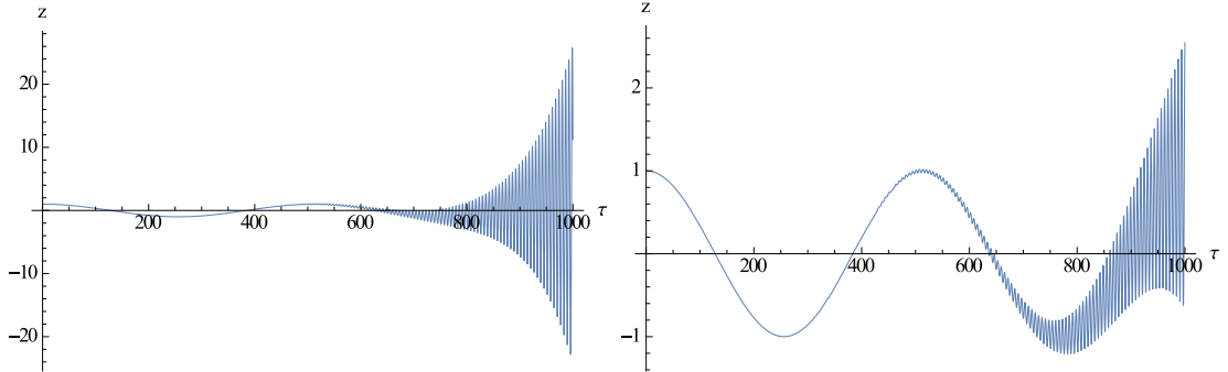
Рис. 3.5: Возбуждение параметрического резонанса z(\tau) для осцилляций кривизны с пиками при y_0 = 30 и \Omega_2/\Omega = 1 (слева) и \Omega_2/\Omega = 0.992 (справа).
