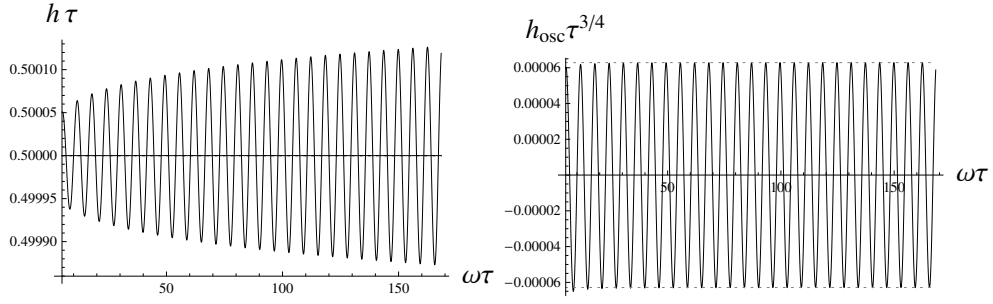
Рис. 2.10: Численное решение системы (2.95) при \delta h_0 = 10^{-4} , \delta h'_0 = 0 , y_0 = 1 и \omega = 10 . Для функциональной формы (2.116) лучше всего подходит \alpha \simeq 1 , \beta \simeq 6.29 \times 10^{-5} .
