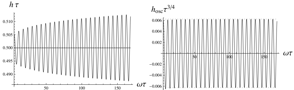
Рис. 2.12: Численное решение системы (2.95) при \delta h_0 = 10^{-2} , \delta h'_0 = 0 , y_0 = 1 , \omega = 10 . Лучше всего подходит \alpha \simeq 1 , \beta \simeq 6.26 \times 10^{-3} .
