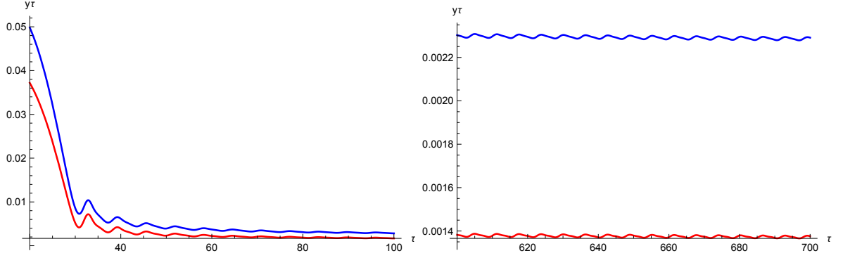
Рис. 2.6: Эволюция безразмерной плотности энергии материи y\tau при малых \tau (слева) и при больших \tau (справа) для w = 1/3 (красным) и w = 0 (синим).
