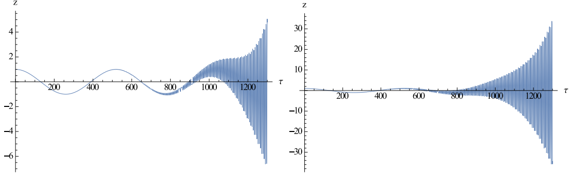
Рис. 3.6: Возбуждение параметрического резонанса z(\tau) для осцилляций кривизны с пиками при y_0 = 30 и \Omega_2/\Omega = 1/3 (слева) и \Omega_2/\Omega = 1/4 (справа).
