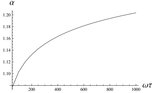
Рис. 2.14: Эволюция \alpha со временем. Начальные условия те же, что и на Рис. 2.13.
