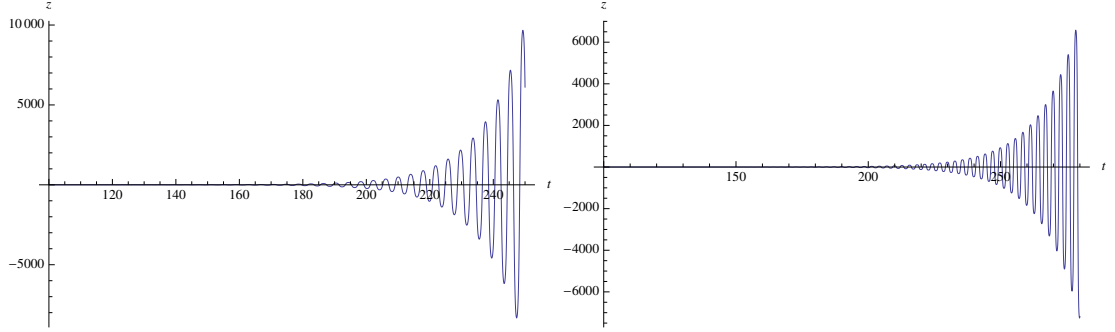
Рис. 3.9: Эффект антитрения в эволюции z(\tau) для гармонических осцилляций кривизны с y_0 = 169 , \Omega_1/\Omega = 3.2 (слева) и y_0 = 267 , \Omega_2/\Omega = 4.4 (справа). Малые радиусы: \chi = 0.01 .
