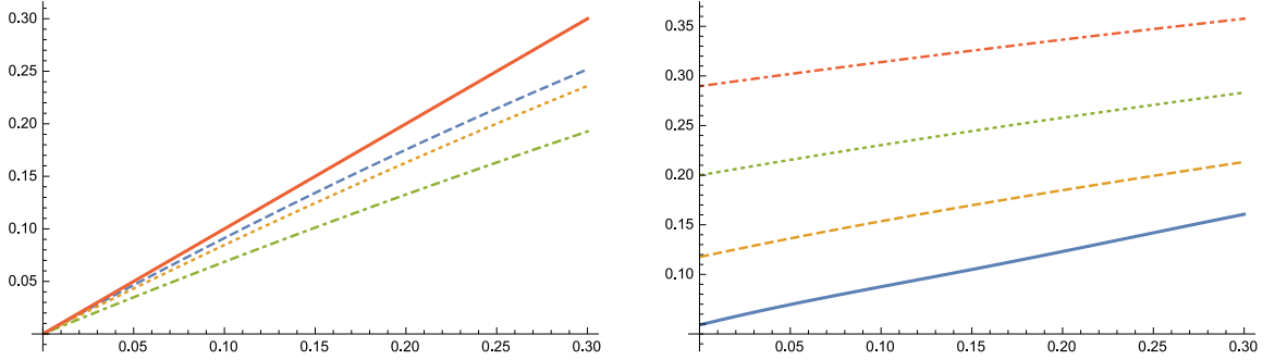
Рис. 4.3: Слева: Правая часть уравнения (4.82), обозначенная \Xi , как функция \dot{\theta}/T , для следующих обрезаний интеграла по времени в Ур. (4.83): \tau \equiv t_{max}T = 30 (штриховая линия); 10 (пунктирная); 3 (штрихпунктирная) и \dot{\theta}/T (сплошная линия). Справа: Относительная разность: \zeta = \Xi/(\dot{\theta}/T) - 1 , как функция \dot{\theta}/T для \tau = 30 (сплошная линия), 10 (штриховая), 5 (пунктирная), 3 (штрихпунктирная).
