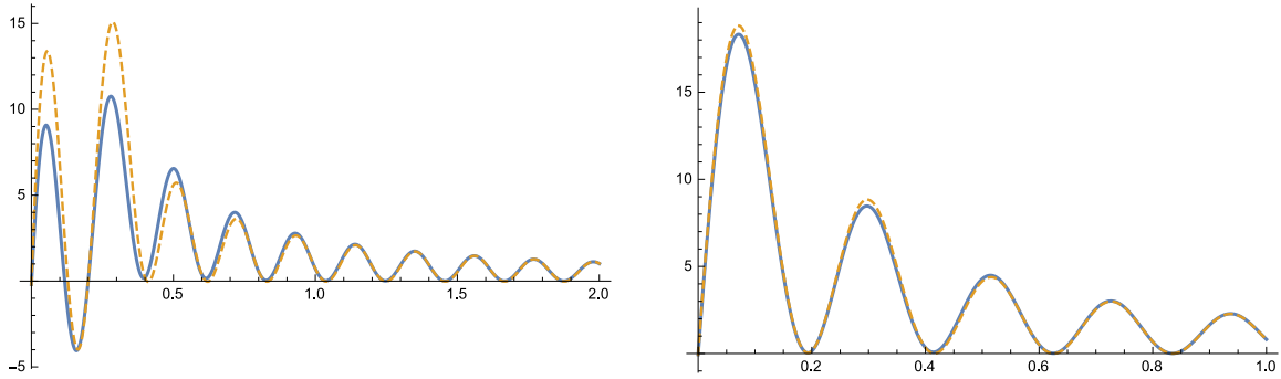
Рис. 4.5: Точное (сплошная линия) и приближенное (штриховая линия) выражения для амплитуды A (4.72) с \theta(t) , заданным уравнением (4.88), как функции mt для \theta_0 = 1 (слева) и \theta_0 = 0.3 (справа).
