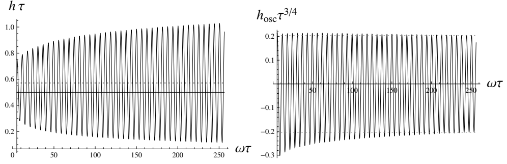
Рис. 2.13: Численное решение системы (2.95) при \delta h_0 = 0.5 , \delta h'_0 = 0 , y_0 = 1 , \omega = 10 . На больших временах лучше всего подходит \alpha \simeq 1.14 (показано пунктиров на левом рисунке), \beta \simeq 0.20 . Отметим, что на правом рисунке осциллирующая часть h не убывает точно как \tau^{-3/4} . Очевидная асимметрия верхней и нижней частей в h_{osc} обусловлена тем, что \alpha является функцией времени, и мы центрировали осцилляции вокруг ее значения в поздние времена.
