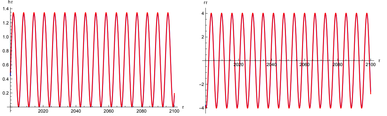
Рис. 2.7: Слева: Сравнение численного решения h\tau (красным) с аналитической оценкой (2.40) (синим). Справа: То же для численно полученного r\tau и аналитического результата (2.41). Не видно никакой разницы между красными и синими кривыми.
