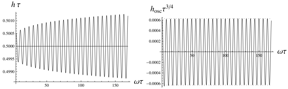
Рис. 2.11: Численное решение системы (2.95) при \delta h_0 = 10^{-3} , \delta h'_0 = 0 , y_0 = 1 , \omega = 10 . Лучше всего подходит \alpha \simeq 1 , \beta \simeq 6.28 \times 10^{-4} .
