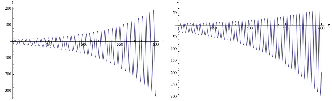
Рис. 3.11: Эффект антитрения в эволюции z(\tau) для осцилляций кривизны с пиками при y_0 = 400 , \Omega_2/\Omega = 0.6 (слева) и y_0 = 702 , \Omega_2/\Omega = 0.7 (справа).
