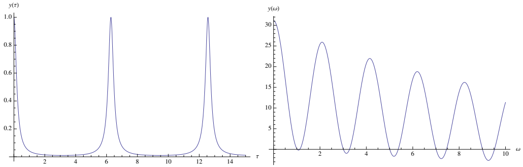
Рис. 3.3: Слева: y(\tau) из уравнения (3.136) с y_0 = 1 , \Omega_2 = 0.5 и d = 0.1 . Справа: Фурье образ y(\tau) .
