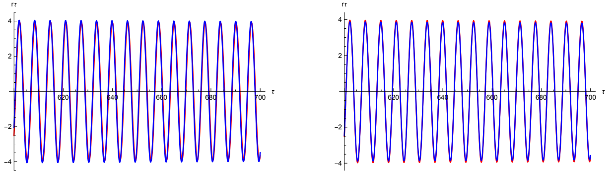
Рис. 2.4: Эволюция безразмерного скаляра кривизны \tau r(\tau) в пост-инфляционную эпоху. Слева ( w=1/3 ): r_{in} = -300 (красным), r_{in} = -600 (синим). Не видно никакой разницы между кривыми. Справа ( r_{in} = -300 ): w = 1/3 (красным) и w = 0 (синим). Разница между кривыми ничтожно мала.
