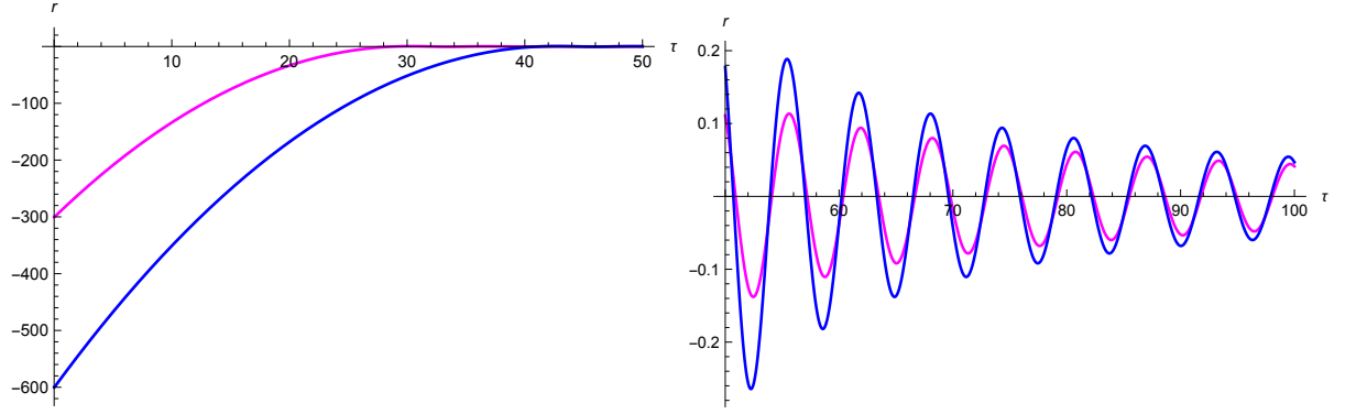
Рис. 2.3: Эволюция безразмерного скаляра кривизны для r_{in} = -300 (фиолетовым) и r_{in} = -600 (синим). Слева : эволюция во время инфляции. Справа : эволюция после окончания инфляции, скаляр кривизны осциллирует.
