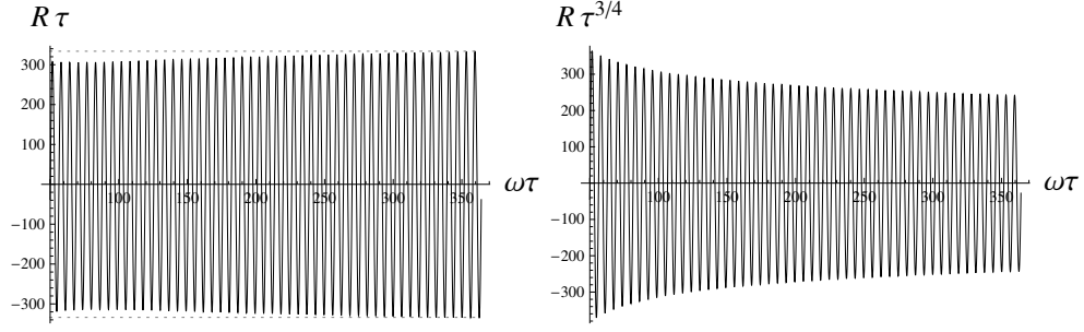
Рис. 2.16: Численное решение для безразмерного скаляра кривизны r с начальными условиями (2.117).
