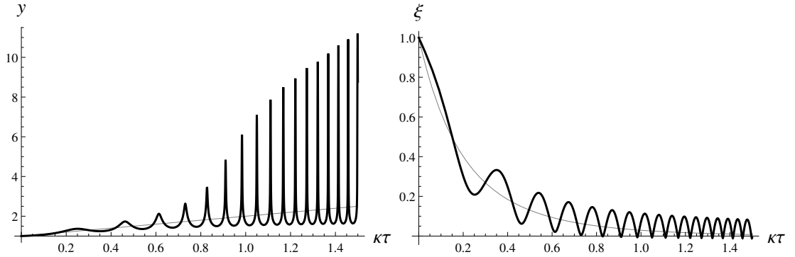
Рис. 1.5: «Пики» в решениях. Результаты представлены для n = 2 , g = 0.001 , \kappa = 0.04 , и y'_0 = \kappa/2 . Отметим асимметрию осцилляций y вокруг y = z и их негармоничность.
