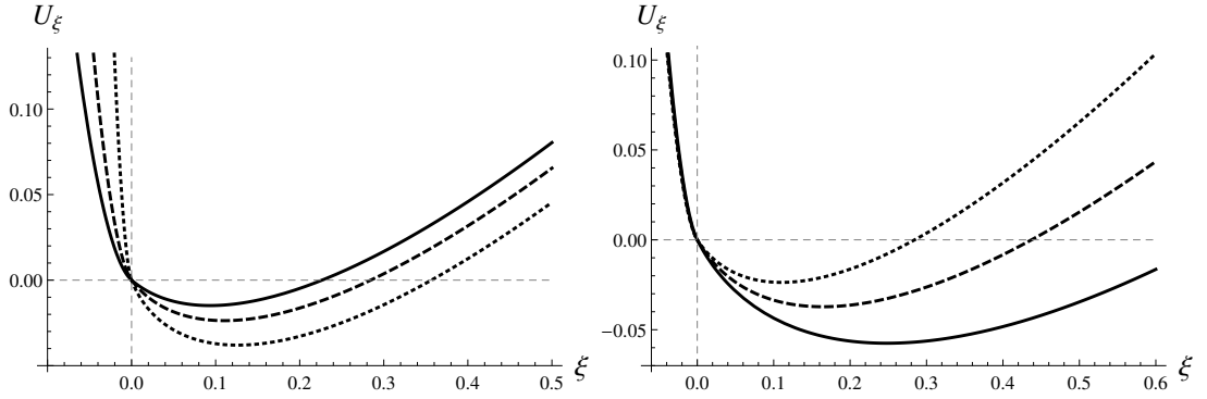
Рис. 1.3: Примеры изменения потенциала (1.33) как функции \xi для разных значений параметров. Слева ( n = 2 , z = 1.5 ) сплошная линия: g = 0.02 , штриховая линия: g = 0.01 , пунктирная линия: g = 0.002 ; часть потенциала при \xi < \xi_{min} ( \xi_{min} определено в Ур. (1.28)) становится более крутой с уменьшением g ; дно потенциала смещается к нулю. Справа ( n = 2 , g = 0.01 ) сплошная линия: z = 1.3 , штриховая линия: z = 1.4 , пунктирная линия: z = 1.5 ; при возрастании z дно потенциала движется к большим значениям U и меньшим значениям \xi .
