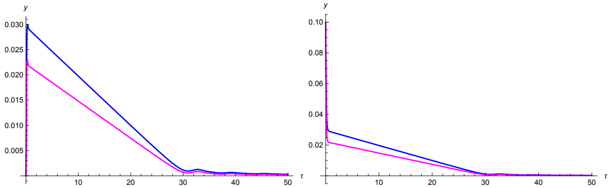
Рис. 2.2: Эволюция безразмерной плотности энергии материи во время инфляции для w = 0 (синим) и w = 1/3 (фиолетовым). Слева: y_{in} = 0 , справа: y_{in} = 0.1 . Результаты нечувствительны к виду S[r] , поскольку при инфляции y(\tau) быстро стремится к нулю.
