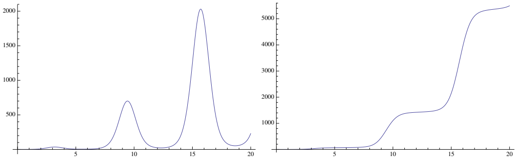
Рис. 3.8: Функция z(\tau) (справа) и ее производная z'(\tau) (слева) из Ур. (3.140) при C_2 = 1 , C_0 = C_1 = 0 , y(\tau) = y_0 \cos(\tau) , and \alpha y_0 = 2 .
