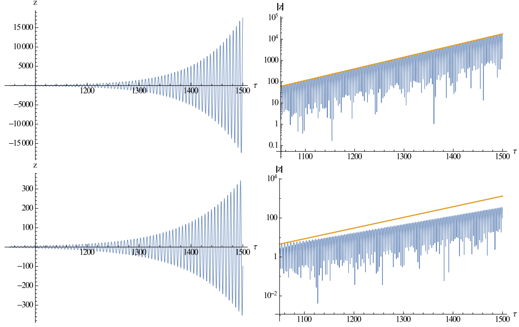
Рис. 3.1: Решения для параметров (3.134). Слева : Осцилляции z как функция безразмерного времени \tau . Справа : |z(\tau)| (в логаримическом масштабе) и, оранжевым, амплитуда осцилляций (3.133) с темпом роста, определяемым (3.130). Сверху : Возбуждение параметрического резонанса z(\tau) для гармонических осцилляций кривизны с y_0 = 5 и \Omega_1/\Omega = 2 и сравнение с предсказанным экспоненциальным ростом. Относительная разность между точным и оценочным темпами роста около 5 \times 10^{-5} . Снизу : Результаты для \Omega_1/\Omega = 2.015 , другие параметры неизменны. Резонансное поведение намного слабее, но согласие между численным значением \Gamma и аналитической оценкой (оранжевым) удовлетворительное: |\Gamma_{\text{res}}/\Gamma_{\text{num}} - 1| \sim 0.24 . Заметим, что хотя решения показаны при относительно больших временах, эволюция системы начинается при \tau = 0 .
