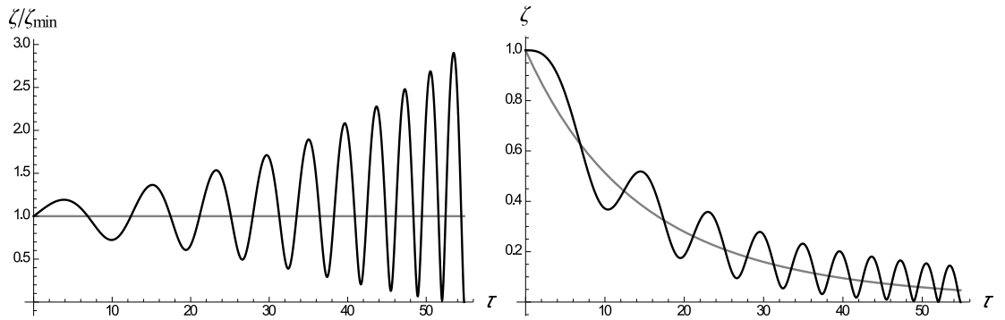
Рис. 1.1: Слева: отношение \zeta/\zeta_{min} , справа: функции \zeta (осциллирующая) и \zeta_{min} (гладкая) в зависимости от времени \tau при n = 3 , \kappa = 0.01 , \rho_m/\rho_c = 10^5 .
