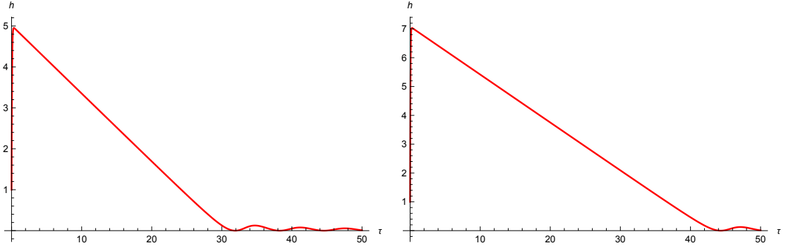
Рис. 2.1: Эволюция h(\tau) на инфляционной стадии с начальными значениями безразмерной кривизны r = 300 (слева) и 600 (справа). Исходно h берется равным нулю, h_{in} = 0 , но быстро достигает значения, определяемого Ур. (2.22), h(0) = \sqrt{-r_0/12} . Показатели экспоненты, согласно Ур. (2.21), равны, соответственно, 75 и 150 .
