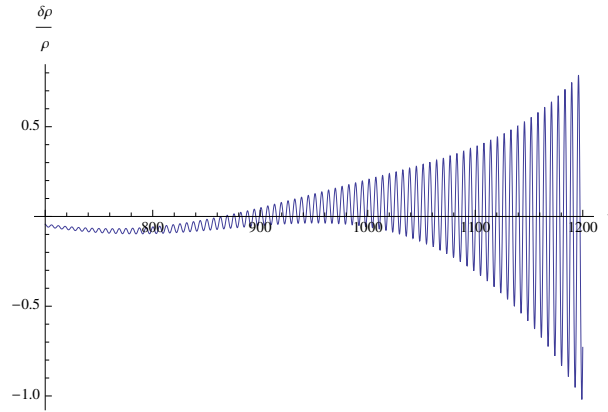
Рис. 3.14: Эволюция \delta\rho/\rho в области параметрического резонанса, индуцированного решениями с пиками при y_0 = 30 , \Omega_2/\Omega = 0.5 . Начальное значение возмущений метрики \delta B(0) \equiv z(0) = 10^{-3} .
