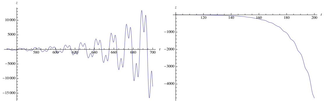
Рис. 3.13: Эффект антитрения в эволюции z(\tau) для осцилляций кривизны с пиками при y_0 = 14 , \Omega_2/\Omega = 0.4 (слева) и y_0 = 9 , \Omega_2/\Omega = 0.6 (справа). Большие радиусы: \chi = 10 .
