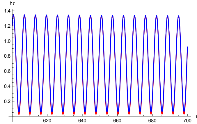
Рис. 2.5: Эволюция безразмерного параметра Хаббла h\tau в пост-инфляционную эпоху для w = 1/3 (красным) и w = 0 (синим).
