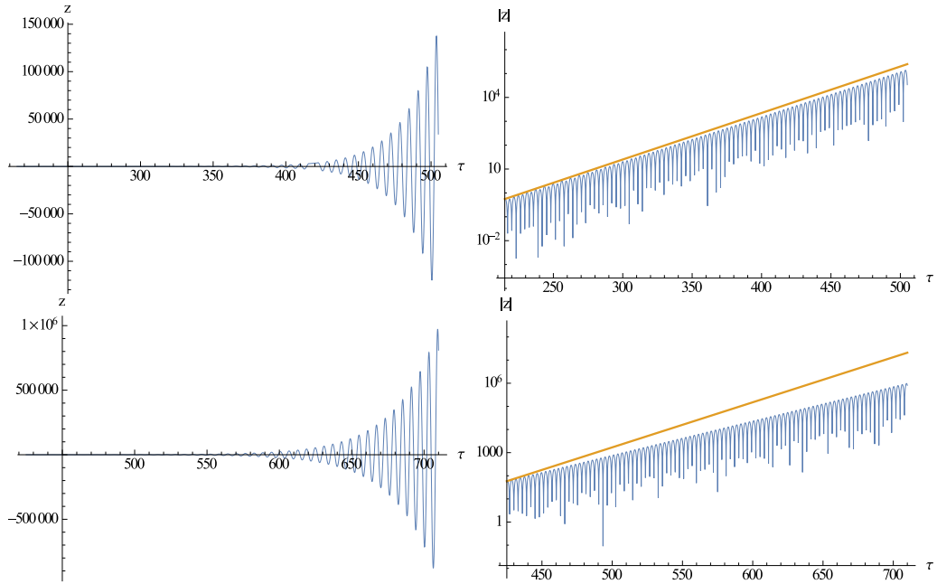
Рис. 3.2: Решения для параметров (3.135). На левой и правой панелях показаны те же величины, что и на Рис. 3.1. Сверху : Решение для y_0 = 1 и \Omega_1/\Omega = 2 и сравнение с предсказанным поведением (оранжевым). Относительная разность между точным и оценочным темпами роста \sim 3 \times 10^{-2} . Снизу : Результаты для \Omega_1/\Omega = 2.075 , другие параметры неизменны. Резонансное поведение слабее, но все еще достаточно сильное, однако согласие между численным значением \Gamma и аналитической оценкой (оранжевым) уменьшается: |\Gamma_{\text{res}}/\Gamma_{\text{num}} - 1| \sim 0.32 . Тем не менее, наши аналитические оценки находятся в пределах одного порядка от численных результатов.
