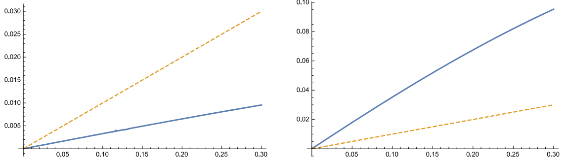
Рис. 4.6: Слева : Сплошная линия: правая часть уравнения (4.82), \Xi , при m/T = 0.1 и максимальном пределе интегрирования по времени \tau = 30 ; штриховая линия: \dot{\theta}/T как функция \theta_0 , см. Ур. (4.87). Справа : То же самое при максимальном пределе интегрирования по времени \tau = 3 .
