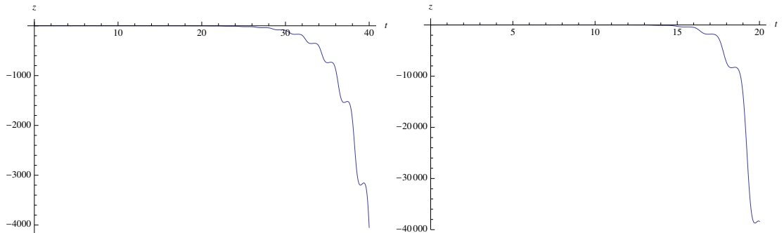
Рис. 3.10: Эффект антитрения в эволюции z(\tau) для гармонических осцилляций кривизны с y_0 = 10 , \Omega_1/\Omega = 3.2 (слева) и y_0 = 11 , \Omega_2/\Omega = 4.4 (справа). Большие радиусы: \chi = 10 .
