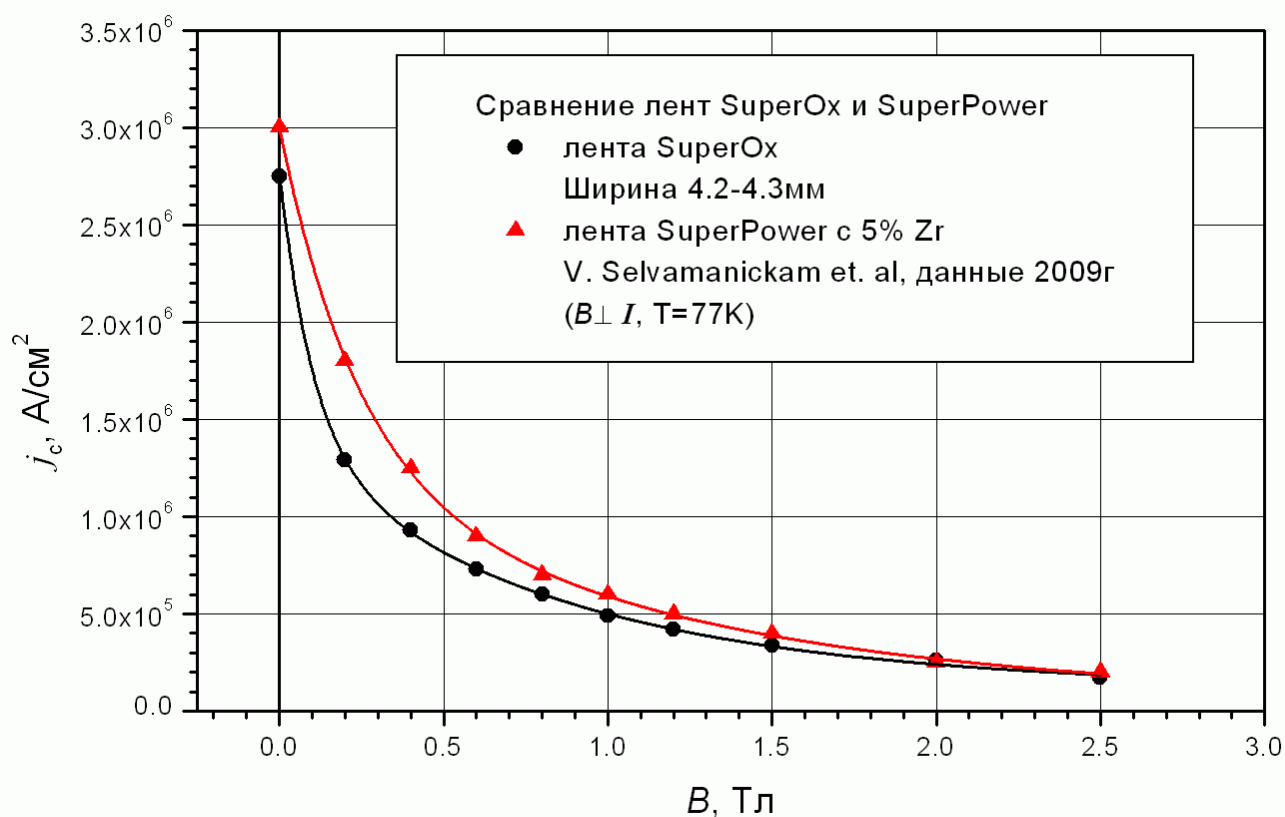
Рис. 5.4. Сравнение зависимостей j_c(B) , полученных в геометрии B \perp I при T = 77 К, для ВТСП лент на основе GdBa_2Cu_3O_{7-x} (●) и YBa_2Cu_3O_{7-x} (▲).
