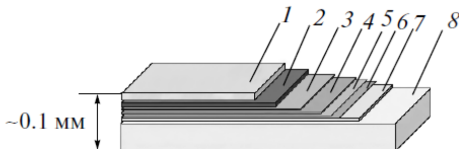
Рис. 3.9. Архитектура ВТСП ленты SF12100 производства SuperPower Inc. (USA): 1 – серебро, 2 мкм; 2 – сверхпроводник YBCO (123), 1 мкм; 3–7 – буферные слои, состоящие из эпитаксиальных диэлектрических пленок; 8 – подложка из сплава хастеллой, 100 мкм.
