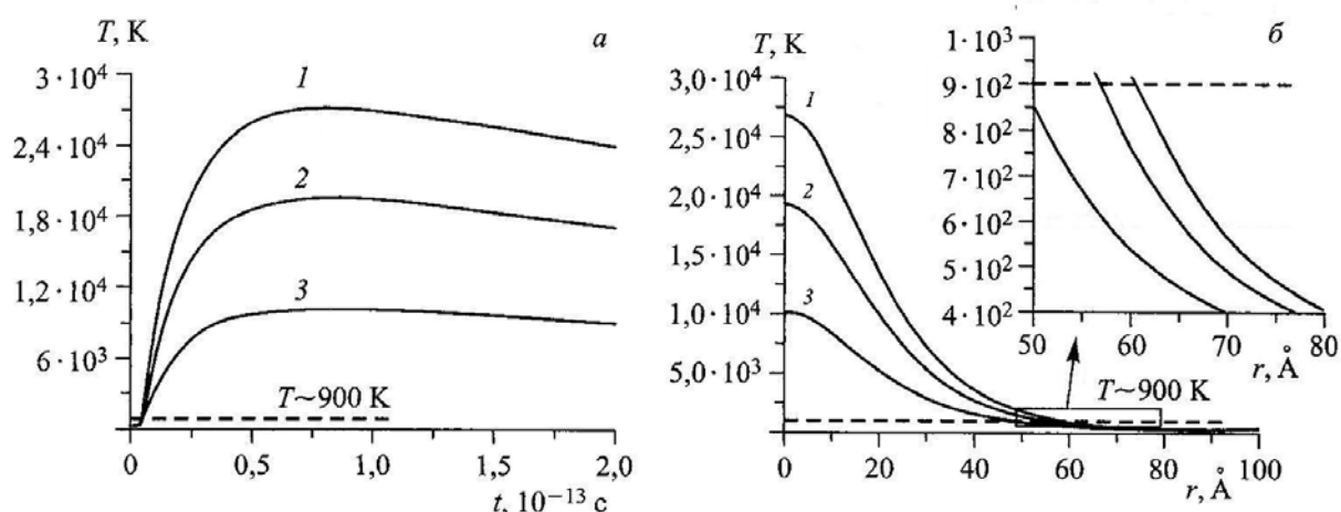
Рис. 3.5. Кинетические зависимости температуры решетки слоя ВТСП (а) и радиальные профили температуры в этом слое в момент времени t=10^{-13} с (б) при облучении ионами Xe (167 МэВ) – 1, Kr (107 МэВ) – 2 и Ar (48 МэВ) – 3.
