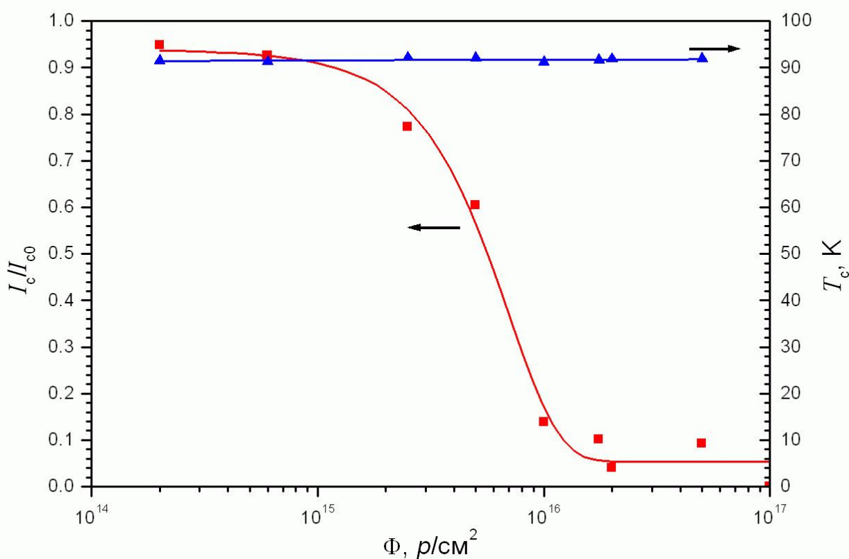
Рис. 4.5. Зависимости I_c/I_{c0}(\Phi) и T_c(\Phi) для ВТСП ленты YBCO(123). (▲) – T_c ; (■) – I_c/I_{c0} .
