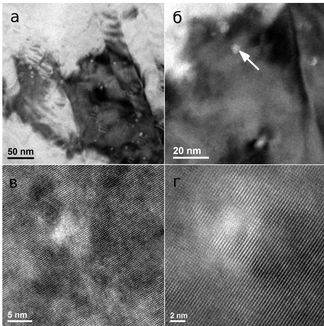
Рис. 3.8. Микрофотографии ВТСП ленты SF12100, полученные с помощью просвечивающей электронной микроскопии высокого разрешения. На изображениях б-г хорошо видны дефекты размером 3-5 нм (на б – отмечен стрелкой).
