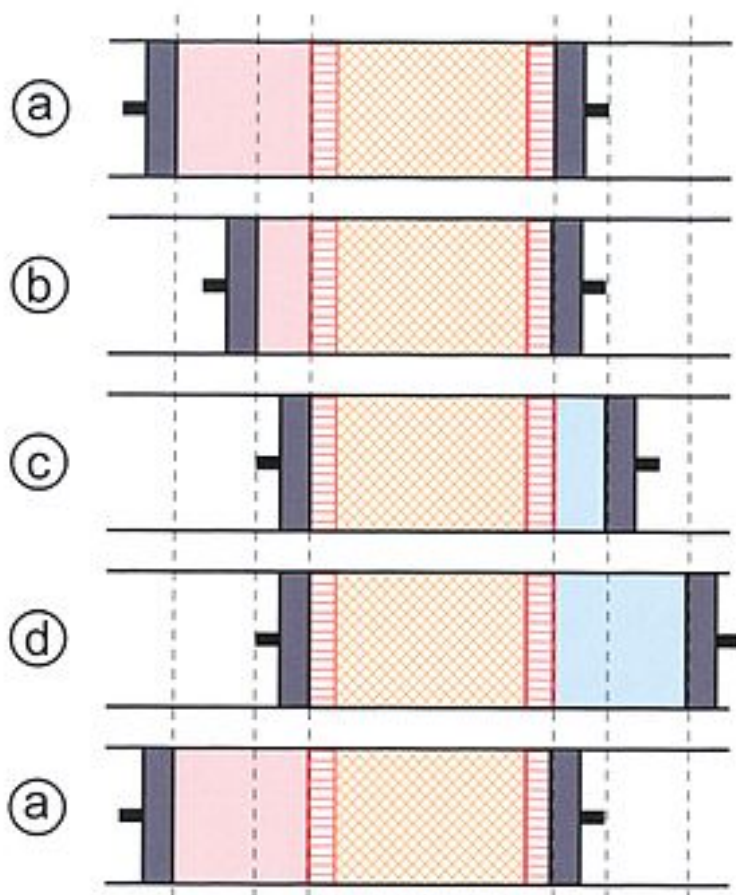
Рис. 1.11. Четыре состояния криогенной машины Стирлинга.
