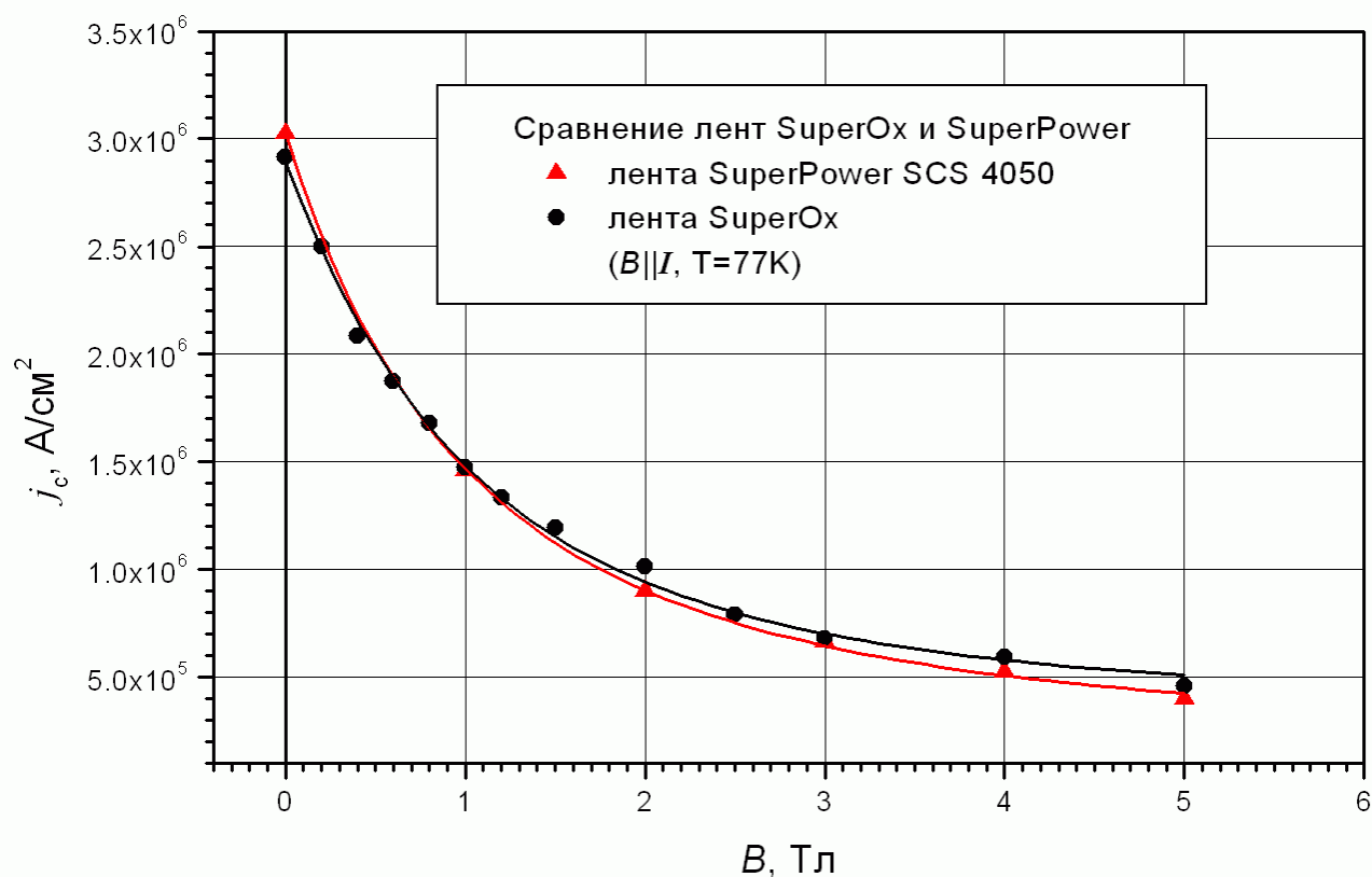
Рис. 5.5. Сравнение зависимостей j_c(B) , полученных в геометрии B||I при T=77K , для ВТСП лент на основе GdBa_2Cu_3O_{7-x} (●) и YBa_2Cu_3O_{7-x} (▲).
