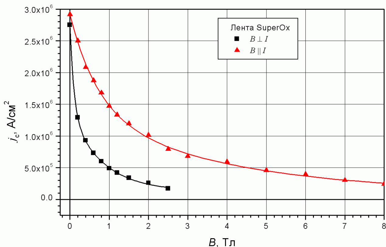
Рис. 5.3. Зависимости плотности критического тока от индукции внешнего магнитного поля для ВТСП ленты \text{GdBa}_2\text{Cu}_3\text{O}_{7-x} ( B \perp I и B \parallel I , T = 77 \text{ K} ).
