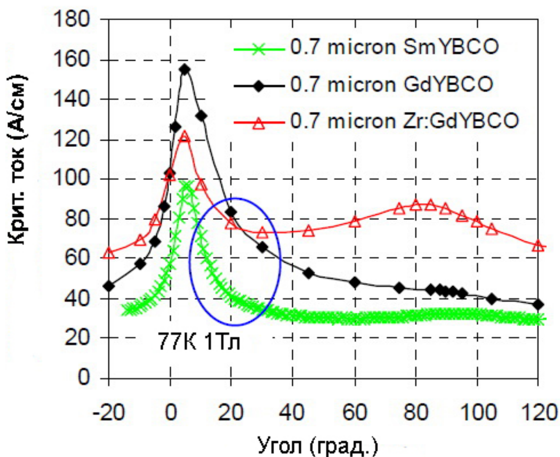
Рис. 1.20. Зависимость критического тока от угла между плоскостью ВТСП пленки и направлением магнитного поля для различных ВТСП материалов [68]. Синий овал – критическая область для производительности соленоида из ВТСП.
