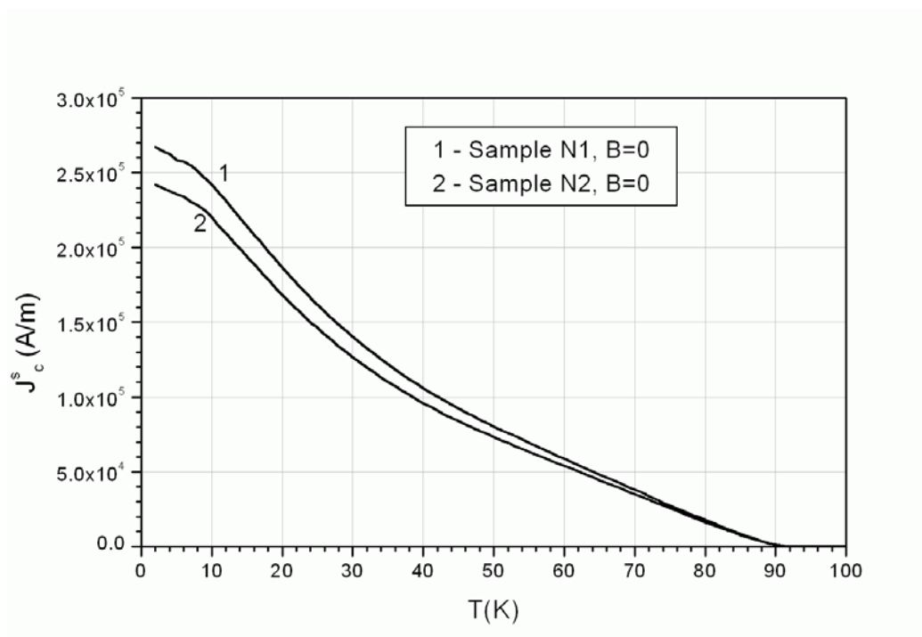
Рис. 5.6. Зависимости поверхностной плотности критического тока от температуры в отсутствие магнитного поля для двух образцов ленты на основе GdBCO, полученные с помощью СКВИД магнетометра.
