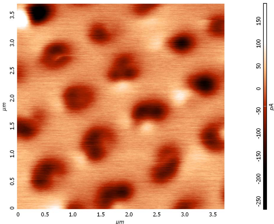
Рис. 5.16. MCM изображение участка массива трехслойных частиц диаметром 300 нм, толщины Co слоев 16/11/8 нм, толщина Si прослойки 3 нм.
