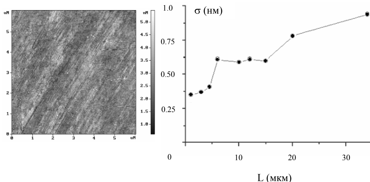
Рис. 3.16. Типичное АСМ изображения поверхности (слева) и зависимость среднеквадратичной шероховатости от размера кадра для подложки № 4.
