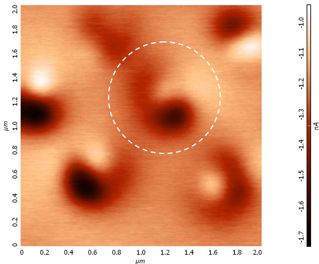
Рис. 5.17. MCM изображение участка массива трехслойных дисков диаметром 300 нм, толщины Co слоев 16/11/8 нм, толщина Si прослойки 5 нм. Частица со спиральным распределением намагниченности помечена кружком.
