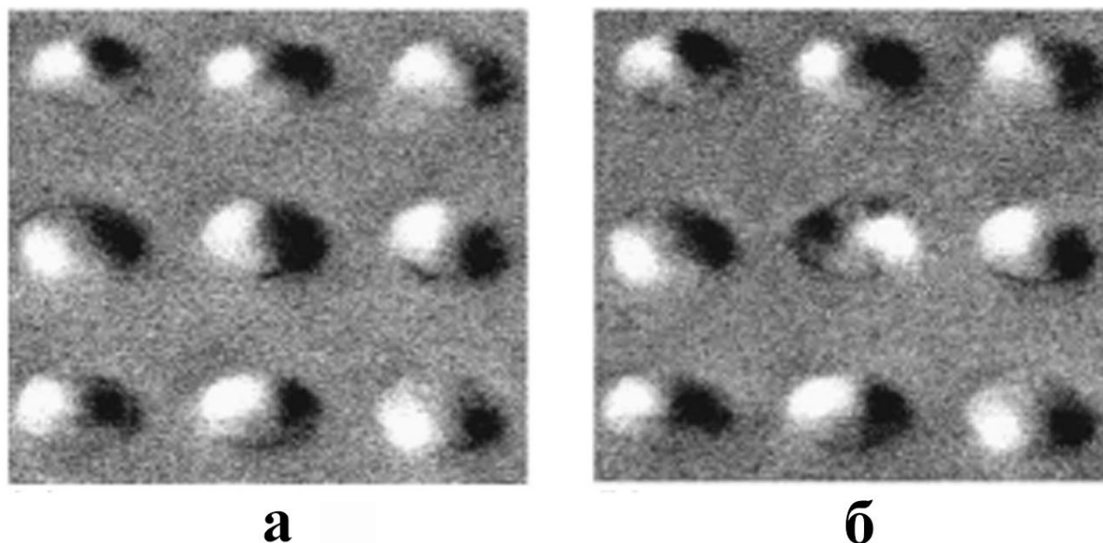
Рис. 1.9. Перемагничивание центральной частицы при помощи ее сканирования МСМ зондом во внешнем магнитном поле. (а) до перемагничивания, (б) после процедуры перемагничивания. Из работы [71].
