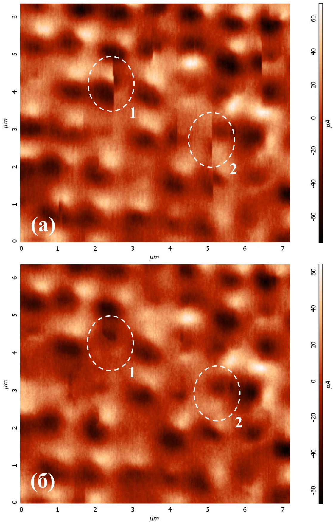
Рис. 5.7. Последовательные MCM изображения массива двухслойных ферромагнитных частиц. Изображения получены при помощи MCM зонда с большим магнитным моментом. Использовалась неконтактная MCM, высота прохода – 60 нм (а), 80 нм (б).
