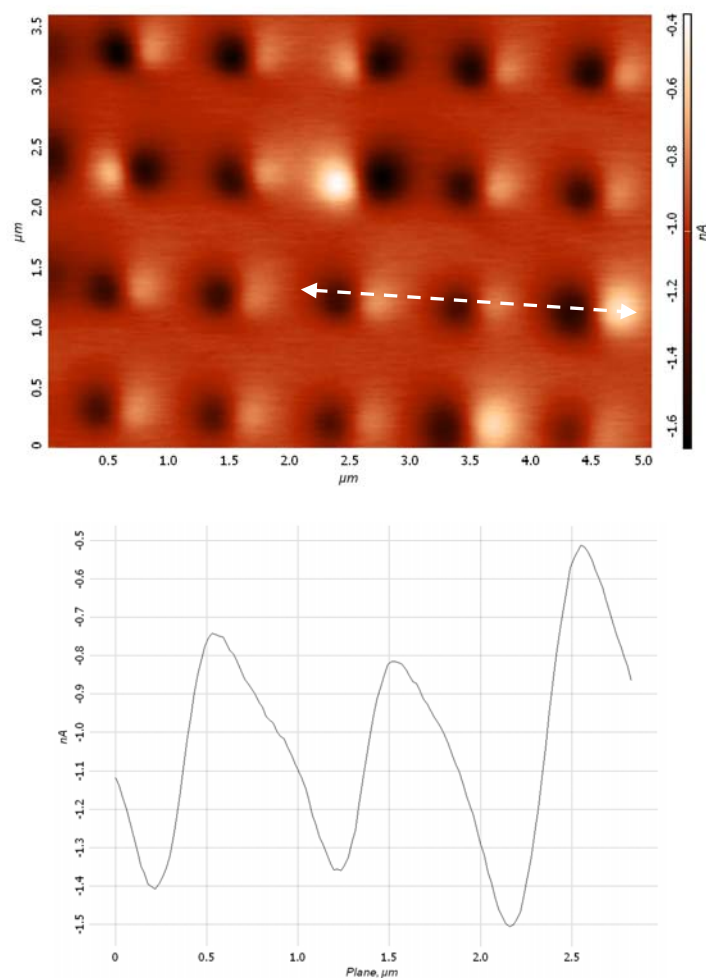
Рис. 5.2. МСМ изображение двухслойных ферромагнитных частиц размером 400 \times 250 нм, толщина каждого Со слоя 15 нм, толщина Si прослойки 3 нм (сверху). Поперечное сечение, показанное на МСМ изображении белой линией (снизу).
