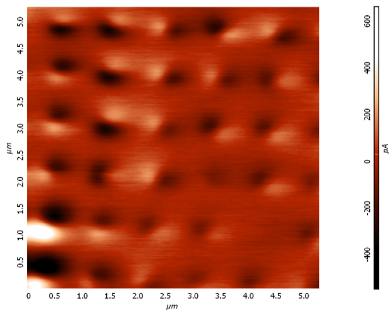
Рис. 5.3. МСМ изображение двухслойных субмикронных дисков диаметром 300 нм. Толщина каждого Со слоя 15 нм, толщина Si прослойки 3 нм.
