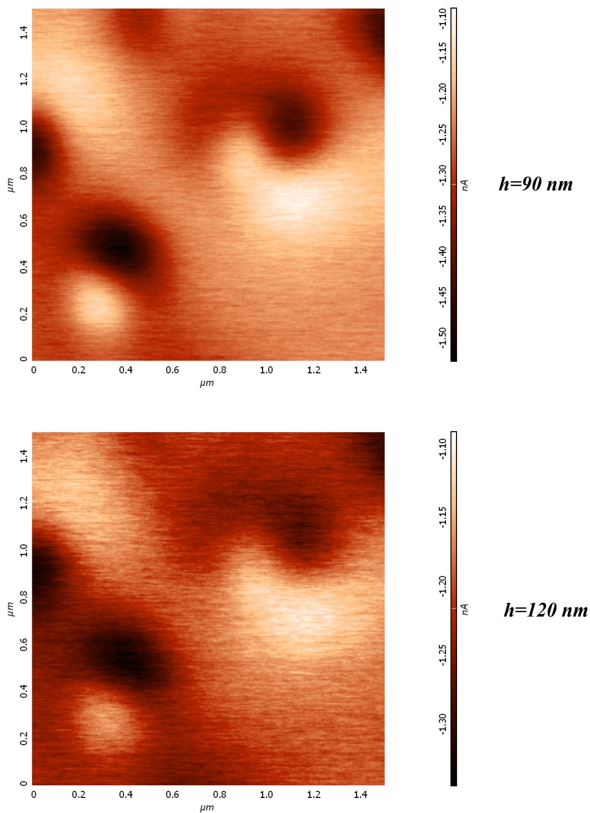
Рис. 5.19. МСМ изображения трехслойных ферромагнитных дисков, полученные при различной высоте прохода МСМ зонда над верхней гранью диска. Параметры структур: диаметр 300 нм, толщины Со слоев 16/11/8 нм, толщина Si прослойки 5 нм.
