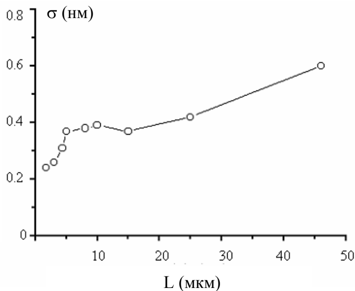
Рис. 3.13. Зависимость среднеквадратичной шероховатости от размера кадра для образца №2.
