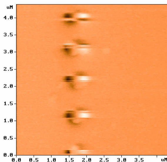
Рис. 4.8. МСМ изображения эффектов перемагничивания частиц эллиптических Со при направлении сканирования параллельном длинной оси частиц (горизонтальная ось на рисунке).
