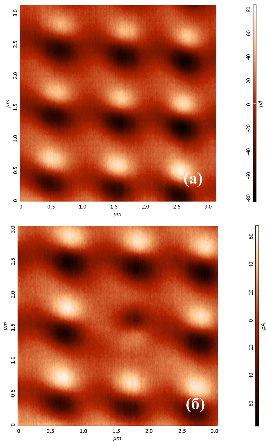
Рис. 5.8. Начальное состояние (а) и результат процедуры перемагничивания зондом МСМ центральной частицы (б).
