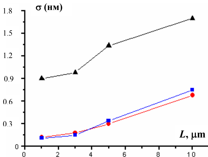
Рис.3.8. Масштабная зависимость среднеквадратичной шероховатости поверхности полимерной реплики с поверхности кремния (обозначены квадратными точками ■) на подложках из стекла. Масштабная зависимость параметра \sigma эталонной поверхности кремния показана круглыми (●) точками, а исходной поверхности стеклянной подложки треугольными (▲) точками. ( L – размер кадра).
