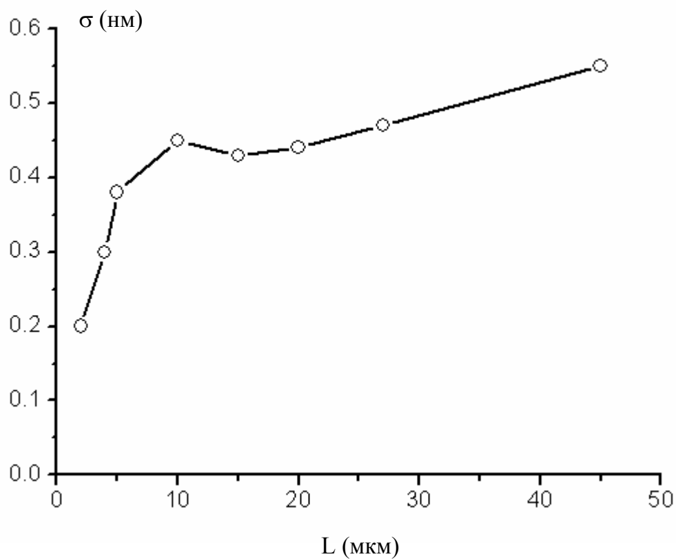
Рис. 3.14. Зависимость среднеквадратичной шероховатости от размера кадра для образца № 3.
