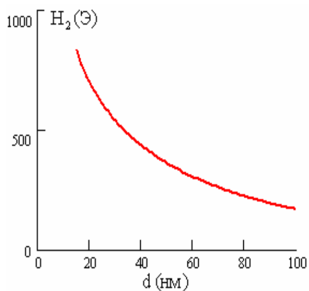
Рис. 5.10. Зависимость средней напряженности магнитного поля, создаваемого одним слоем Со в объеме другого, от расстояния между центрами слоев. Диаметр двухслойной частицы 300 нм, толщина слоев Со 20 нм.
