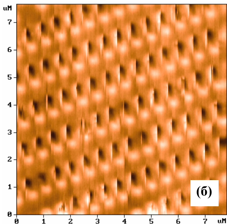
Рис. 4.4. МСМ изображения массива частиц Fe-Cr, полученные при различных направлениях сканирования. Направление сканирования совпадает с горизонтальной осью (а), с вертикальной осью (б). Использовалась 2-х проходная tapping/lift МСМ мода.
