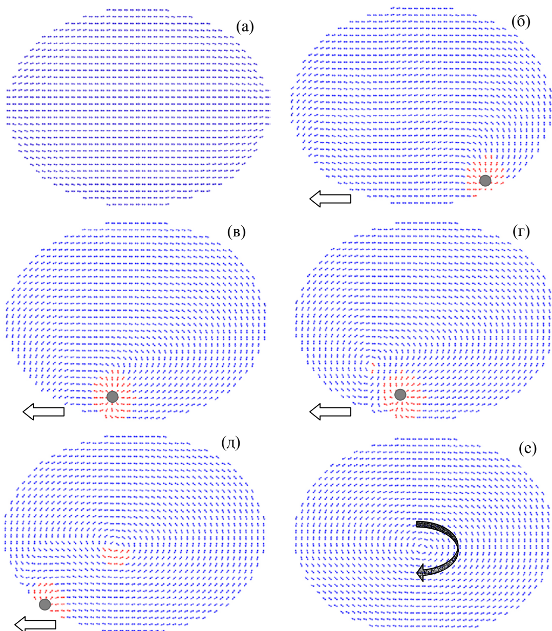
Рис. 4.12. Последовательные стадии процесса перемагничивания частицы Со при движении МСМ зонда (зонд показан серым кружком) по краю частицы. Начальное состояние частицы соответствует однородно намагниченному.
