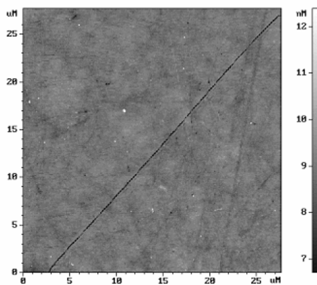
Рис. 3.15. Типичное изображение рельефа поверхности подложки № 3.
