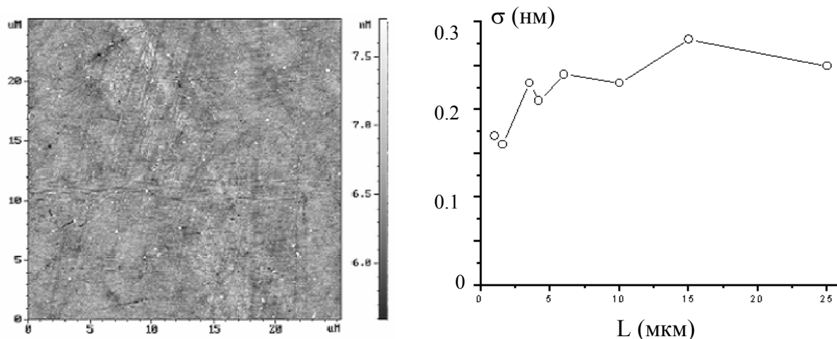
Рис. 3.19. АСМ изображение рельефа поверхности подложки № 6 и зависимость среднеквадратичной шероховатости поверхности от размера кадра после 100 часов глубокой полировки.
