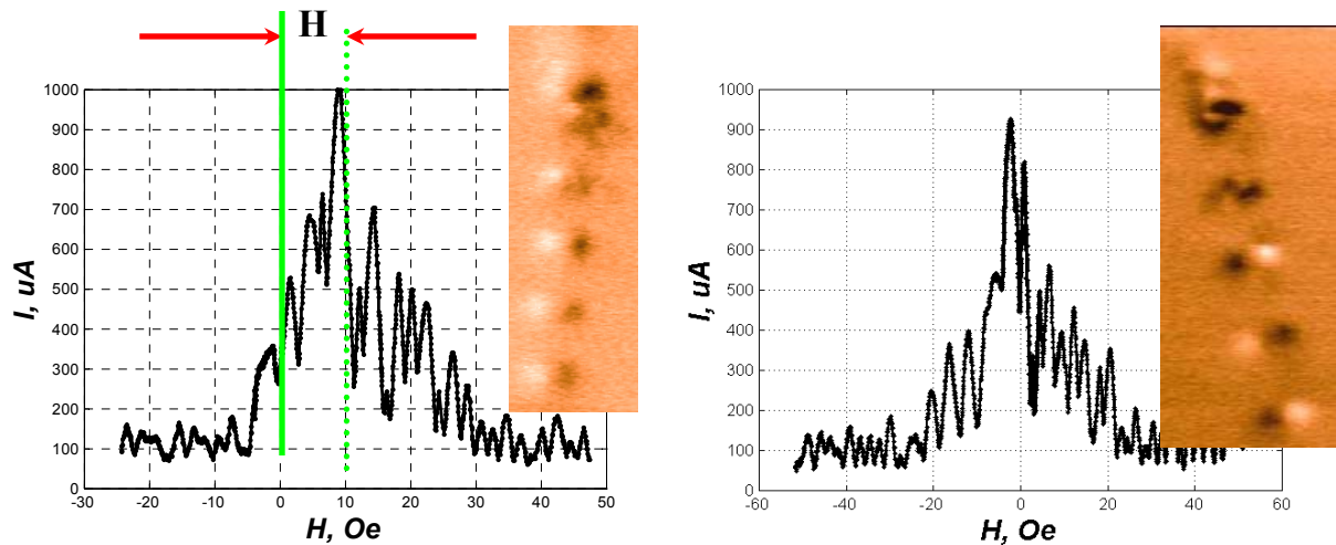
Рис. 4.15. Эффект влияния среднего поля при “ферромагнитном” упорядочении магнитных моментов частиц (слева). Зависимость I_c(H) смещена относительно нулевого значения поля на \Delta H \approx 10 Э. Отсутствие эффекта среднего поля при “антиферромагнитном” упорядочении (справа).
