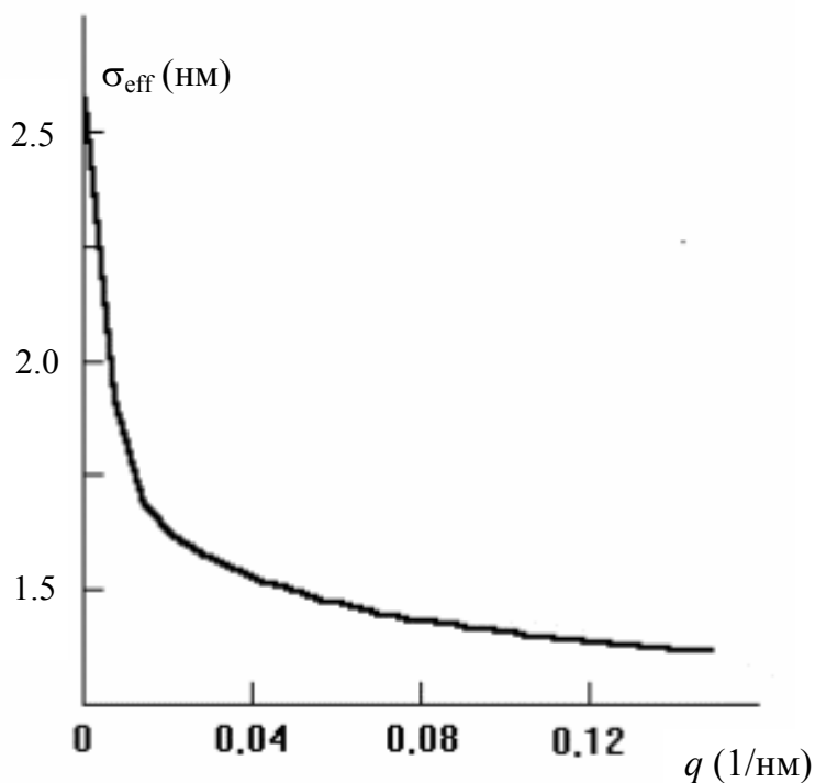
Рис. 3.4. Угловая зависимость параметра эффективной шероховатости рассчитанная непосредственно по АСМ рельефу поверхности одной из подложек. Значение \sigma_{eff} при q=0 совпадает с величиной среднеквадратичного отклонения высот рельефа, рассчитываемого по АСМ профилю поверхности.
