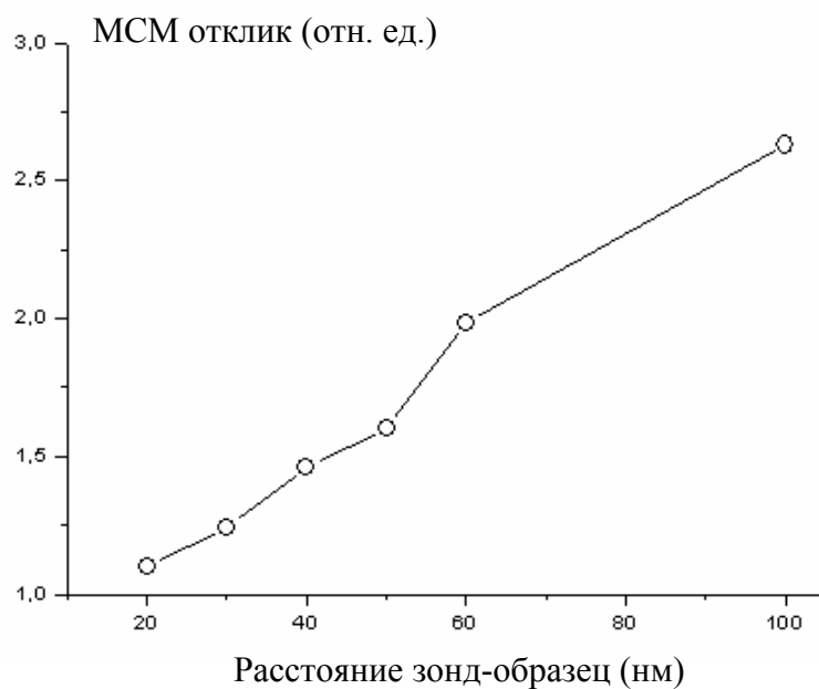
Рис. 5.6. Отношение величины \uparrow\uparrow МСМ отклика к величине \uparrow\downarrow МСМ отклика в зависимости от высоты прохода зонда.
