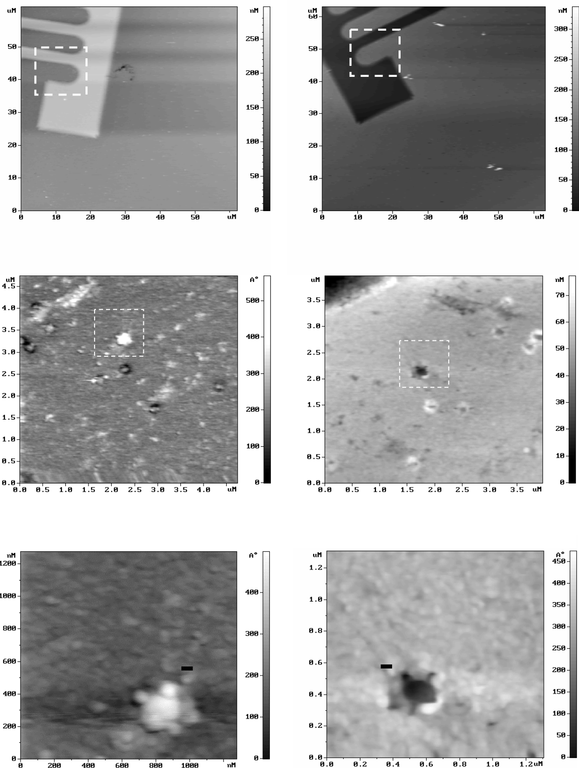
Рис. 3.10. АСМ исследования сопряженных участков поверхности эталонного образца (слева) и поверхности полимерной реплики (справа). В качестве эталонного образца использована решетка на кремнии, изготовленная методами фотолитографии. Черточка на нижних рисунках соответствует размеру 50 нм.
