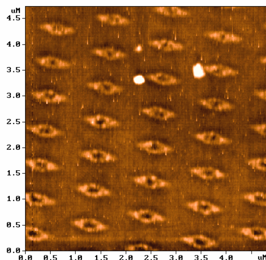
Рис. 4.1. АСМ изображение пленки Fe-Cr после проведения процедуры интерференционной лазерной литографии.
