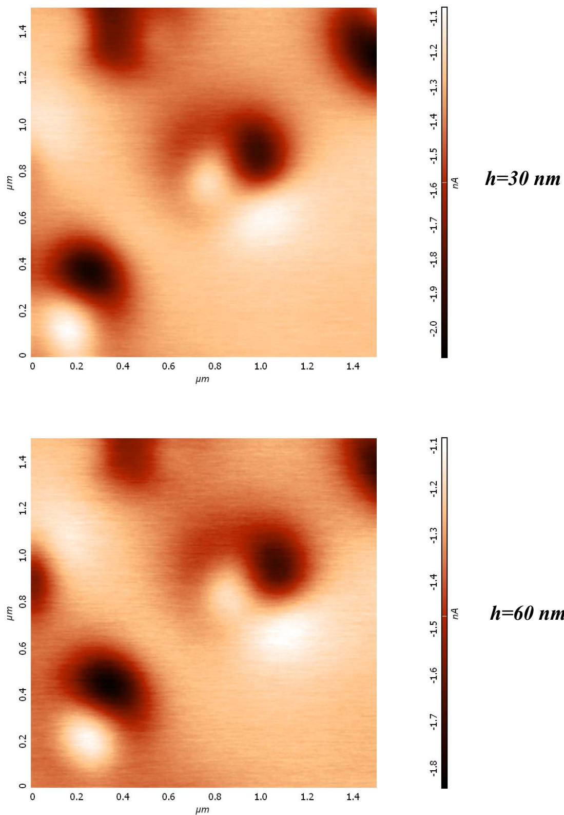
Рис. 5.18. MFM изображения трехслойных ферромагнитных дисков, полученные при различной высоте прохода MFM зонда над верхней гранью диска. Параметры структур: диаметр 300 нм, толщины Co слоев 16/11/8 нм, толщина Si прослойки 5 нм.
