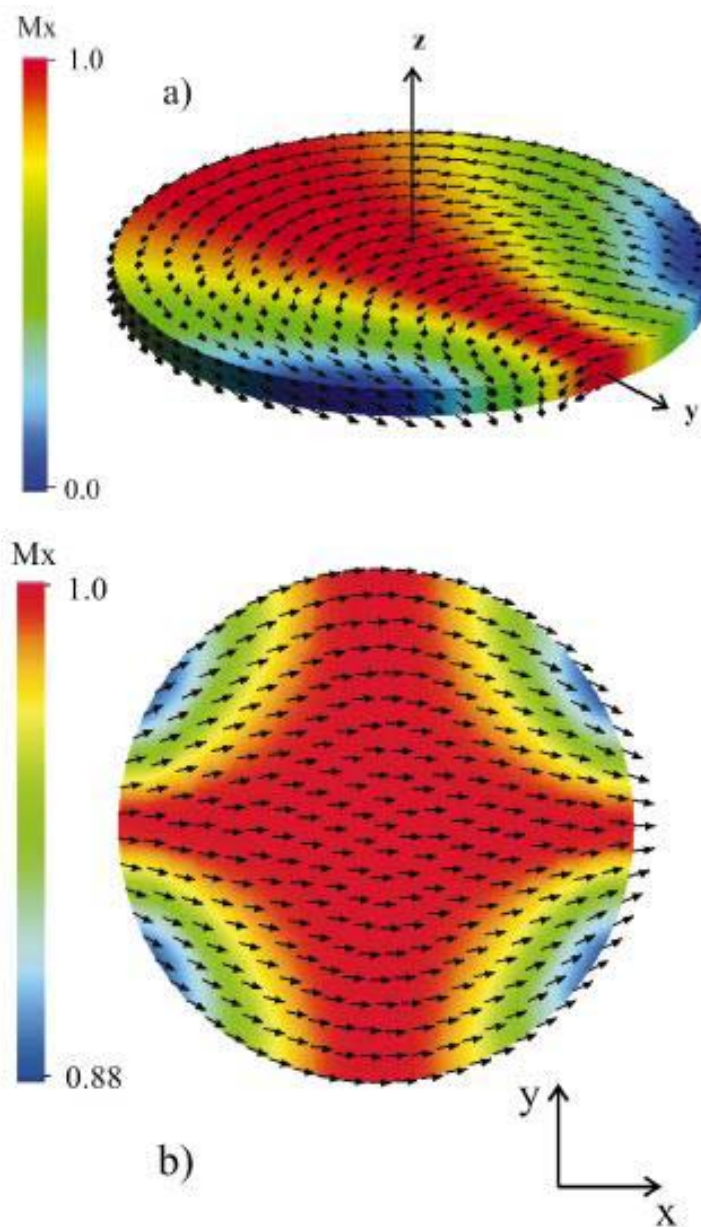
Рис. 1.2. Квазиоднородные состояния намагниченности. (a) – С – состояние, (b) – “onion state” (“луковая рубашка”). Рисунки взяты из работы [44].
