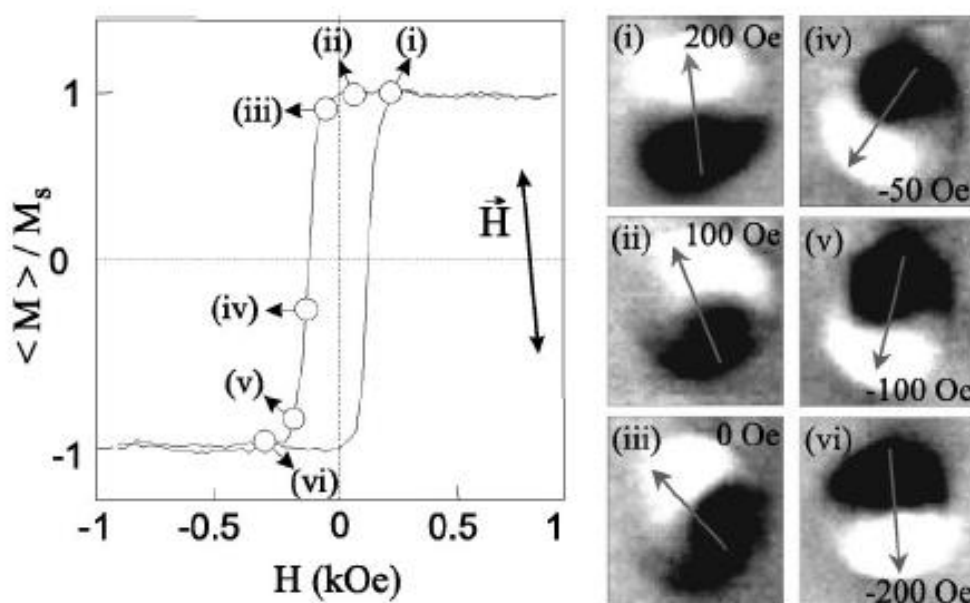
Рис. 1.3. Гистерезисная петля массива ферромагнитных дисков диаметром 500нм и толщиной 10нм. МСМ изображения одного из дисков массива, полученные при различных значениях внешнего магнитного поля.
