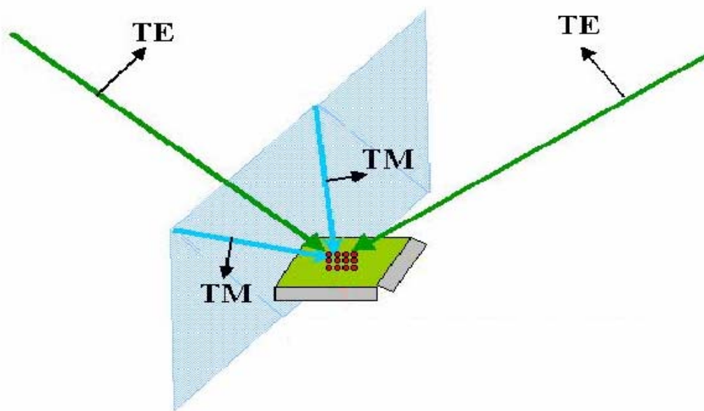
Рис. 2.1. Формирование двумерного упорядоченного массива субмикронных ферромагнитных частиц методом интерференционного лазерного отжига.
