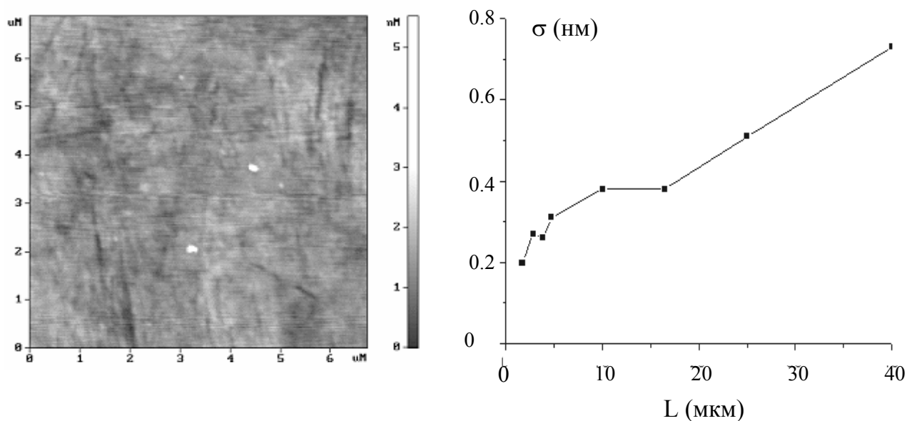
Рис. 3.12. Типичное АСМ изображения поверхности (слева) и зависимость среднеквадратичной шероховатости от размера кадра для подложки №1.
