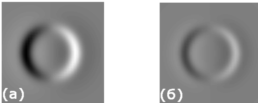
Рис. 5.4. Теоретически рассчитанные МСМ изображения двухслойной частицы Со (а) - направление магнитных моментов в слоях совпадают; (б) – магнитные моменты направлены противоположно. (Диаметр частицы 300 нм, толщина слоев Со 15 нм, толщина прослойки 3 нм, высота прохода МСМ зонда над верхней гранью частицы 50 нм).
