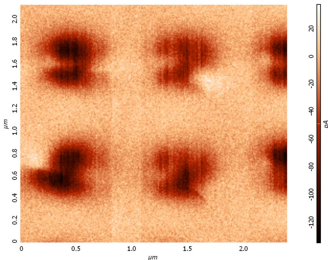
Рис. 5.1. MCM изображение двухслойных ферромагнитных частиц размером 400 \times 250 нм. Толщина каждого Co слоя 15 нм, толщина Si прослойки 2 нм.
