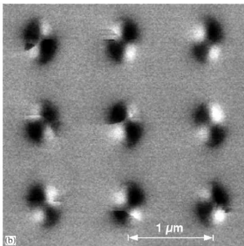
Рис. 1.8. МСМ изображение одновихревых эллиптических частиц. Из работы [55].
