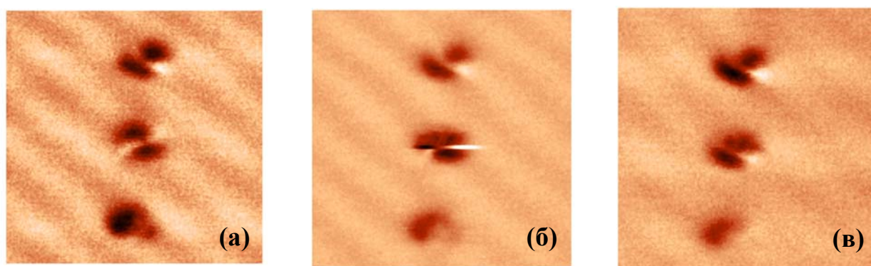
Рис.4.13. МСМ изображения участка массива частиц Со. (а) Исходное состояние. (б) МСМ изображение тех же частиц, полученное в процессе сканировании образца с переменной высотой. (в) Конечное состояние.
