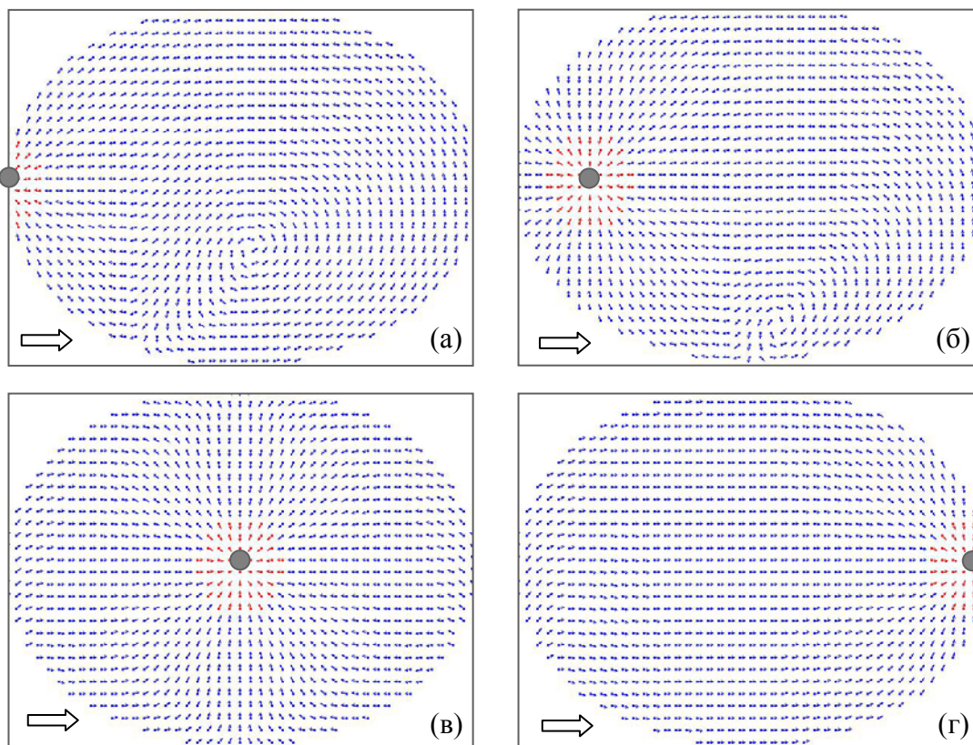
Рис. 4.10. Последовательные стадии процесса перемагничивания частицы S_0 при движении МСМ зонда (зонд показан серым кружком) по центру частицы. Начальное состояние частицы соответствует одновихревому.
