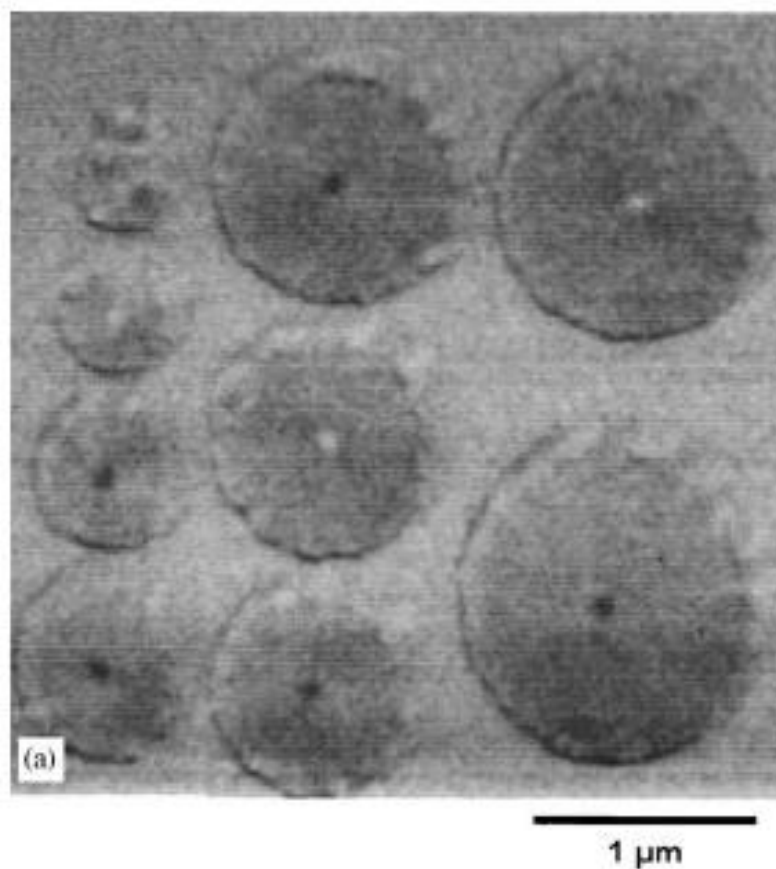
Рис. 1.5. Экспериментальные МСМ изображения вихревых состояний в субмикронных дисках различного размера. Из работы [47].
