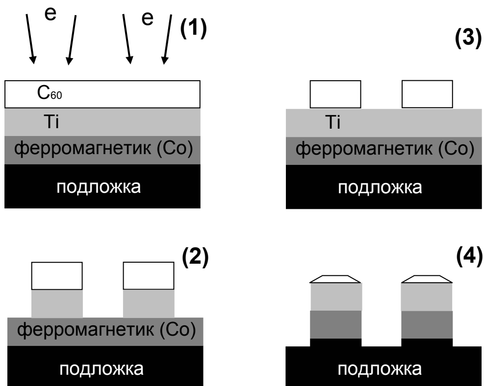
Рис. 2.2. Основные этапы процесса изготовления ферромагнитных частиц при помощи метода электронной литографии. (1) - Нанесение на подложку пленок ферромагнетика (Co), титана (Ti) и пленки фуллерена ( \text{C}_{60} ) с последующей засветкой в электронном микроскопе. (2) - Формирование фуллереновой маски для травления путем обработки СЭМ засвеченной пленки в растворе толуола. (3) - Плазмохимическое травления Ti во фреоне. (4) - Ионное травление Co в атмосфере аргона.
