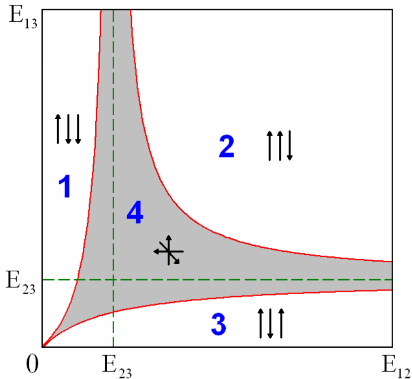
Рис. 5.12. Диаграмма состояний трехслойных субмикронных ферромагнитных дисков.
