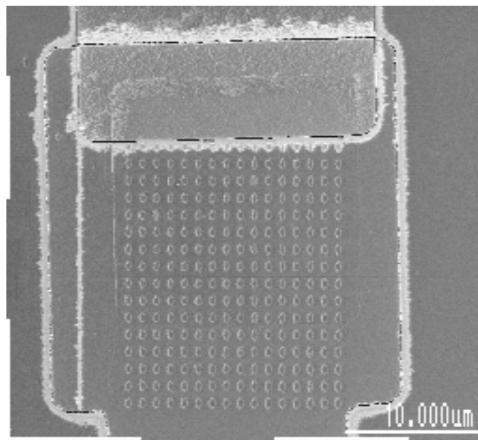
Рис. 4.16. Электронное изображение планарного джозефсоновского контакта с изготовленной на нем прямоугольной решеткой ферромагнитных частиц с размерами 600×400 нм и толщиной 27 нм.
