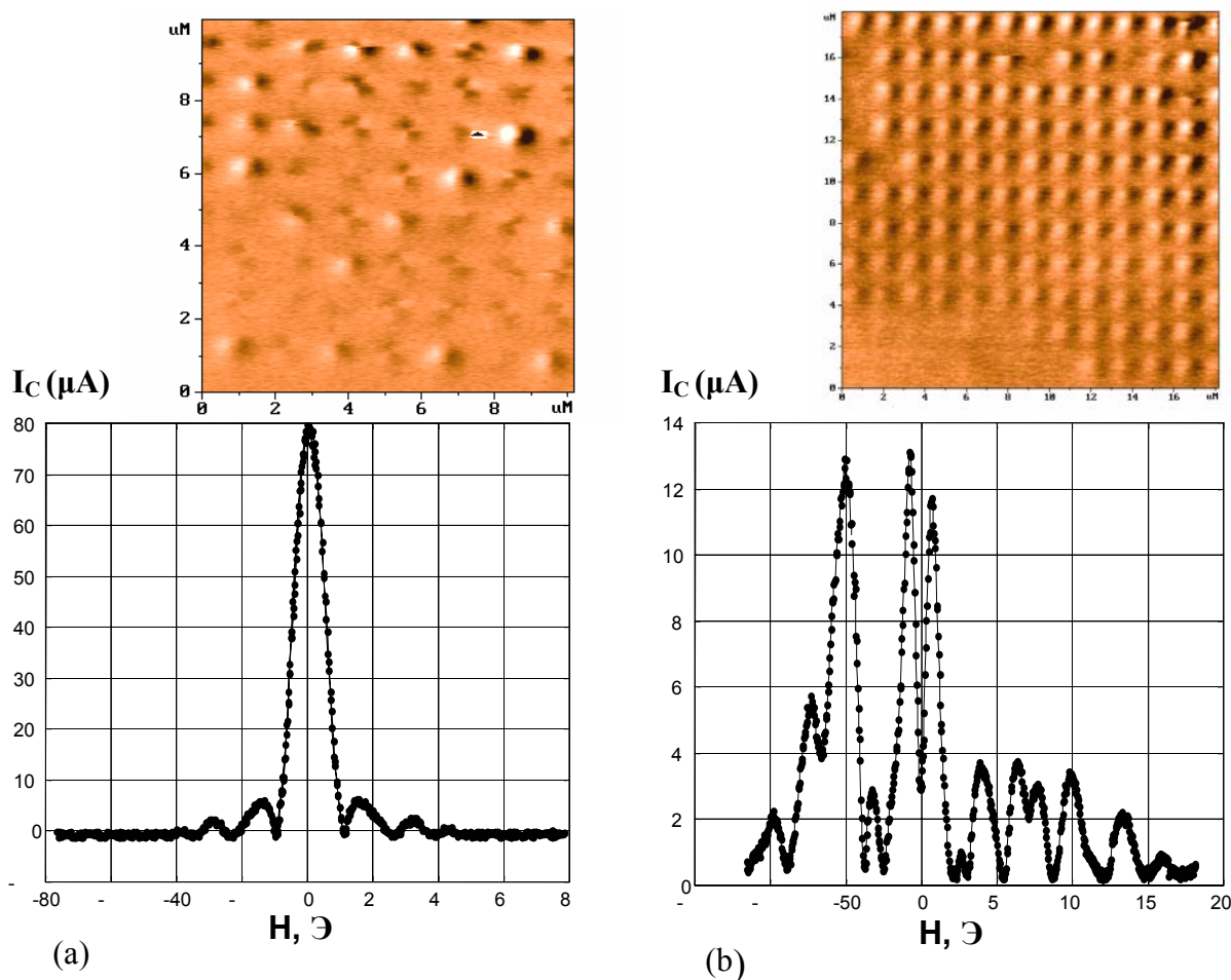
Рис. 4.17. Зависимость критического тока планарного джозефсоновского контакта I_c(H) для двух различных случаев: (а) большинство частиц находится в вихревом состоянии, (б) большинство частиц намагничено однородно. Сверху – MFM изображения состояний намагниченности решетки частиц.
