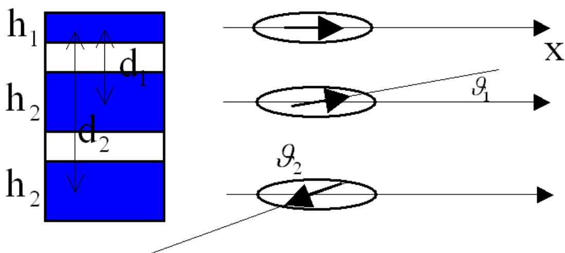
Рис. 5.11. Схематическое изображение трехслойного ферромагнитного диска.
