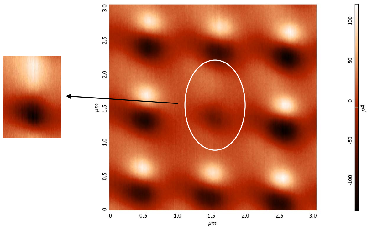
Рис. 5.9. Результат переориентирования \uparrow\downarrow конфигурации при помощи МСМ зонда. На маленьком рисунке слева отдельно показана перемангниченная частица
