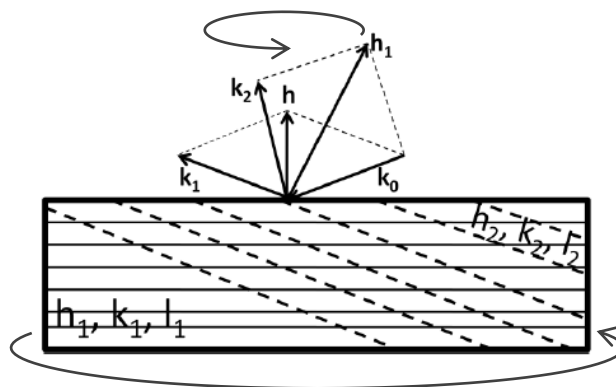
Рис. 2.7. Отражение рентгеновского излучения от двух систем атомных плоскостей (h_1k_1l_1) и (h_2k_2l_2) . k_0, k_1, k_2 – волновые вектора падающего и отраженных излучений соответственно, \mathbf{h} и \mathbf{h}_1 – вектора обратной решетки этих плоскостей. Вращение вектора \mathbf{h}_1 вокруг \mathbf{h} при азимутальном повороте образца.
