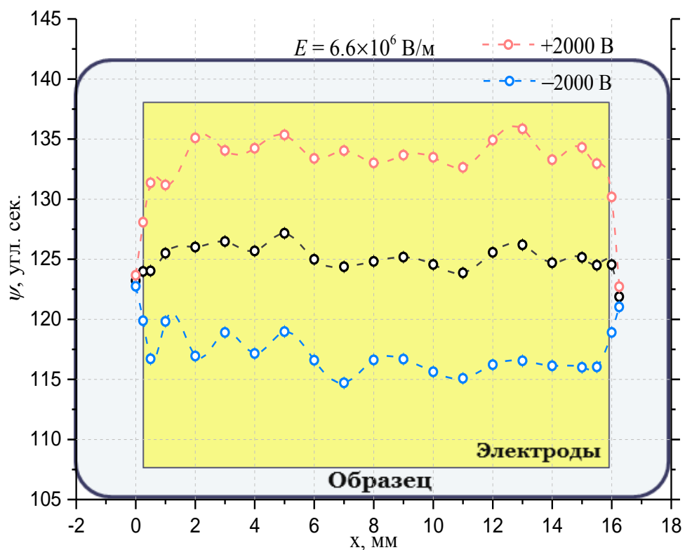
Рис. 2.17. Распределение углового расстояния \psi между пиками КДО рефлексов (770) и (260) кристалла LGT при различных значениях приложенного напряжения.
