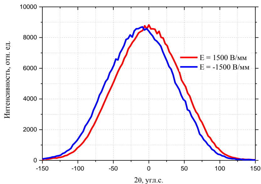
Рис. 2.14. КДО рефлекса (770) кристалла LGT, измеренная методом двухкристальной дифрактометрии при различных значениях напряженности электрического поля, приложенного к образцу.
