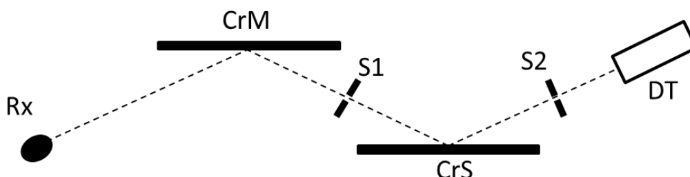
Рис. 3.2. (n, -n)-схема двухкристального дифрактометра для измерения бездисперсионных КДО. Rx – рентгеновская трубка, CrM - кристалл-монохроматор, CrS - кристалл-образец, DT - детектор, S1 и S2 – щели.
