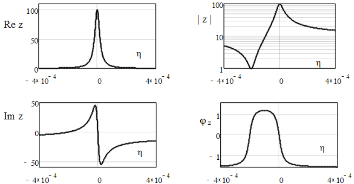
Рис. 1.17. Частотная зависимость нормированного импеданса пьезорезонатора z = Z_1/R . Q = 5 \cdot 10^4 , m = 2 \cdot 10^{-4} .
