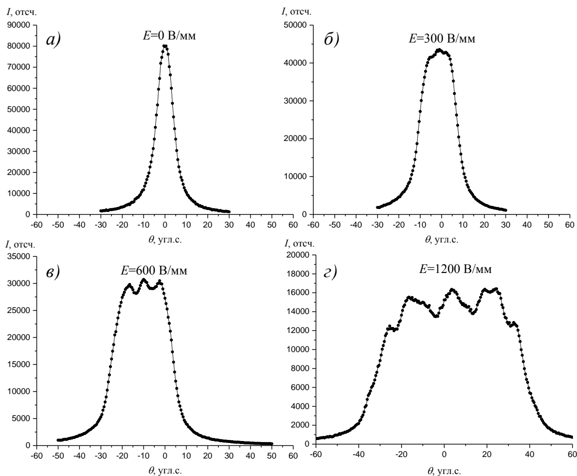
Рис. 3.3. Расщепление КДО рефлекса (220) кристалла \text{TeO}_2 в зависимости от величины напряженности внешнего постоянного ЭП: E = 0 В/мм (а), E = 300 В/мм (б), E = 600 В/мм (в), E = 1200 В/мм (г).
