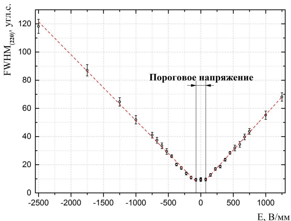
Рис. 3.4. Зависимость полуширины рефлекса (220) кристалла \text{TeO}_2 от величины напряженности приложенного внешнего ЭП (точками обозначены экспериментальные данные, пунктирной линией – линейная аппроксимация).
