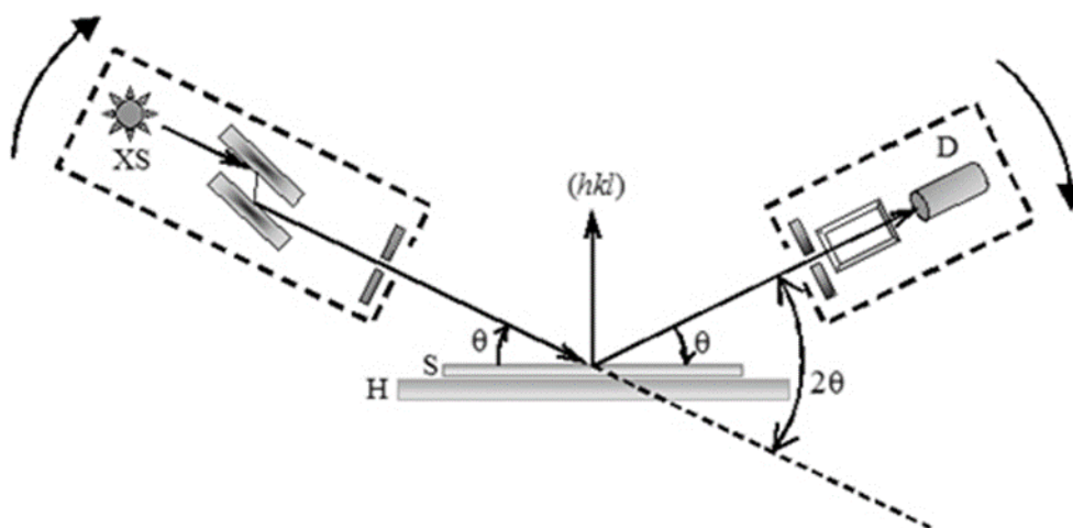
Рис. 2.13. Схема эксперимента по определению пьезомодуля кристалла методом высокоразрешающей дифрактометрии на дифрактометре SmartLab.
