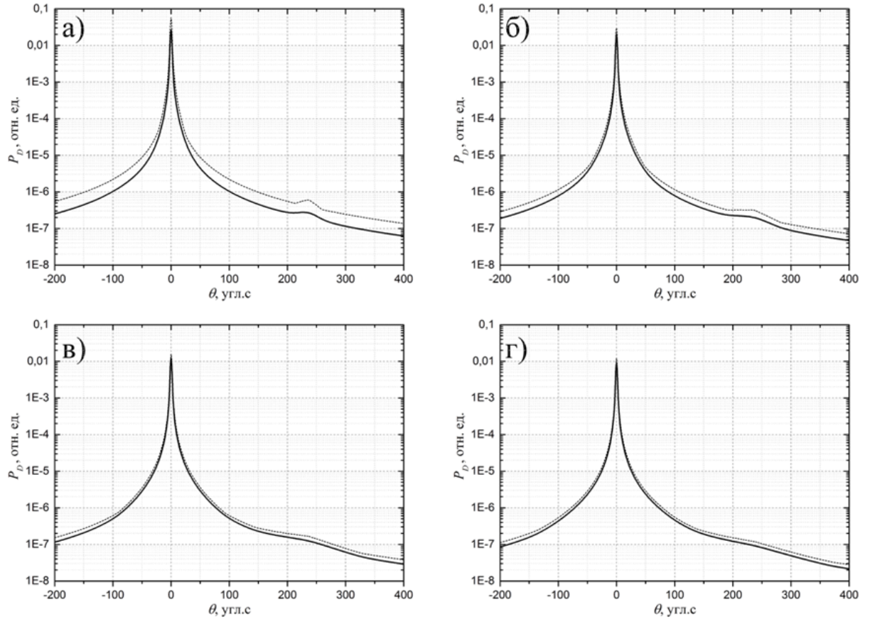
Рис. 4.3. Теоретические КДО, рассчитанные по точной (1) (сплошная линия) и приближенной (4) (пунктирная линия) формулам для различных значений ширины коллимирующих щелей S = S_1 = S_2 : 50 мкм (а), 100 мкм (б), 200 мкм (в), 300 мкм (г).
