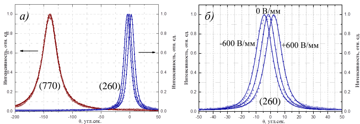
Рис. 2.15. КДО рефлексов (260) и (770) кристалла LGT, находящиеся в условиях квазимноговолновой дифракции и измеренные при различных значениях напряженности электрического поля, приложенного к образцу (а) и увеличенное изображение КДО рефлекса (260) при различных значениях напряженности электрического поля (б).
