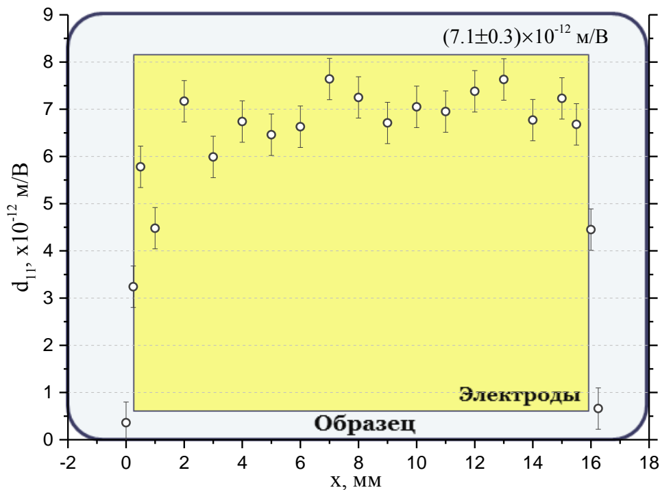
Рис. 2.18. Вариация величины пьезомодуля d_{11} кристалла LGT вдоль поверхности образца, измеренная методом квазимноговолновой дифракции.
