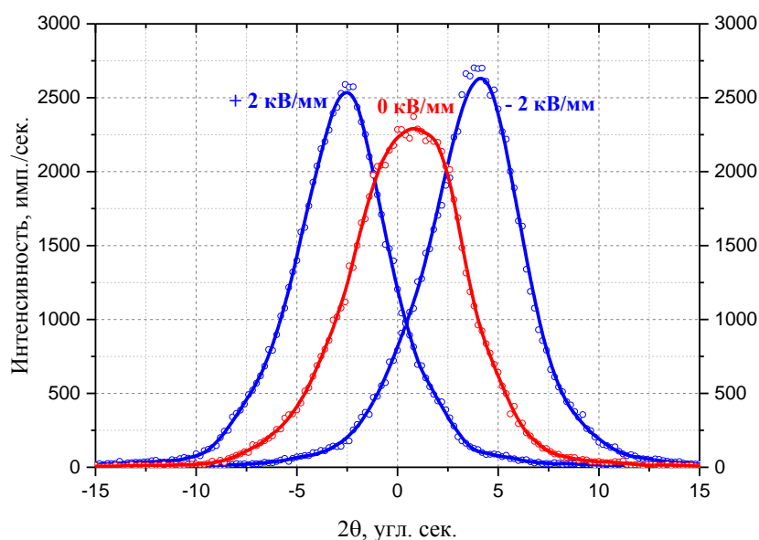
Рис. 2.16. КДО рефлекса (440) кристалла LGT, измеренная методом трехкристальной дифрактометрии (б) при различных значениях напряженности электрического поля, приложенного к образцу. Полуширина КДО, измеренной в трехкристальной схеме, в отсутствие электрического поля 7 угл. с.. при наличии внешнего поля – 5 угл. с.
