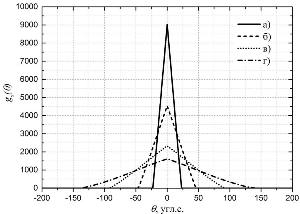
Рис. 4.2. Аппаратная функция углового распределения, рассчитанная по формулам (3) для различных значений ширины коллимирующих щелей S=S_1=S_2 : 50 мкм (а), 100 мкм (б), 200 мкм (в), 300 мкм (г). Оптические расстояния двухкристального дифрактометра l_1 , l_2 и l_{12} равны 0.54, 0.99 и 0.45 м, соответственно.
