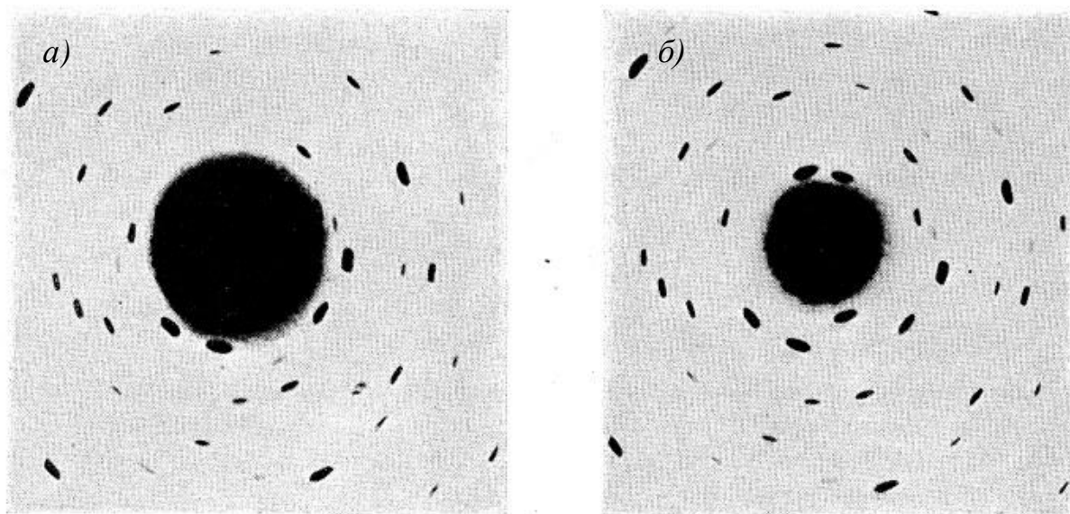
Рис. 1.18. Лауэграммы слюды в отсутствие (а) и при наличии (б) внешнего поля.
