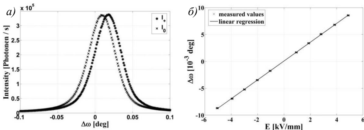
Рис. 1.20. Сдвиг максимума КДО рефлекса (08\bar{7}) кристалла \text{BiV}_3\text{O}_6 вследствие пьезоэлектрической деформации решетки при наложении электрического поля вдоль кристаллографического направления [010] (а) и зависимость углового сдвига пика КДО рефлекса (\bar{7}510) от напряженности приложенного электрического поля (б).
