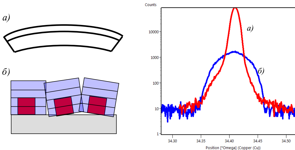
Рис. 3.10. КДО неидеальной кристаллической структуры. Красный пик соответствует разориентированным по углу областям (а), синий – равномерному изгибу (б).
