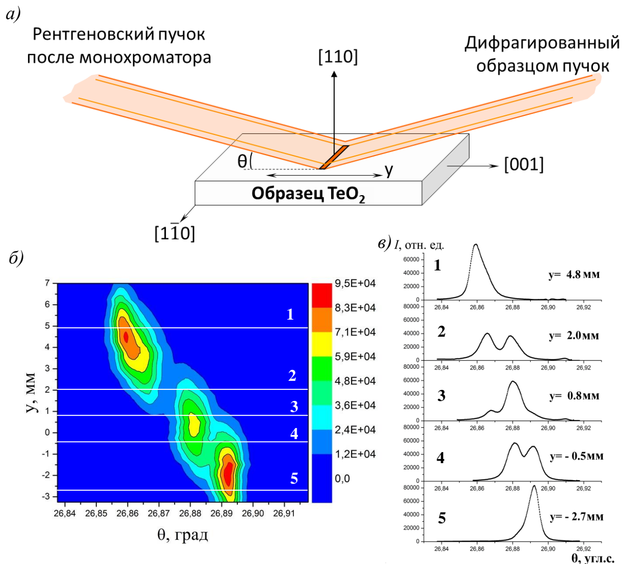
Рис. 3.15. Взаимная разориентация и линейные размеры доменов в кристалле \text{TeO}_2 под действием ЭП ( E = 3750 \text{ В/мм} ): а) – схема сканирования, б) – двумерная картина дифракции в координатах «угол падения излучения ( \theta ) – положение рентгеновского пучка на поверхности образца ( y )», иллюстрирующая пространственную локализацию и изменение формы КДО при смещении пучка по поверхности исследуемого кристалла (цвет отражает интенсивность излучения, дифрагированного образцом), в) – примеры трехкристалльных КДО, измеренных при засветке рентгеновским пучком как областей образца, содержащих отдельные домены (1, 3, 5), так и областей, включающих междоменную границу (2, 4).
