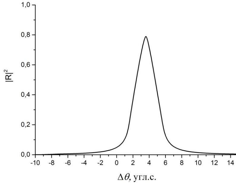
Рис. 1.6. Двухкристальная КДО рассчитанная для параллельной схемы дифракции Si(220)-Si(220).
