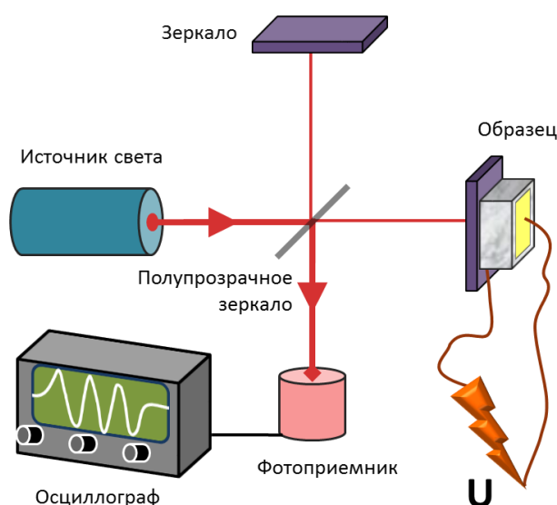
Рис. 1.13. Оптическая схема интерферометра Майкельсона
