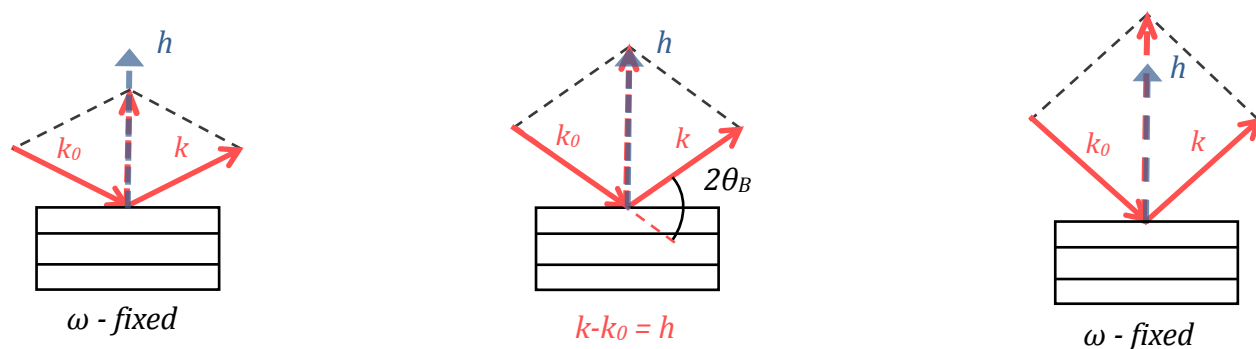
Рис. 3.11. Схема изменения модуля вектора рассеяния при \theta - 2\theta -сканировании.
