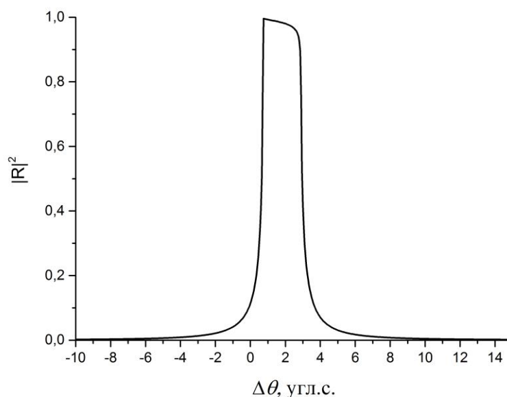
Рис. 1.4. Теоретическая кривая качания, рассчитанная для рефлекса (220) кристалла Si по формулам динамической теории дифракции рентгеновских лучей.
