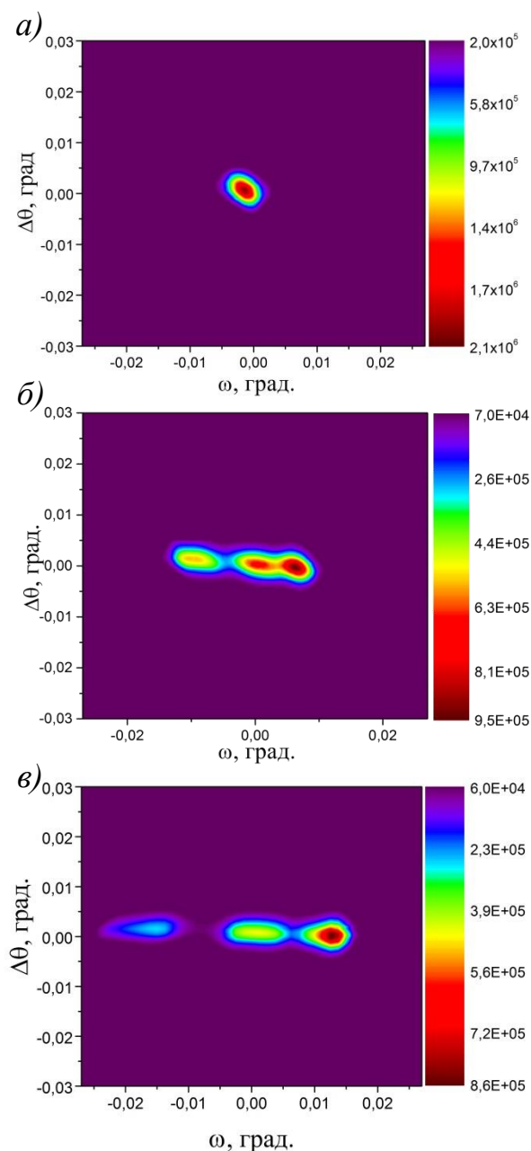
Рис. 3.14. Результаты 2D-картирования рефлекса (220) кристалла \text{TeO}_2 в отсутствие ЭП (а) и при наложении поля -2125 \text{ В/мм} (б), -3750 \text{ В/мм} (в).
