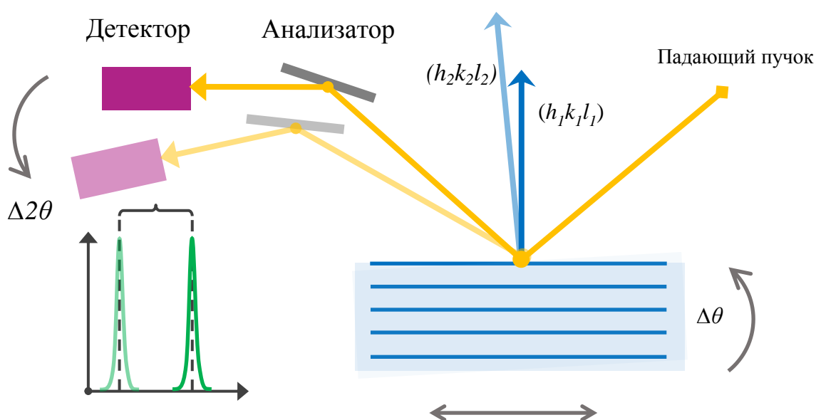
Рис. 2.6. Схема измерения вариации параметра решетки с использованием кристалла-анализатора.
