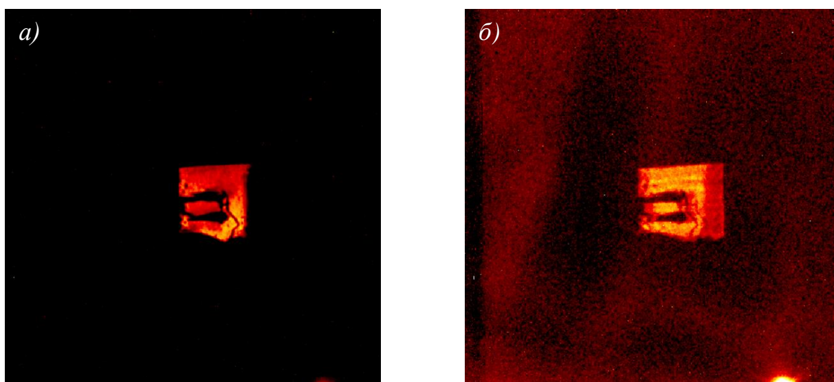
Рис. 3.17. Топограммы кристалла парателлурита измеренные в отсутствие электрического поля в статическом режиме (а) и при наличии поля (2 кВ/мм) в режиме сканирования по углу падения рентгеновского пучка на поверхность образца (б).
