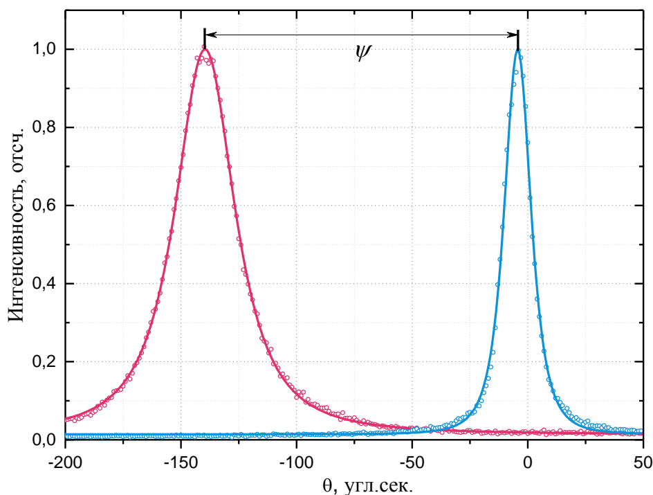
Рис. 2.11. Кривые дифракционного отражения от атомных плоскостей (770) (красный пик) и (260) (синий пик) LGT в условиях квазимноговолновой дифракции.
