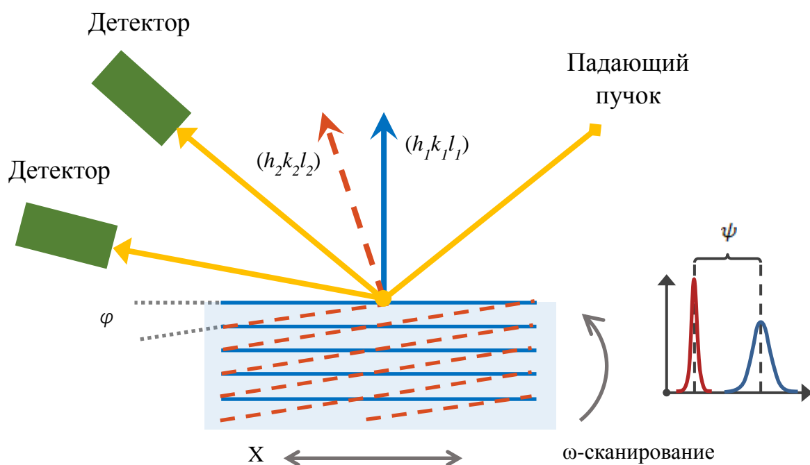
Рис. 2.10. Схема измерения вариации параметра решетки с использованием пары компланарных рефлексов
