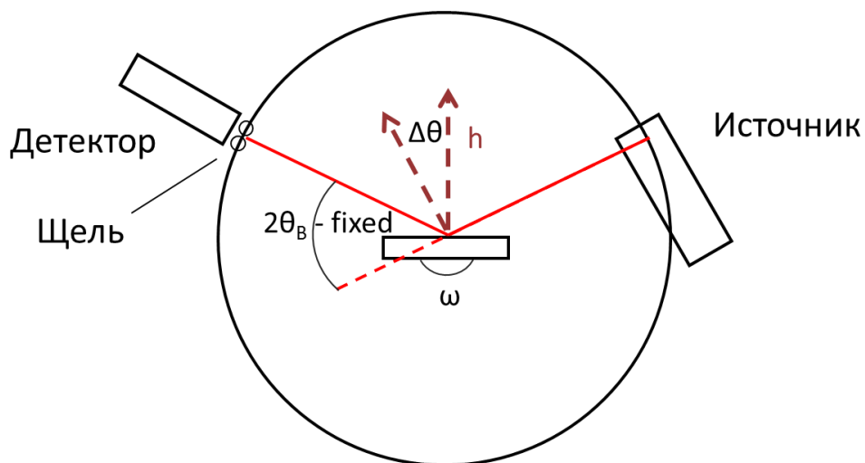
Рис. 3.8. Схема реализации \omega -сканирования.
