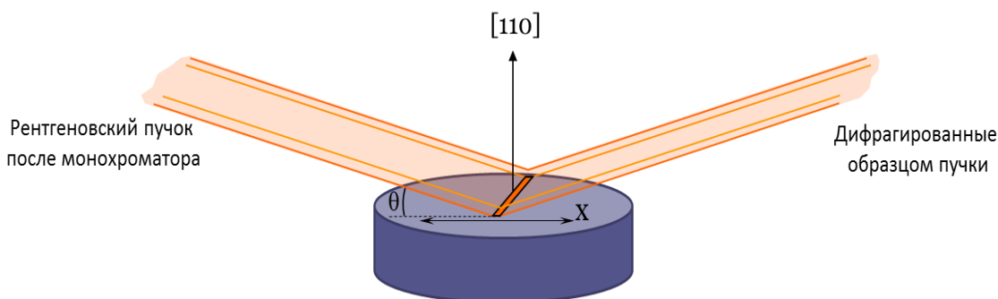
Рис. 4.4. Схема пространственного исследования дефектной структуры кристалла парателлуриита рентгенодифракционными методами.
