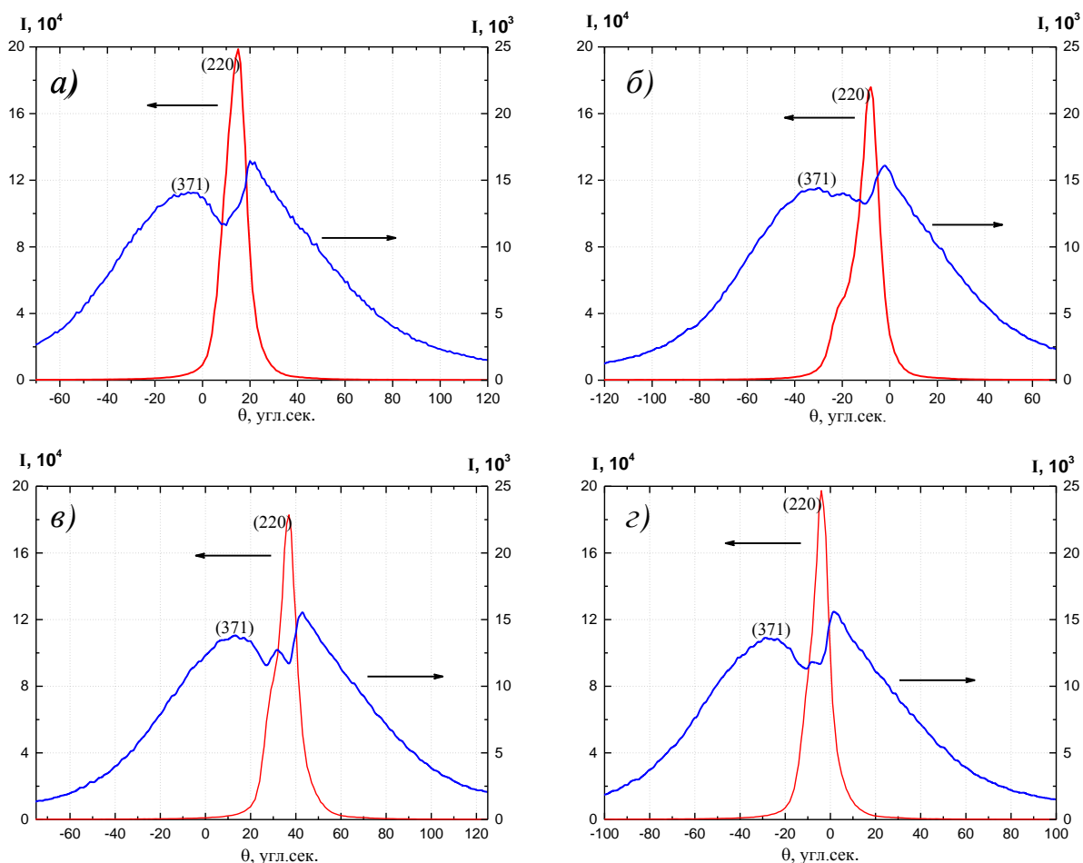
Рис. 4.8. Кривые дифракционного отражения рефлексов (220) и (371), находящиеся в условиях многоволновой дифракции, измеренные в бездефектной (а) и дефектной (б-г) областях поверхности исследуемого образца. На (в) и, особенно, (г) уширения двухволновой кривой отражения (220) уже практически не наблюдается, в то время как многоволновая область отражения (371) отличается от отражения от бездефектной области (а) весьма заметно.
