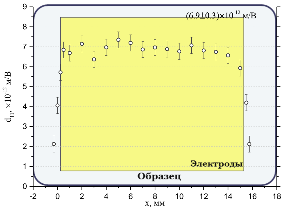
Рис. 2.20. Вариация величины пьезомодуля d_{11} кристалла LGT вдоль поверхности образца, измеренная методом трехкристальной дифрактометрии.
