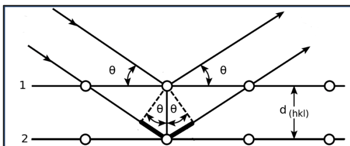
Рис. 1.3. Схема рентгеновской дифракции в брэгговской геометрии.
