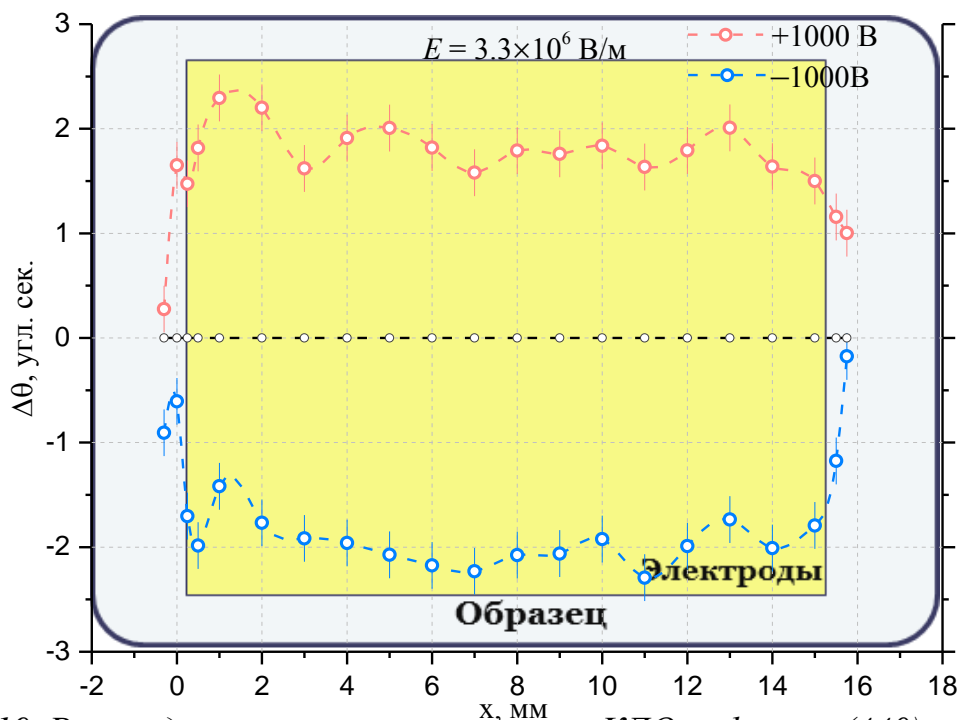
Рис. 2.19. Распределение углового смещения КДО рефлекса (440) кристалла LGT при различных значениях приложенного напряжения.
