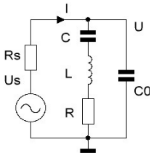
Рис. 1.16. Схема установки для измерения резонансной частоты пьезоэлектрика.
