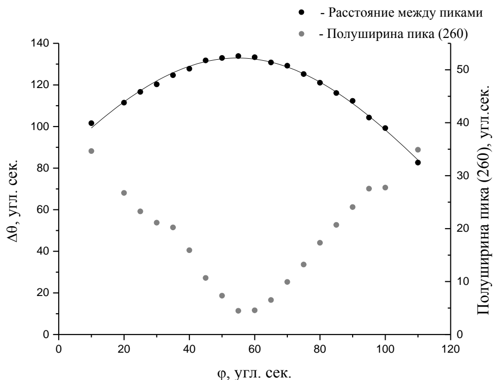
Рисунок 2.9. График зависимости углового расстояния между пиками КДО рефлексов (260) и (770) LGT (1) и полуширины асимметричного рефлекса (2) от азимутального угла.
