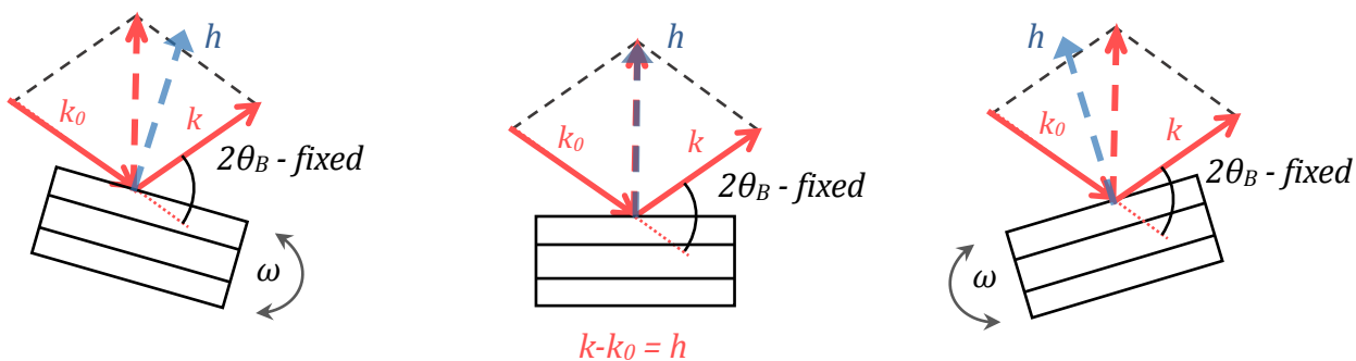
Рис. 3.9. Схема поворота вектора рассеяния при \omega -сканировании.
