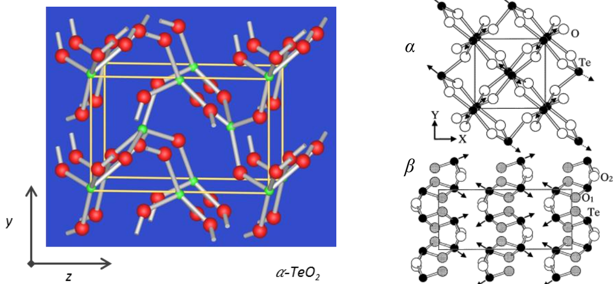
Рис. 3.1. Атомная структура \alpha - \text{TeO}_2 , проекция YZ (слева). Структура \alpha - и \beta - \text{TeO}_2 , проекция XY (справа)
