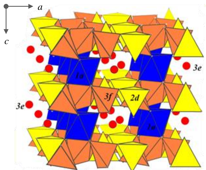
Рис. 2.1. Схема структуры кристаллов семейства лангасита. 3e – La , 1a – Ga , 3f – Ga , 2d – Ga , Si .
