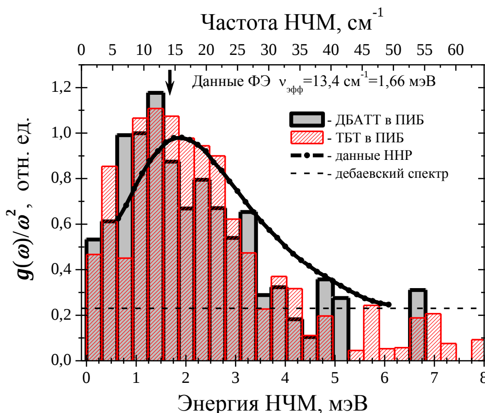
Рис. 6.24. Энергетические спектры НЧМ в аморфном полиизобутилене (420000 г/моль), допированном дибензоантатреном (серая гистограмма, 155 одиночных молекул) и тетра-tert-бутилтерриленом (штрихованная гистограмма, 281 одиночная молекула), измеренные методом СОМ. Сплошная линия - бозонный пик, измеренный в чистом полиизобутилене методом неупругого нейтронного рассеяния [52]. Распределения нормированы на квадрат частоты g(\omega)/\omega^2 для выделения колебательной плотности состояний, превышающей Дебаевский спектр. Кроме того, данные по СОМ были нормированы на Бозе фактор в соответствии с температурными диапазонами измерений. Пунктирной линией показан вклад Дебаевского спектра (звуковых волн) в случае нейтронного рассеяния. Стрелкой показано значение эффективной частоты НЧМ в системе ТБТ/ПИБ, измеренной с помощью метода фотонного эха [A17, A33].
