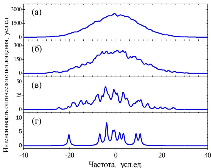
Рис. 2.2. Численное моделирование оптического спектра поглощения образца, содержащего различное число хромофоров: (а) 10000, (б) 1000, (в) 100, (г) 10 молекул. Спектр каждого хромофора смоделирован функцией Лоренца (ширина - 1 усл.ед). Положение центра каждой линии выбрано случайным образом в соответствии с распределением Гаусса (ширина распределения - 20 усл.ед).
