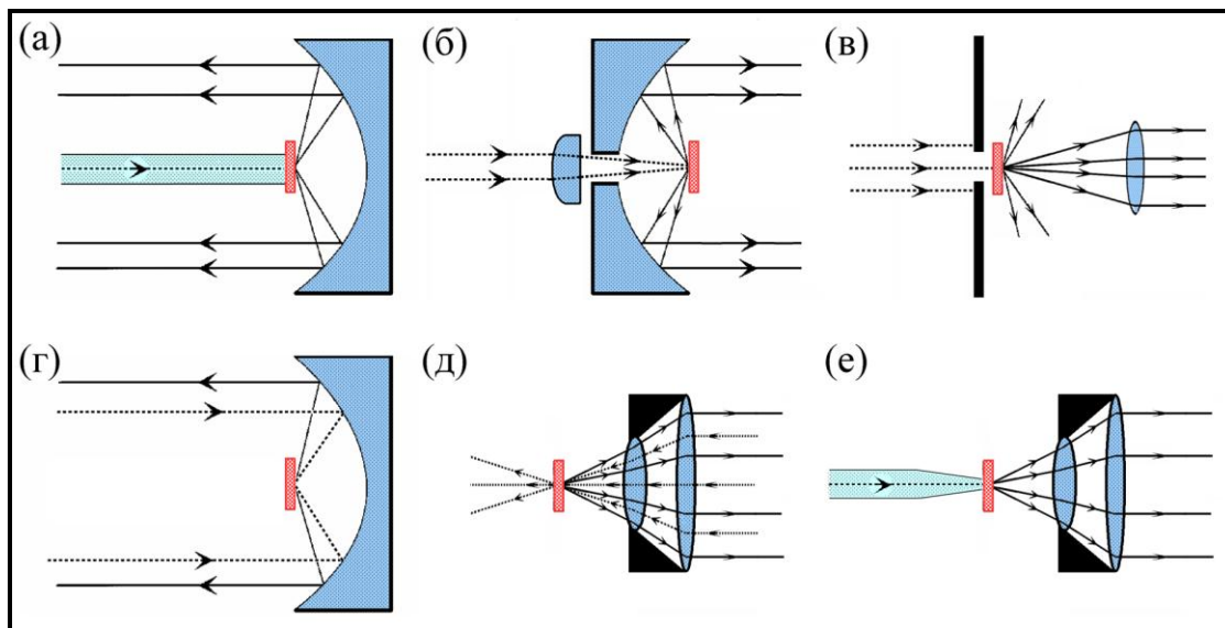
Рис. 2.4. Возможные принципиальные схемы установок для возбуждения спектров одиночных молекул и сбора их флуоресценции. (Взято из [145]) (а) Оптическое волокно + параболическое зеркало. (б) Линза + параболическое зеркало. (в) Малая диафрагма + линза. (г) Конфокальное параболическое зеркало. (д) Конфокальный микрообъектив. (е) Микроскоп ближнего поля с заостренным оптическим волокном.
