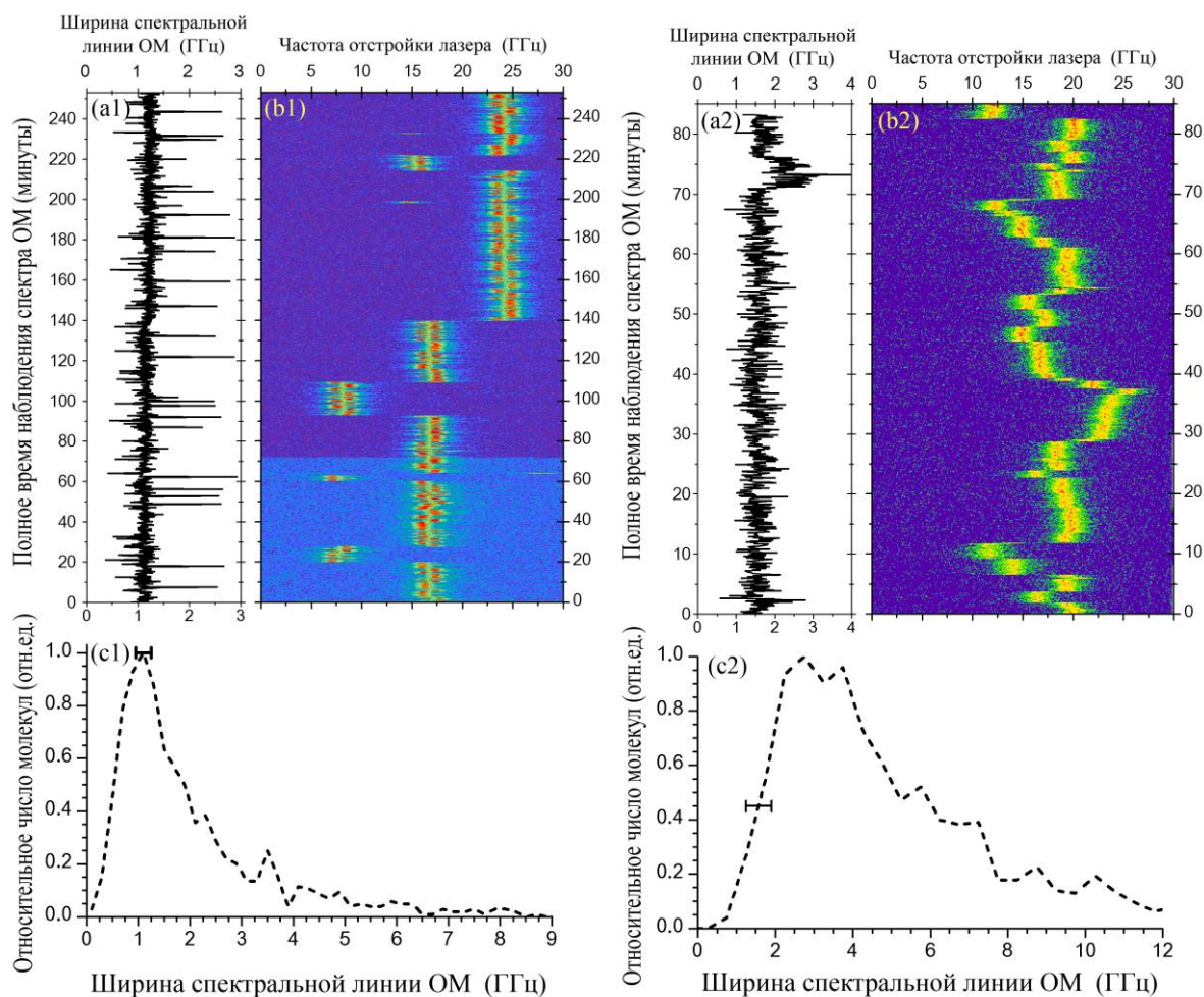
Рис. 5.13. (a1, б1, в1) Спектральная динамика одиночной молекулы ТБТ в ПИБе (420000 г/моль) и (a2, б2, в2) ТБТ в замороженном толуоле при температуре 7К. (a1, a2) Временное поведение ширины спектральной линии ОМ; (б1, б2) Спектральные траектории ОМ, демонстрирующие в случае ПИБ спектральные прыжки, вызванные переходами в ДУС, а в случае замороженного толуола, дополнительные невоспроизводимые случайные прыжки и непрерывные спектральные дрейфы. Количество сканов – 1513 и 996, соответственно. (в1, в2) Распределения ширин спектров ( штриховые линии ) одиночных молекул ТБТ в ПИБ (951 молекула) и в замороженном толуоле (1238 молекул). Короткие отрезки на графиках изображают дисперсию ширины спектра одной и той же ОМ от скана к скану.
