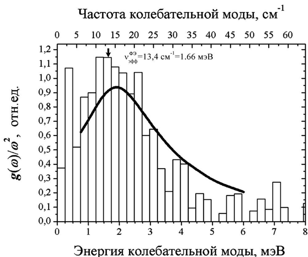
Рис. 6.12. Энергетический спектр НЧМ в аморфном ПИБе (420000 г/моль), допированном молекулами ТБТ, измеренный методом СОМ ( гистограмма ) и бозонный пик в чистом ПИБе, измеренный методом неупругого нейтронного рассеяния ( сплошная линия ) [52]. Для выделения вклада возбуждений, приводящих к возрастанию ПКС над Дебаевским спектром, распределения приведены в виде зависимости g(\omega)/\omega^2 от частоты \omega , где g(\omega) - ПКС. Данные по СОМ нормированы на Бозе фактор в соответствии с температурным диапазоном измерений. Стрелкой отмечена эффективная частота НЧМ, измеренная методом ФЭ [A17, A33].
