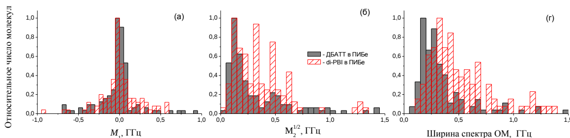
Рис. 6.21. Распределение моментов и ширин линий спектров одиночных димеров di-PBI и одиночных молекул ДБАТТ в аморфном ПИБе ( M_w = 420000 г/моль). T=1,5 К, время измерения 120 с, di-PBI (штрихованная гистограмма, 110 молекул), ДБАТТ (серая гистограмма, 135 молекул).
