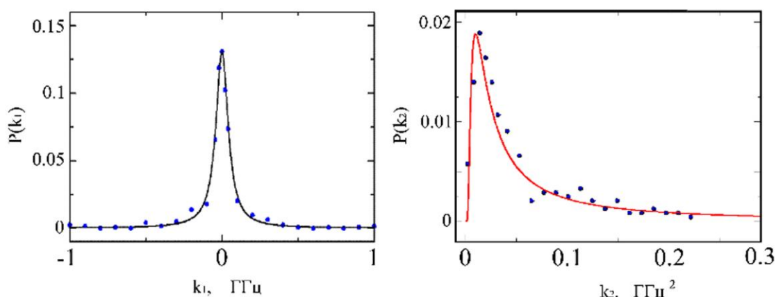
Рис. 6.9. Измеренные распределения первых и вторых кумулянтов и их аппроксимация в рамках статистики Лёви. Точки – распределения, полученные на основе измеренных спектров одиночных молекул ( тетра-tert-бутилтеррилена в полиизобутилене (температура 2 К, время измерения 120 с), сплошные линии - аппроксимация функциями Лоренца и Смирнова (сплошные кривые), соответственно.
