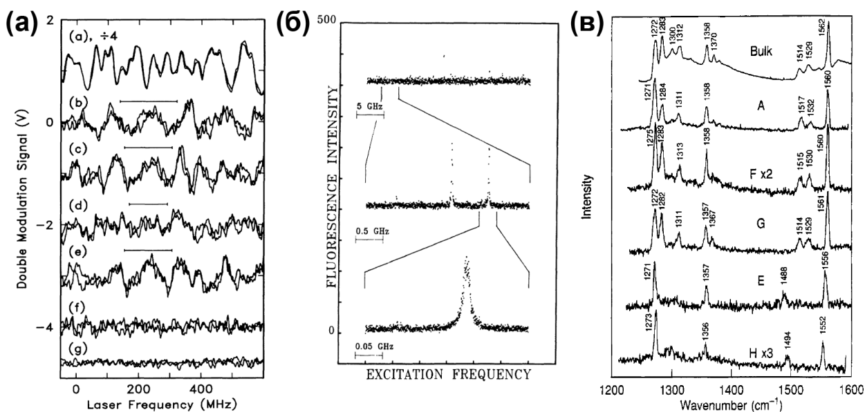
Рис. 2.3. Примеры спектров поглощения (а), возбуждения флуоресценции (б) и флуоресценции (в) одиночных молекул в твердотельных матрицах, взятые из пионерских работ, посвященных развитию методов [14, 15, 155].
