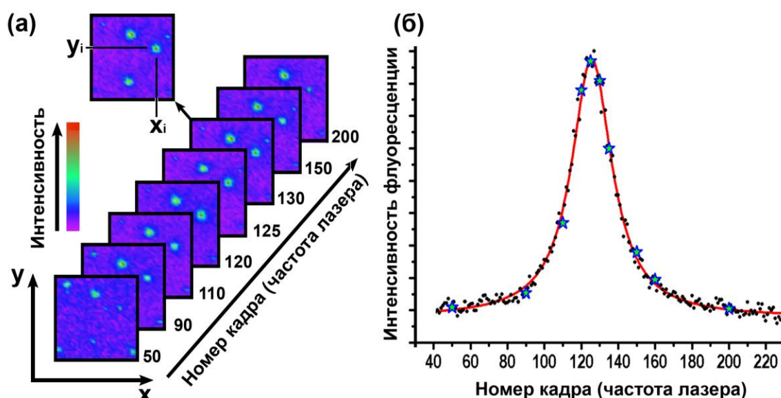
Рис. 4.1. Иллюстрация к процедуре извлечения спектра ОМ из последовательности видеокадров. (а) Идентификация люминесцентных изображений одной и той же одиночной молекулы при сканировании частоты лазера. (б) Спектр возбуждения флуоресценции выбранной i -ой молекулы с координатами x_i, y_i (точки) и его аппроксимация функцией Лоренца (сплошная линия). Звездочки соответствуют видеокадрам, изображенным на рисунке (а).
