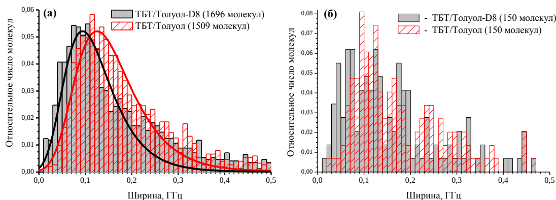
Рис. 4.4. Иллюстрация к вопросу о статистической достоверности при измерениях спектров ОМ. Распределения ширин спектров одиночных молекул в толуоле и дейтерированном толуоле для различного числа молекул ( T=2\text{K} ). Изотопический эффект четко заметен только в случае большого ( \sim 2000 ) числа измеренных спектров.
