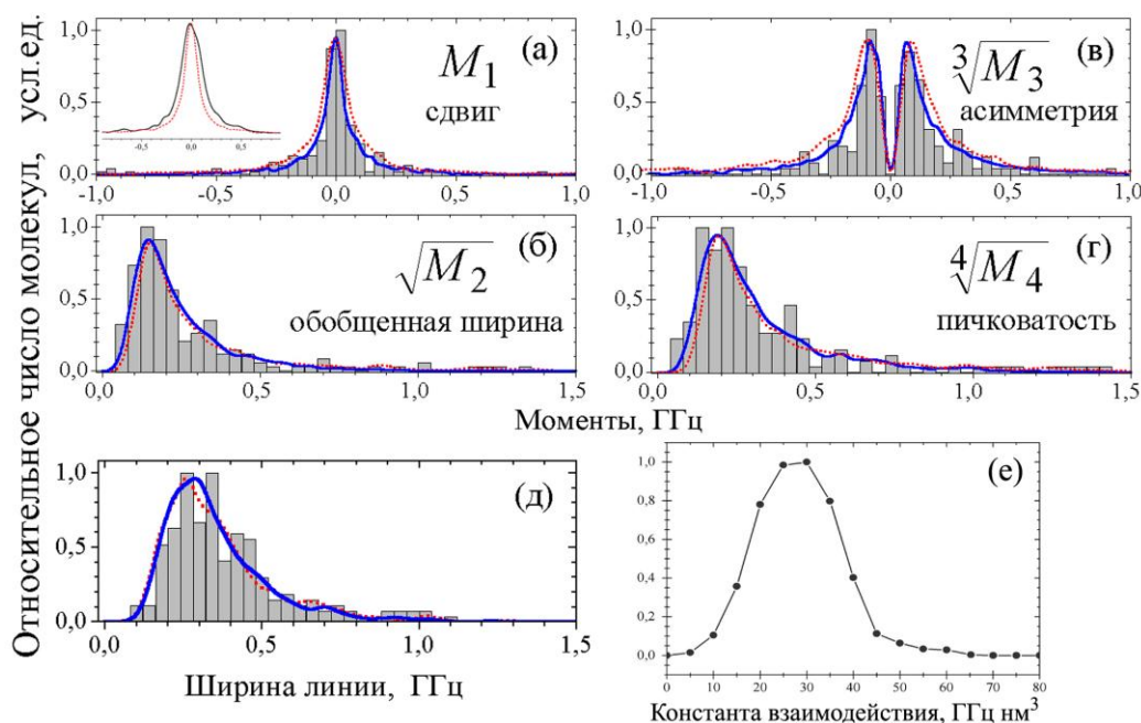
Рис. 6.5. Распределения первых четырех моментов (а-г) и ширины линий (д), полученные на основе \sim 2000 моделированных (сплошные и пунктирные линии) и 244 измеренных (гистограммы) одиночных молекул ТБТ в ПИБ. Точечные линии показывают расчетные распределения без учета минимального радиуса взаимодействия примесь-ДУС. Распределения, изображенные сплошными линиями соответствуют значению r_{\min} = 2,5 нм. Вставка на рисунке (а): распределения первого момента (сдвиг), рассчитанные для двух различных значений начальной частоты: начальная частота установлена к значению \omega_0 = 0 , соответствующему состоянию, когда все ДУС находятся в основном состоянии (сплошная линия), начальная частота равна частоте \omega_{\max} = 0 , соответствующей максимуму флуоресценции (пунктирная линия). (е) Распределение значений константы взаимодействия ДУС-хромофор, A , соответствующее наилучшему согласию экспериментальных и расчетных данных СОМ для системы ТБТ/ПИБ.
