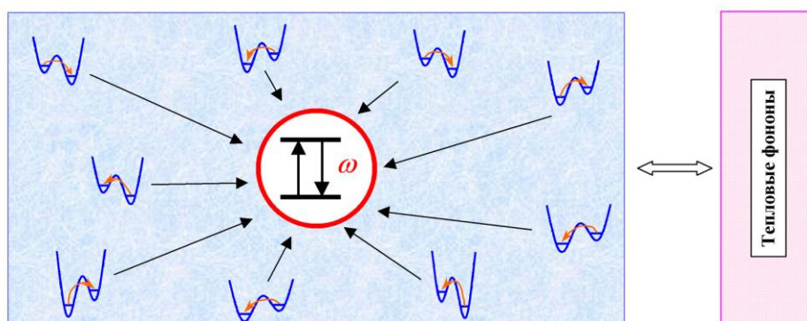
Рис. 1.11. Взаимодействие ДУС с примесным центром (схема).
