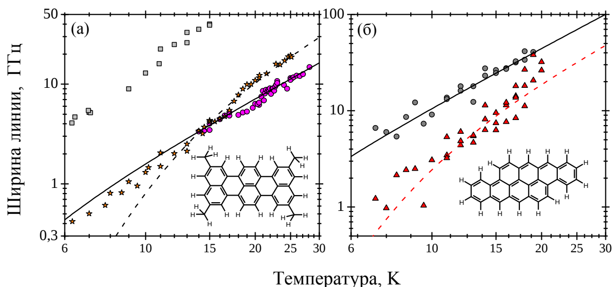
Рис. 6.23. Примеры температурных зависимостей спектральных ширин ОМ для трех молекул тетра-tert-бутилтеррилена (а) и двух молекул дибензоантатрена (б) в аморфном полиизобутилене (420000 г/моль). Линии – графики аппроксимирующих функций (уравнение (1.17)).
