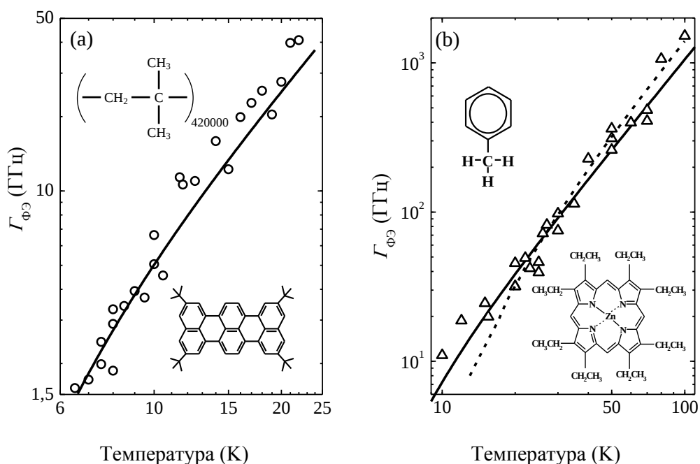
Рис. 6.14. Температурные зависимости обратного времени оптической дефазировки, измеренные методом ФЭ для (а) ПИБа, допированного молекулами ТБТ – кружки и (б) толуола, допированного молекулами ZnОЕР – треугольники . Сплошные линии – результат аппроксимации измеренных зависимостей с использованием формулы (6.12). Штриховая линия на (б) – результат аппроксимации с использованием данных о бозонном пике, измеренном методом КРС в [46] (см. подробнее [A25, A28]).
