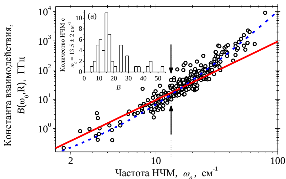
Рис. 6.16. Зависимость константы квадратичного взаимодействия ОМ-НЧМ (в приближении слабой связи) от частоты НЧМ (кружки) для аморфного ПИБа (420000 г/моль), допированного молекулами ТБТ. Штриховая линия изображает наилучшую аппроксимацию данных полиномиальной функцией. Сплошная линия представляет наилучшую аппроксимацию квадратичной зависимостью B = a\omega_0^2 . Стрелки изображают область возможных значений B при частоте НЧМ \omega_{\text{БП}} \approx 13,5 \text{ см}^{-1} вблизи максимума бозонного пика. При выбранной частоте значения B имеют значительное распределение (в частности, из-за различия расстояния и взаимной ориентации между ОМ и НЧМ). Гистограмма на вставке (а) изображает распределение значений B в узком диапазоне частот НЧМ \Delta\omega_0 = \omega_{\text{БП}} \pm 2 \text{ см}^{-1} вблизи максимума бозонного пика.
