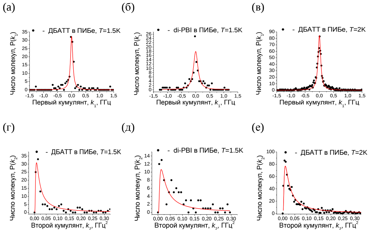
Рис. 6.22. Распределение первых двух кумулянтов спектров ОМ ( точки ) и их аппроксимации функциями Лоренца и Смирнова, соответственно ( линии ), для ДБАТТ/ПИБ при T = 1,5 К (а, г), di-PBI/ПИБ при T = 1,5 К (б, д) и ДБАТТ/ПИБ при T = 2 К (в, е).
