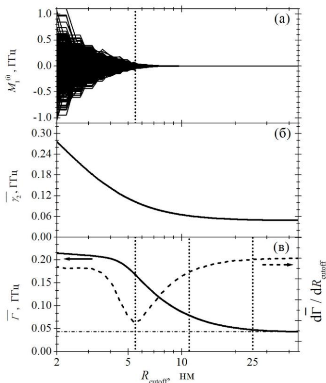
Рис. 6.7. Определение характерных зон взаимодействия ДУС с хромофором. Зависимости первых моментов M_1^{(i)} (а); среднего значения вторых моментов \bar{\gamma}_2 (б); среднего значения ширины спектральных пиков \bar{\Gamma} (в) спектров одиночных молекул от величины минимального радиуса R_{\text{cutoff}} , ограничивающего объем, содержащий двухуровневые системы матрицы, взаимодействие с которыми учитывается при расчете спектров ОМ. Ширина спектрального пика в спектре ОМ определяется на высоте I_{\text{max}}/e . Расчеты проведены для системы ТБТ в ПИБе (температура 2 К, время измерения 120 с). Штриховая линия на (в) представляет первую производную d\bar{\Gamma}(R_{\text{cutoff}})/dR_{\text{cutoff}} , по которой определяется точка перегиба кривой \bar{\Gamma}(R_{\text{cutoff}}) . Вертикальные пунктирные линии демонстрируют положение границ между характерными зонами взаимодействия ДУС с хромофорами. Горизонтальная штрихпунктирная линия на (в) соответствует естественной ширине спектральной линии, определяемой временем T_1 .
