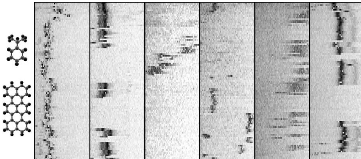
Рис. 5.15. Примеры спектральных траекторий для одиночных молекул ТБТ в замороженном изопропилбензоле. T=4,5\text{K} , диапазон сканирования составляет 30 ГГц, число спектральных точек на скан – 1000, время на одну спектральную точку – 20 мс, количество сканов в спектральных траекторий – 100.
