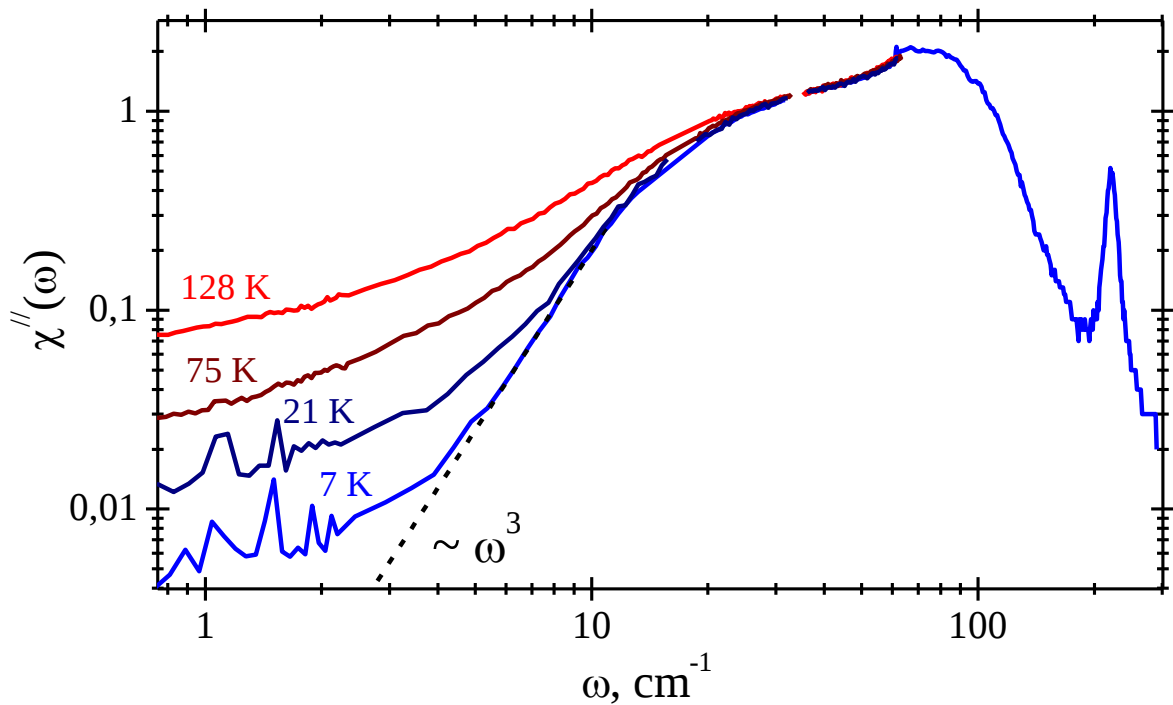
Рис. 1.4. Спектры релаксационной восприимчивости для замороженного толуола при различных температурах, измеренные методом низкочастотного комбинационного рассеяния света [46]. Штрихованная линия показывает экстраполяцию колебательного вклада \omega^3 .
