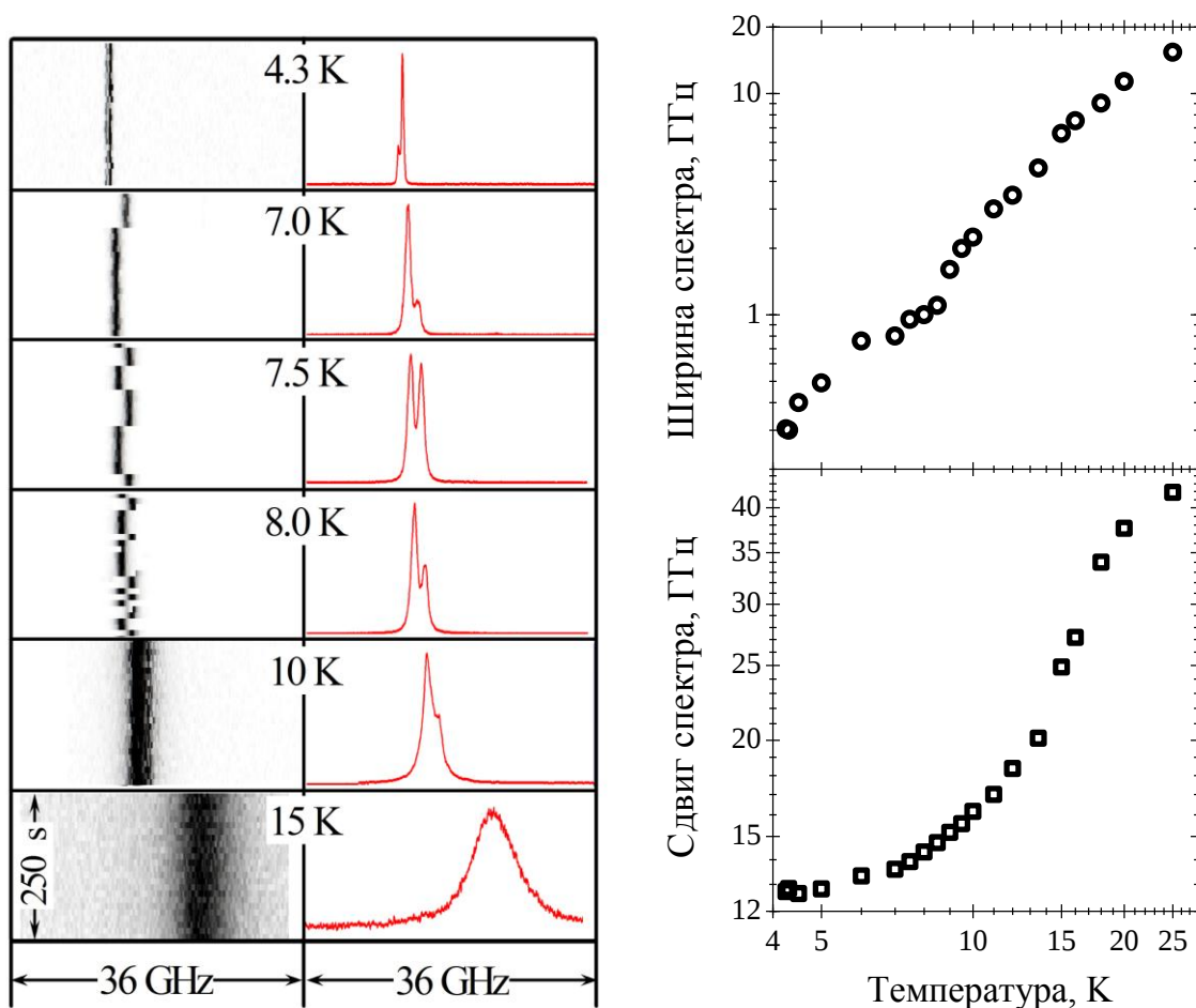
Рис. 5.2. Температурная зависимость формы и временного поведения спектра одиночной молекулы. (а) Спектральные траектории (слева) и соответствующие суммарные спектры (справа) одной и той же одиночной молекулы тетра-tert-бутилтеррилена в аморфном полиизобутилене ( M_w=420000 г/моль) при различных температурах ( t_{\text{scan}}=10 сек). (б) Температурные зависимости ширины (вверху) и сдвига (внизу) спектра ОМ.
