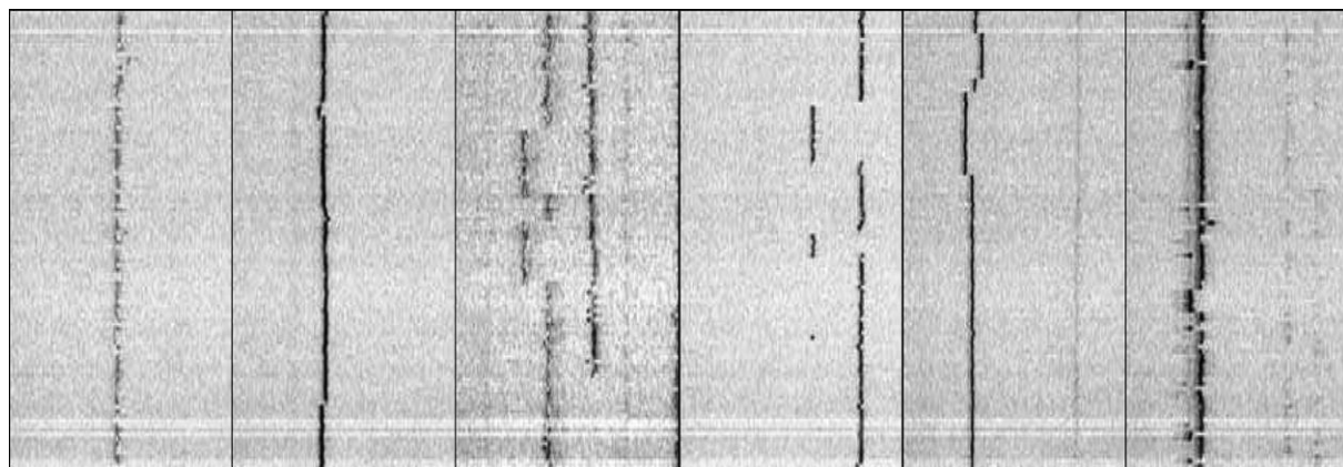
Рис. 5.20. Примеры спектральных траекторий ОМ для ТБТ в ПИБе с молекулярным весом M_w=420000 г/моль. T=4,5\text{K} , диапазон сканирования составляет 30 ГГц, число спектральных точек на скан – 1000, время на одну спектральную точку – 40 мс, количество сканов в спектральных траекторий – 100.
