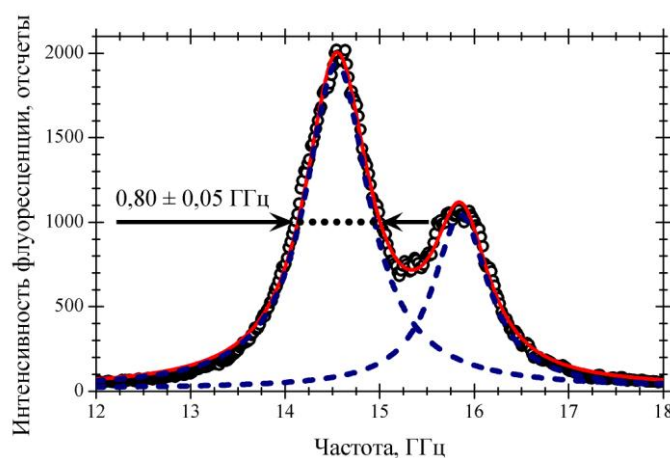
Рис. 3.3. Определение ширины в спектре одиночной молекулы, состоящем из двух перекрывающихся пиков ( кружки ). Система – ТБТ/ПИБ, время измерения спектра 120с, T=8\text{K} . Для определения ширины спектр аппроксимирован суммой двух Лоренцианов ( штриховые линии ). Итоговый аппроксимирующий контур изображен сплошной линией .
