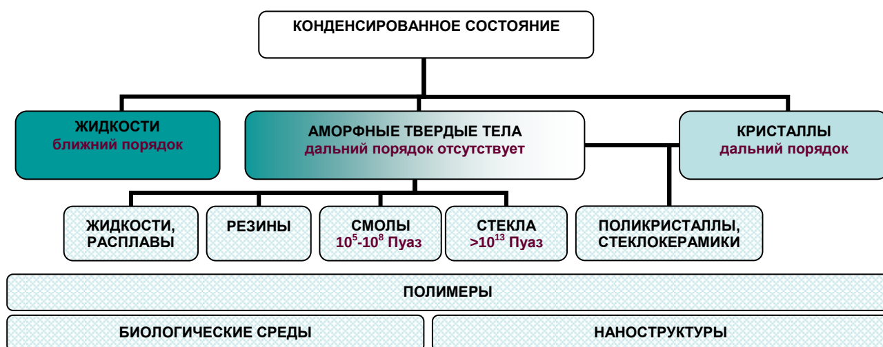
Рис. 1.2. Неупорядоченные твердотельные среды на диаграмме состояний вещества.
