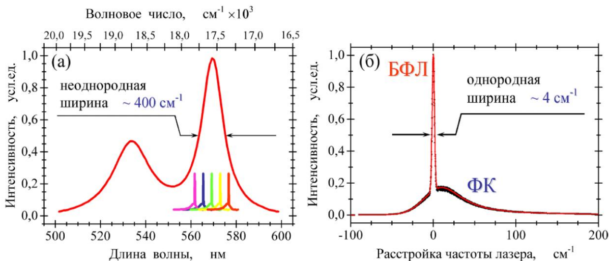
Рис. 1.7. (а) Неоднородно уширенный спектр поглощения ZnOЭП в толуоле при комнатной температуре. (б) Селективно возбуждаемый лазерным источником «однородный» спектр люминесценции MgOЭП в полистироле при температуре 20 К. Взято из [62].
