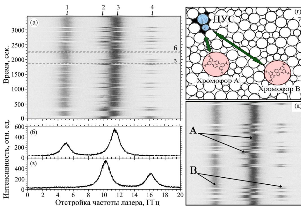
Рис. 5.10. Взаимодействие двух одиночных молекул с одной ДУС. (а) Пример спектральных траекторий, измеренных для ТБТ/ПИБ (420000 г/моль) при T = 7 К. (б,в) Интегральные спектральные контуры за временные интервалы 60 с, изображенные на (а) горизонтальными штриховыми линиями. (г,д) Четко согласованные прыжки четырех спектральных пиков могут быть вызваны взаимодействием двух примесных молекул А и В с одной и той же «сильно взаимодействующей» ДУС.
