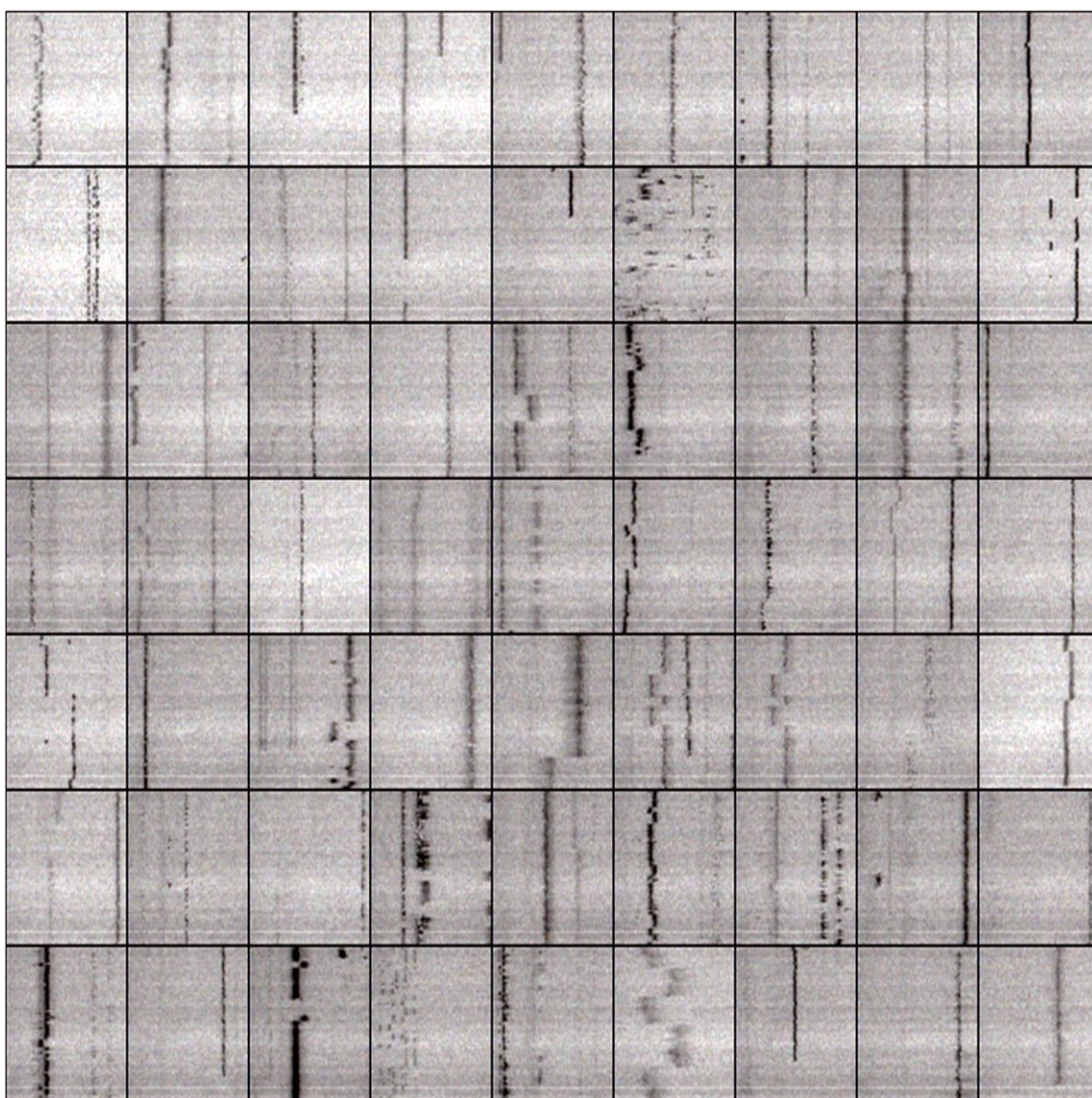
Рис. 4.3. Примеры спектральных траекторий множества одиночных молекул, зарегистрированных с использованием новой техники (образец – ТБТ/ПИБ, T=4,5\text{K} , диапазон сканирования частоты лазера 30 ГГц, количество точек в скане - 1000, время на точку - 40 мс, количество сканов - 100).
