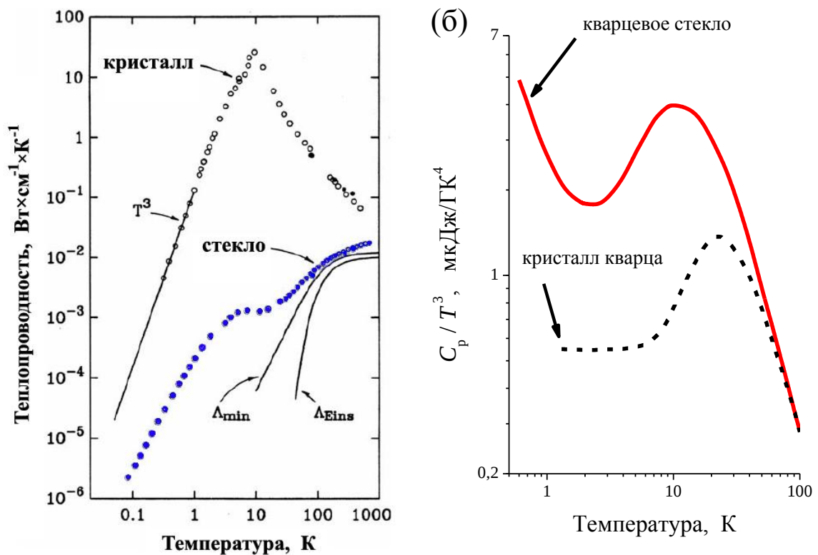
Рис. 1.3. Характерные температурные зависимости теплопроводности и теплоемкости в кристаллах и стеклах. (а) Характерные отличия теплопроводности твердотельной среды (здесь \text{SiO}_2 ) в кристаллическом (верхняя кривая) и аморфном (нижняя кривая) состояниях. Взято с изменениями из [34]. (б) Характерные отличия теплоемкости твердотельной среды в кристаллическом (пунктирная линия) [35] и аморфном (сплошная линия) [1] состояниях. Взято с изменениями из [36].
