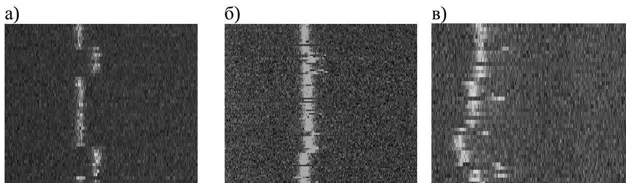
Рис. 6.19. Примеры спектральных траекторий одиночных хромофорных молекул ТБТ (а), ДБАТТ (б) и молекулярного комплекса di-PBI (в) в аморфном полиизобутилене. Измерения проведены при температурах T = 1,5 К и 2 К. Спектральный диапазон составляет 10 ГГц, число спектральных точек на скан – 1000, количество сканов варьируется от 50 до 100. Соответствующие суммарные (по всем сканам) спектры приведены внизу 2D графиков.
