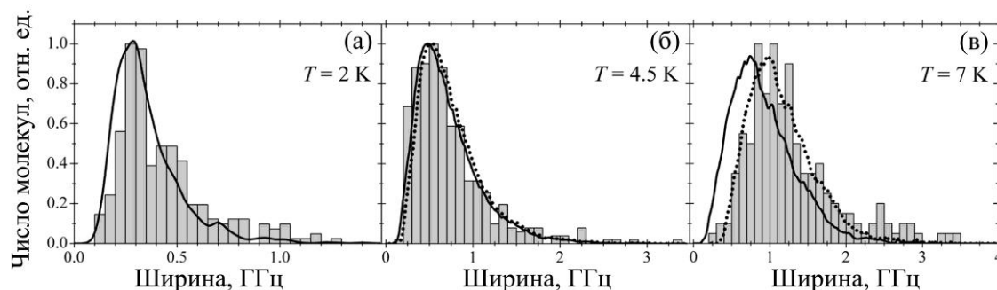
Рис. 6.11. Распределения ширин спектров ОМ при различных температурах. Сплошные и пунктирные линии – результат расчетов, гистограммы – экспериментальные данные. Система - тетра-терт-бутилтеррилен в полиизобутилене при T = 2, 4.5 и 7 К (244, 381 и 187 молекул, соответственно), время измерения 120 с. Пунктирные линии показывают расчетные распределения при учете вклада низкочастотных колебательных мод (НЧМ) в полную дефазировку, сплошные линии представляют результаты расчетов без учета указанного НЧМ-вклада.
