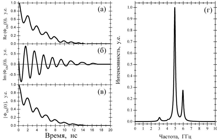
Рис. 6.1. Пример рассчитанного спектра ОМ (г) и соответствующая ему корреляционная функция (а-в) для системы ТБТ/ПИБ при T = 2 К, время измерения, t_m = 120 с.
