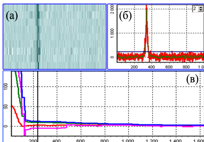
Рис. 6.3. Иллюстрация к процедуре расчета моментов применительно к измеренному спектру ОМ (ТБТ/ПИБ, T=2\text{K} ) (screenshots программы обработки измеренных данных). (а) Спектральная траектория. (б) Спектр ОМ, полученный путем суммирования всех спектров в спектральной траектории. (в) Зависимость расчетных первых четырех моментов от уровня дискриминации. Уровень дискриминации изображен горизонтальной (б) и вертикальной (в) линиями.
