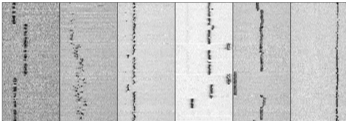
Рис. 5.19. Примеры спектральных траекторий ОМ для ТБТ в ПИБе с молекулярным весом M_w=34000 г/моль. T=4,5\text{K} , диапазон сканирования составляет 30 ГГц, число спектральных точек на скан – 1000, время на одну спектральную точку – 25 мс, количество сканов в спектральных траекторий – 100.
