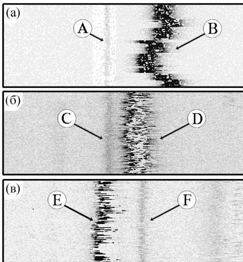
Рис. 5.11. Мерцающая флуоресценция в спектрах одиночных молекул. Примеры спектральных траекторий, измеренных для ТБТ/ПИБ (420000 г/моль) при T = 4,5 К, показывающие наличие в спектрах возбуждения флуоресценции молекул В, D и E короткоживущих «провалов», которые проявляются как белые «промежутки» на темном фоне спектральных пиков. «Время жизни» указанных «провалов» распределено в диапазоне от миллисекунд (а) до секунд (в).
