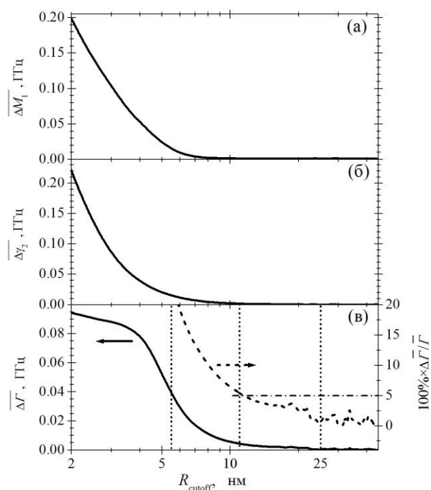
Рис. 6.8. Определение характерных зон взаимодействия ДУС с хромофором. Зависимости величин среднеквадратичных отклонений значений первых моментов \overline{\Delta M_1} (а), вторых моментов \overline{\Delta \gamma_2} (б) и ширин спектральных пиков \overline{\Delta \Gamma} (в) модельных спектров одиночных молекул от величины минимального радиуса R_{\text{cutoff}} . Этот радиус ограничивает снизу сферический слой, взаимодействие с двухуровневыми системами внутри которого учитывается при расчете спектров ОМ. Штриховая линия на (в) показывает процентное отношение среднего отклонения значений ширины спектральных линий \overline{\Delta \Gamma} к среднему значению ширины \bar{\Gamma} . Последняя зависимость используется для определения нижней границы зоны одинаковых ширин (точка, где \overline{\Delta \Gamma}/\bar{\Gamma}=5\% , детали см. в тексте). Вертикальные пунктирные линии демонстрируют положение границ между различными зонами взаимодействия ДУС с хромофорами. Расчеты проведены для системы ТБТ в ПИБе (температура 2 К, время измерения 120 с).
