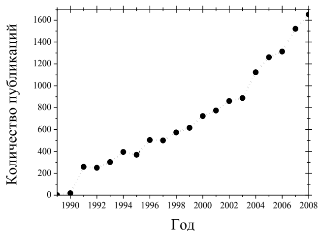
Рис. 2.1. Количество публикаций, содержащих ключевые слова «single molecule» и «fluorescence»/«luminescence». (Согласно международной базе данных об индексах цитирования «ISI-Web of Science»).
