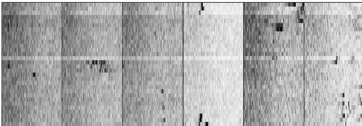
Рис. 5.18. Примеры спектральных траекторий ОМ для ТБТ в ПИБе с молекулярным весом M_w=2500 г/моль. T=4.5\text{K} , диапазон сканирования составляет 30 ГГц, число спектральных точек на скан – 500, время на одну спектральную точку – 90 мс, количество сканов в спектральных траекторий – 30.
