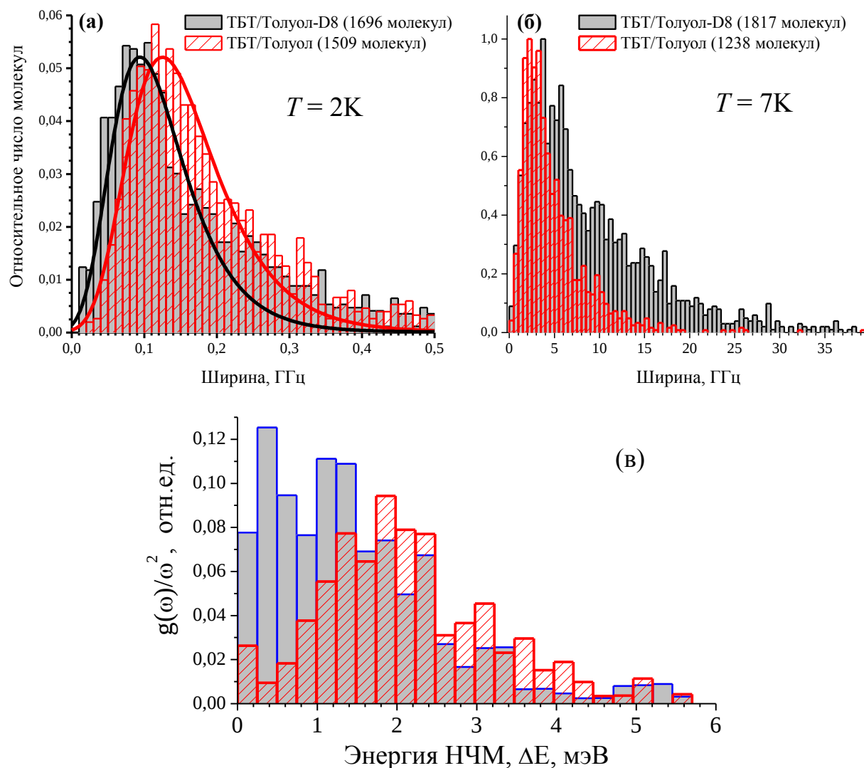
Рис. 6.15. Распределения ширин спектров одиночных молекул в толуоле и дейтерированном толуоле при T=2\text{K} (а) и T=7\text{K} (б) и энергетические спектры НЧМ для указанных систем, измеренные методом СОМ.
