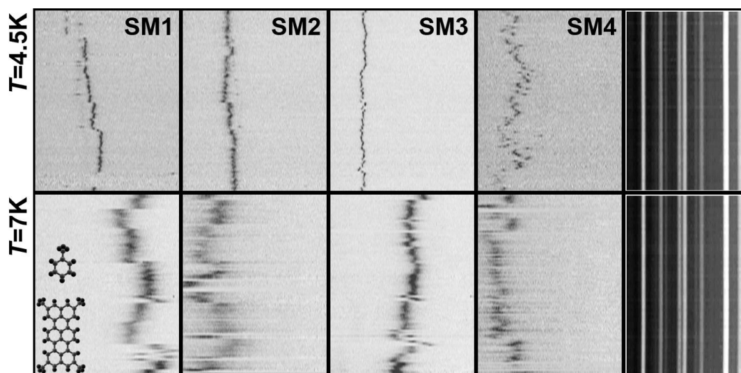
Рис. 5.14. Примеры спектральных траекторий четырех ОМ тетра-терт-бутилтеррилена в замороженном толуоле при T = 4,5\text{K} (верхние графики) и при T = 7\text{K} (нижние графики). Диапазон сканирования – 30 ГГц, каждый из них разбит на 1000 спектральных точек, количество сканов в каждой траектории равно 100, время одного скана – 20 с (20 мс на одну спектральную точку). Два самых правых графика демонстрируют спектр поглощения йодной ячейки, которая используется для контроля стабильности перестройки лазера.
