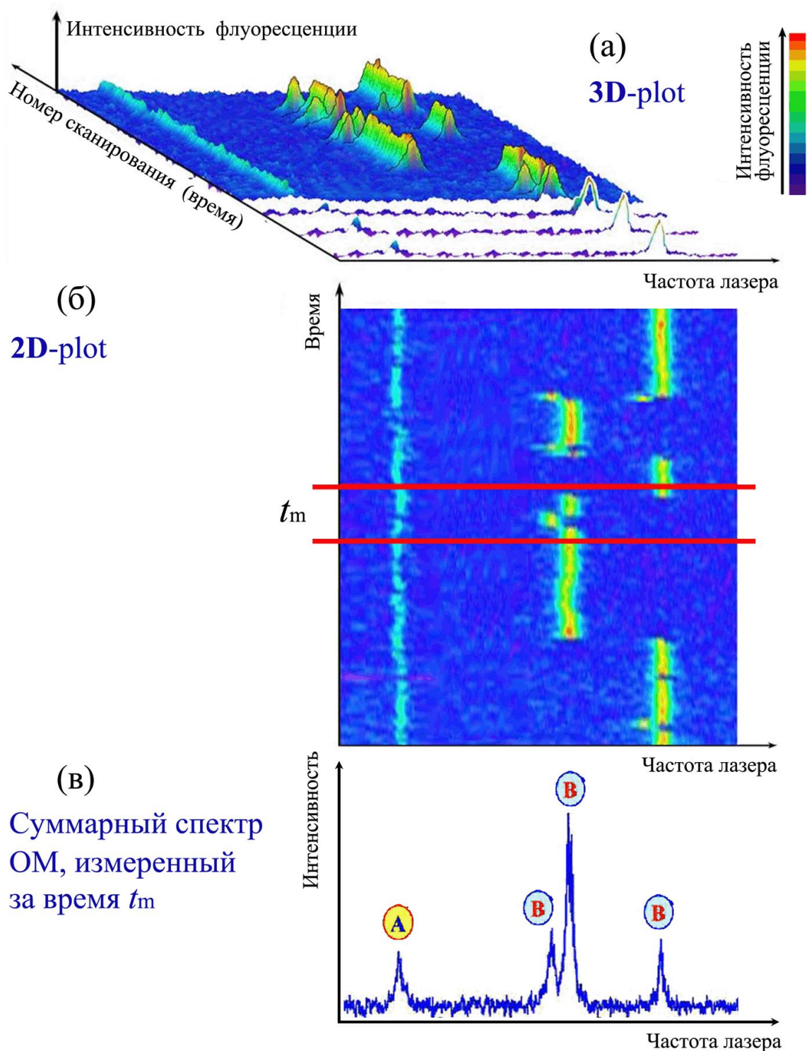
Рис. 3.1. Пример временной эволюции спектров двух одиночных молекул ТБТ, внедренных в ПИБ, регистрируемых многократно при T = 2 К (а,б). Результаты измерений представлены в виде трехмерной (а) и двухмерной (б) картин. Цветовая гамма точек на (а) и (б) поставлена в соответствие с интенсивностью флуоресценции. Результирующий интегральный спектр (в) соответствует сумме всех спектров в выбранном временном интервале t_m = 120 с, показанном на (б) сплошными горизонтальными линиями. Суммарный спектр на (в) соответствует двум молекулам: молекуле А (синглет) и молекуле В (триплет).
