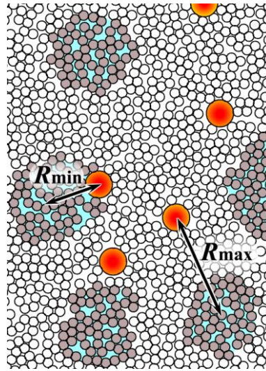
Рис. 6.17. Схематичное представление двумерной модели стекла и НЧМ, состоящего из круглых частиц. Маленькие круги представляют атомы (или молекулы) стекла. Большие круги соответствуют примесным молекулам. Атомы, вовлеченные в гипотетические НЧМ, выделены серым цветом. Стрелками обозначены характеристические минимальные и максимальные расстояния между ОМ и НЧМ, которые определяются пространственными размерами локализации и средними расстояниями между ними, соответственно.
