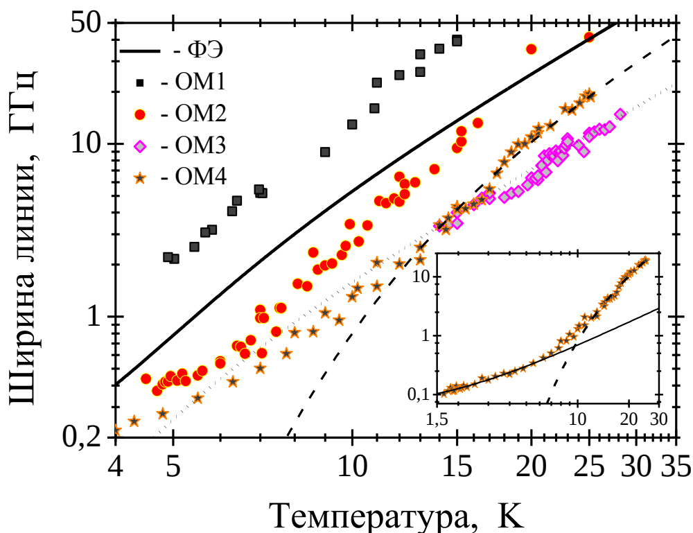
Рис. 5.4. Экспериментальные температурные зависимости ширины спектральных линий четырех одиночных молекул ТБТ в ПИБе ( M_w=420000 г/моль) (значки) и температурная зависимость обратного времени оптической дефазировки, измеренная с использованием техники некогерентного ФЭ (сплошная линия). Пунктирная и штриховая линии – результат аппроксимации экспериментальных данных с использованием зависимости (1.17). На вставке изображена температурная зависимость ширины спектральной линии одной из ОМ в широком температурном диапазоне. Сплошной и штриховой линиями на вставке показаны вклады в уширение спектральной линии от взаимодействия с ДУС и НЧМ, соответственно (см. формулы (1.17, 2.4, 5.3)).
