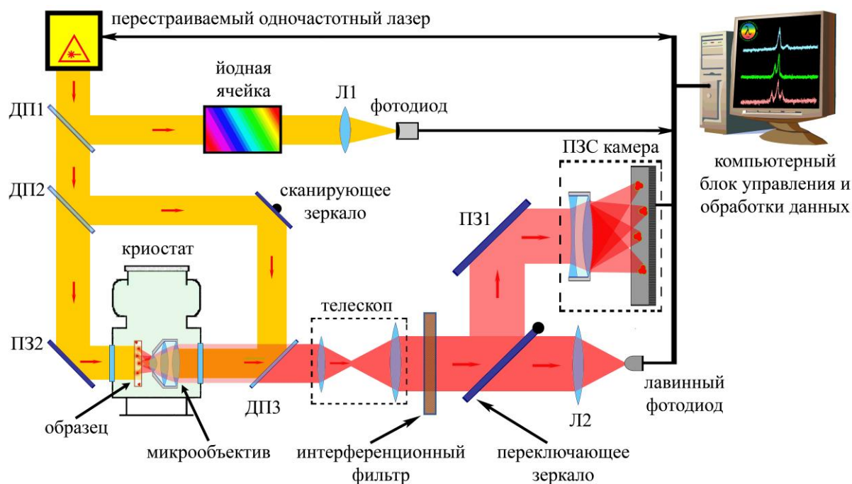
Рис. 3.5. Принципиальная схема установки для регистрации спектров возбуждения флуоресценции одиночных молекул. Переход между двумя режимами работы – конфокальной схемой с одноканальным приемником и схемой люминесцентного микроскопа с многоканальной системой регистрации – осуществляется с помощью переключающего зеркала. Интерференционный фильтр позволяет отсеять рассеянное лазерное излучение несмещенной частоты и пропускает стоксовую компоненту флуоресценции детектируемых молекул. Йодная ячейка использовалась для контроля стабильности частоты лазера. Обозначения на схеме: Л1, Л2 – собирающие линзы, ДП1, ДП2, ДП3 – светоделительные пластинки; ПЗ1, ПЗ2 – поворотные зеркала.
