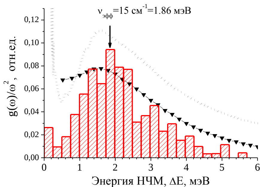
Рис. 6.13. Энергетический спектр НЧМ и бозонный пик в замороженном толуоле, измеренные тремя различными методами. Гистограмма - спектр НЧМ, измеренный методом СОМ в замороженном толуоле с примесью ТБТ. Данные по СОМ нормированы на Бозе фактор в соответствии с температурными диапазонами измерений. Треугольники - бозонный пик, измеренный методом рассеяния на ядрах в толуоле, допированном молекулами ферроцена, штриховая линия - измеренный методом КРС бозонный пик в чистом толуоле без примесей ( T=7\text{K} ). Стрелка отображает «эффективную» частоту НЧМ, измеренную методом ФЭ в толуоле, допированном молекулами ZnOЭП.
