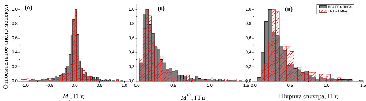
Рис. 6.20. Распределения первых двух спектральных моментов (а, б) и ширин линий (в) молекул ТБТ и молекул ДБАТТ в аморфном ПИБе ( M_w = 420000 г/моль). T = 2 К, время измерения спектров 120 с, ТБТ (штрихованная гистограмма, 244 молекулы), ДБАТТ (серая гистограмма, 855 молекул).
