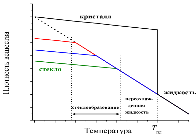
Рис. 1.1. Иллюстрация к процессу стеклования: плотность как функция температуры в различных фазах вещества.
