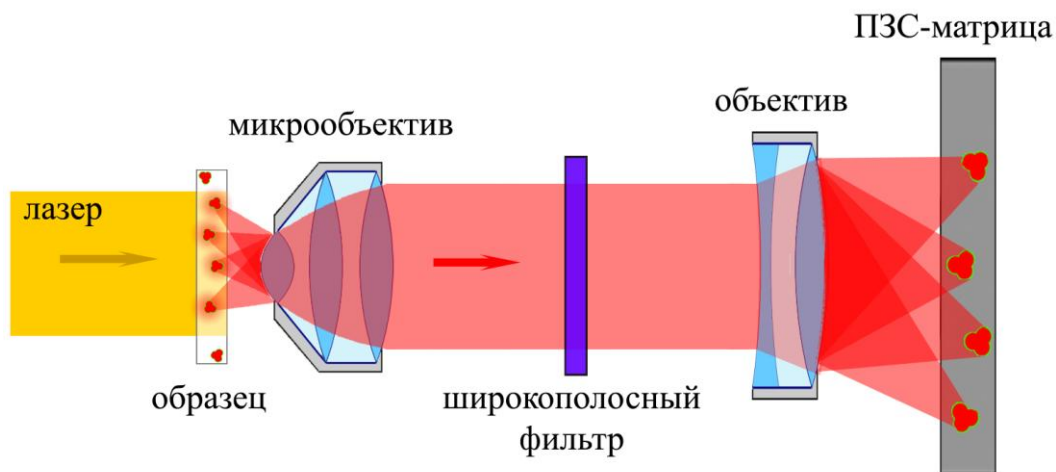
Рис. 2.6 Принципиальная схема возбуждения и регистрации спектров одиночных примесных молекул в твердых матрицах с использованием многоканальной схемы с высокочувствительным матричным фотодетектором на основе ПЗС-матрицы.
