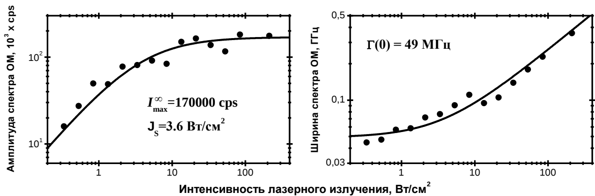
Рис. 3.6. Пример зависимостей амплитуды и ширины спектра ОМ от интенсивности лазерного излучения (на примере системы Тер/о-ДХБ, T=1,5 \text{ К} ).
