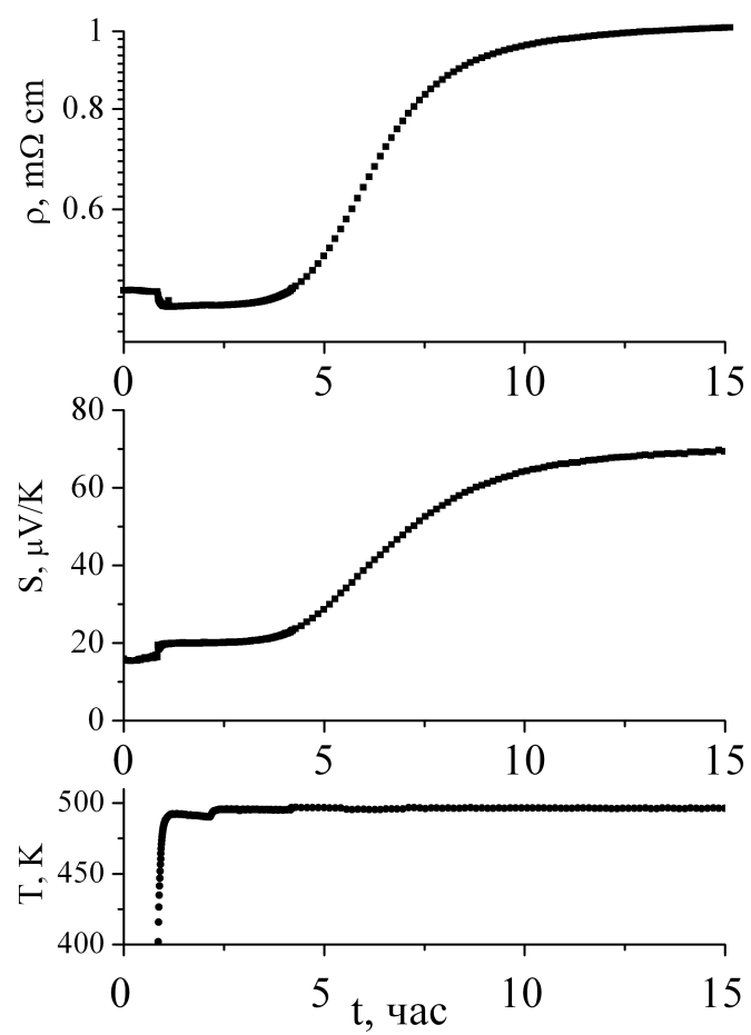
Рис. 3.13: Зависимость электрического сопротивления и термоэдс плёнки \text{CrSi}_2 от времени изотермического отжига при температуре 496 К.
