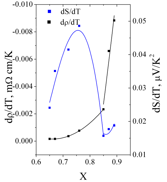
Рис. 4.12: Зависимость производной удельного сопротивления и термоэдс по температуре аморфной фазы плёнок \text{Cr}_{1-x}\text{Si}_x в интервале 320-350 К.
