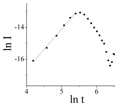
Рис. 3.23: Временная зависимость скорости нуклеации пленки \text{Cr}_{0.35}\text{Si}_{0.65} в логарифмическом масштабе.
