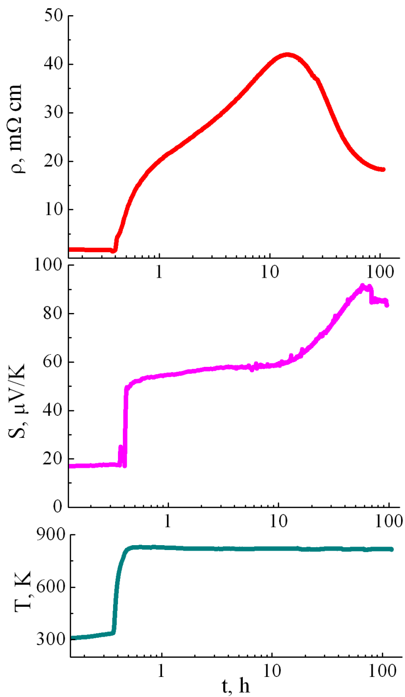
Рис. 3.16: Зависимость термоэдс ( S ) и удельного сопротивления ( \rho ) плёнки \text{C}_{0.15}\text{Si}_{0.85} толщиной 100 нм от времени отжига.
