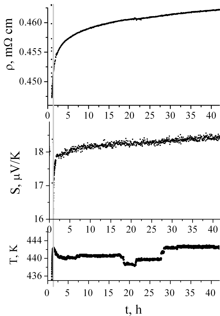
Рис. 3.6: Изменение термоэлектрических свойств плёнки 125 нм \text{CrSi}_2 при фиксированной температуре отжига ( T > T_{\text{so}} ).
