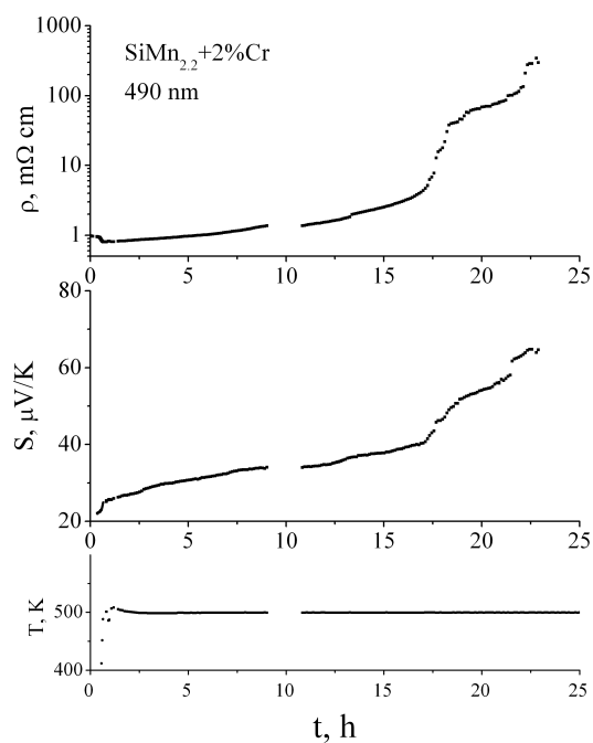
Рис. 3.25: Изменение термоэлектрических свойств плёнки \text{MnSi}_{2.2}+2\% \text{ Cr} в ходе отжига при фиксированной температуре.
