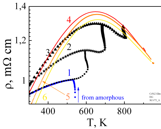
Рис. 3.18: Температурные зависимости термоэдс ( S ) и удельного сопротивления ( \rho ) плёнки \text{CrSi}_2 толщиной 100 нм. Начиная со стадии 4 происходит уменьшение сопротивления относительно предыдущих этапов, что указывает на появление перколяционного кластера.
