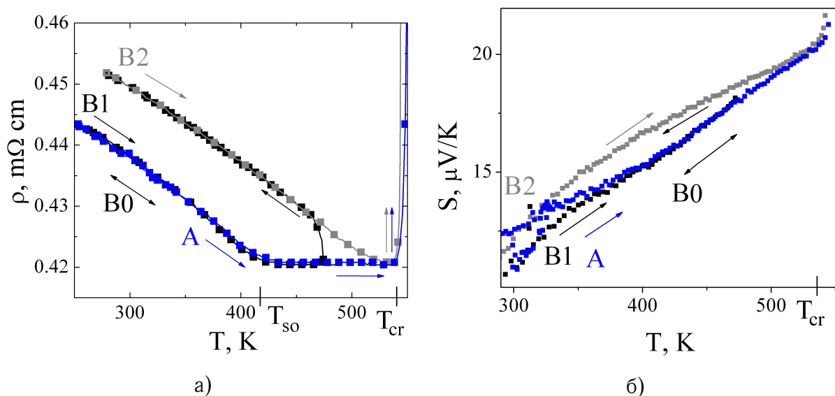
Рис. 3.3: Температурные зависимости удельного сопротивления а) и термоэдс б) для 164 нм плёнки CrSi 2 . Скорость нагрева 5 K/мин.
