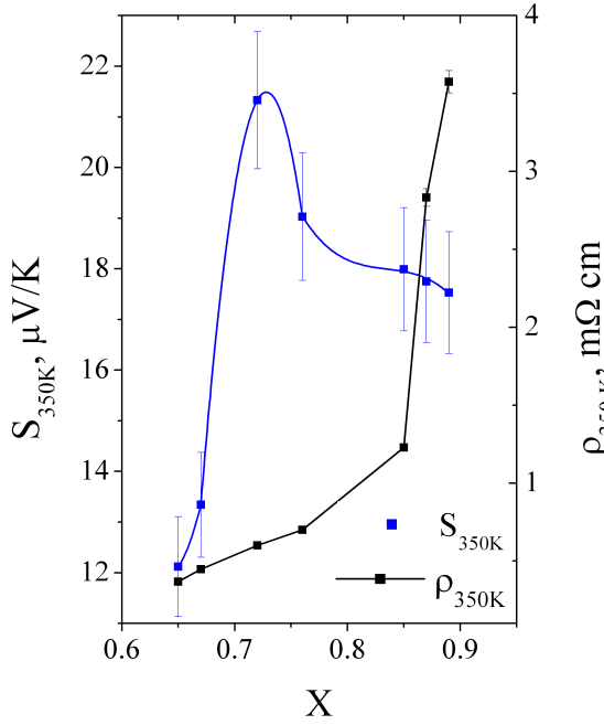
Рис. 4.11: Зависимость удельного сопротивления и термоэдс аморфной фазы плёнок \text{Cr}_{1-x}\text{Si}_x при температуре 350 К.
