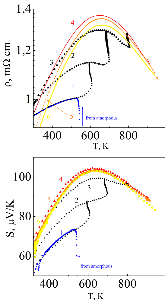
Рис. 4.14: Зависимость удельного сопротивления и термоэдс от температуры на разных стадиях отжига плёнки \text{CrSi}_2 .
