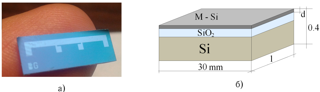
Рис. 2.1: Тонкая аморфная плёнка, полученная методом магнетронного распыления на холодную Si/SiO 2 подложку. Толщины образцов (d) варьировались от 21 до 500 нм.
