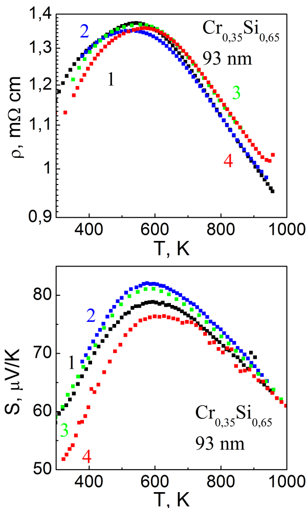
Рис. 4.15: Зависимость удельного сопротивления и термоэдс от температуры на разных стадиях отжига плёнки \text{Cr}_{0.35}\text{Si}_{0.65} .
