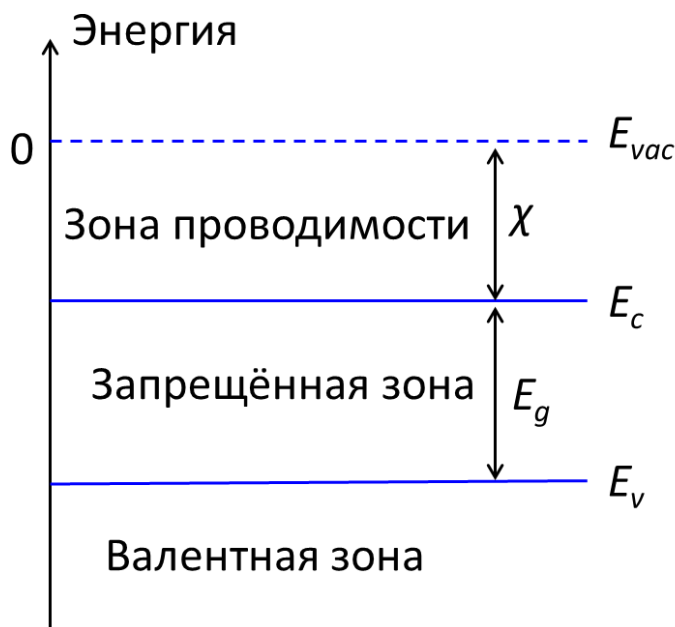
Рис. 2. Энергетические зоны полупроводника. E_{vac} – вакуумный уровень, \chi – электронное сродство, E_c – нижний край зоны проводимости, E_g – ширина запрещённой зоны, E_v – верхний край валентной зоны.
