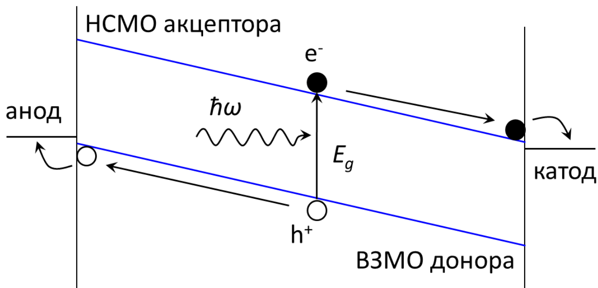
Рис. 12. Модель органического фотоэлемента с объёмным гетеропереходом.
