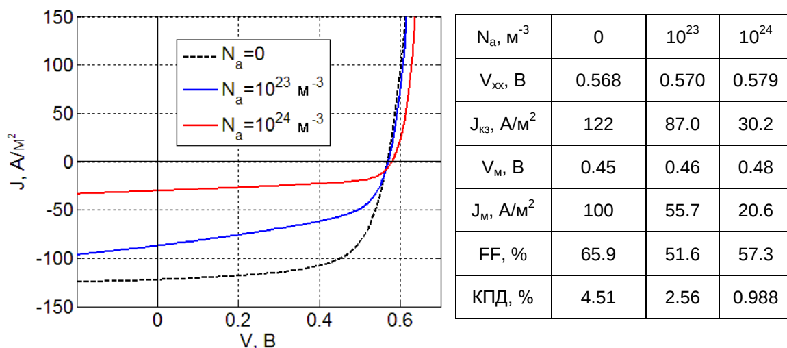
Рис. 26. Вольтамперные характеристики при различных концентрациях легирующих примесей акцепторного типа N_a .
