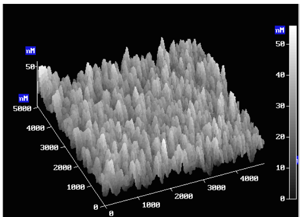
Рис. 71. Изображение поверхности неотожжённой плёнки на основе РЗНТ:ИФ3 1:1, полученное с помощью АСМ.
