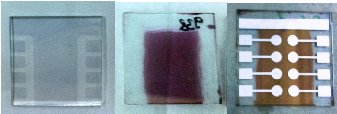
Рис. 20. Фотографии образцов СФ на различных стадиях приготовления, слева направо: чистая стеклянная подложка с паттернированным ИТО, та же подложка с нанесённым активным слоем и готовый образец с напылёнными металлическими электродами.
