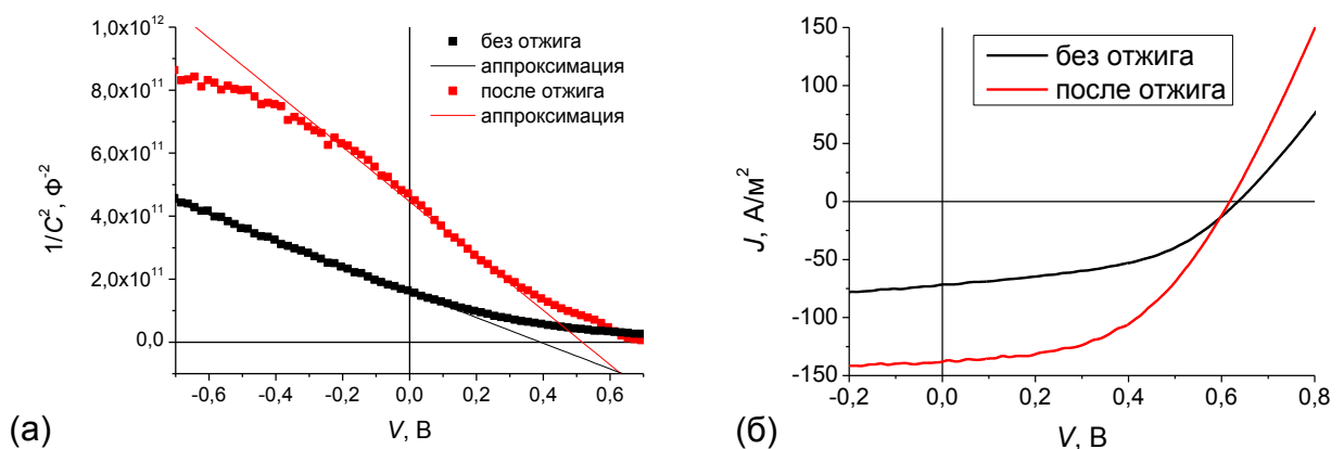
Рис. 63. Экспериментальные зависимости обратного квадрата ёмкости 1/C^2 от постоянной компоненты приложенного напряжения для отожжённого при 130°C в течение 15 минут в аргоне и неотожжённого образца с РЗНТ и их аппроксимация по формуле (2.2) (а) и ВАХ при освещении неотожжённого и отожжённого образцов органических СФ на основе РЗНТ:PCBM (б), изготовленных в тех же условиях, что и образцы с РЗНТ.
