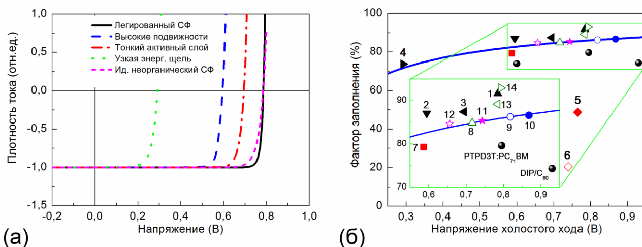
Рис. 57. ВАХ двухслойных органических СФ с различными задаваемыми параметрами и ВАХ идеального неорганического СФ (а) и их факторы заполнения на диаграмме FF-V_{XX} (б). Точки 1-14 соответствуют моделированным СФ, описанным в основном тексте, черными сферами показаны наиболее высокие значения FF , достигнутые в эксперименте.
