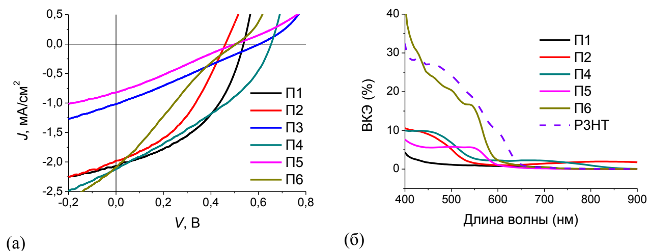
Рис. 66. Измеренные ВАХ органических СФ на основе узкозонных полимеров П1 – П6 в смеси с РСВМ (1:1) (а) и спектры их внешней квантовой эффективности (б). Штриховая линия соответствует опорному образцу на основе РЗНТ:РСВМ.
