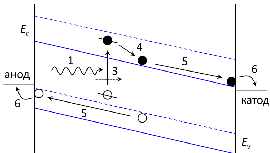
Рис. 7. Энергетическая диаграмма фотоэлемента на основе объёмного гетероперехода. Штриховые линии – НСМО и ВЗМО донора, сплошные линии – НСМО и ВЗМО акцептора.
