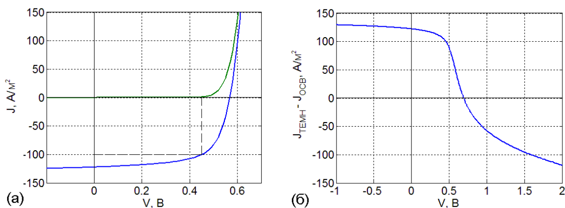
Рис. 25. Рассчитанные вольтамперные характеристики фотоэлемента с объёмным гетеропереходом в темноте (синяя кривая) и при освещении (зелёная кривая) (а) и их разность (б). Штриховыми линиями показана точка максимальной мощности.
