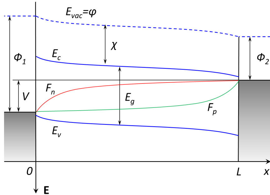
Рис. 11. Энергетическая зонная диаграмма для слоя полупроводника толщиной L , находящегося между двумя электродами с работами выхода \Phi_1 и \Phi_2 . Напряжение, приложенное к электродам, равно V . На контактах металл-полупроводник x=0 и x=L вакуумный уровень и квазиуровни Ферми F_n и F_p непрерывны.
