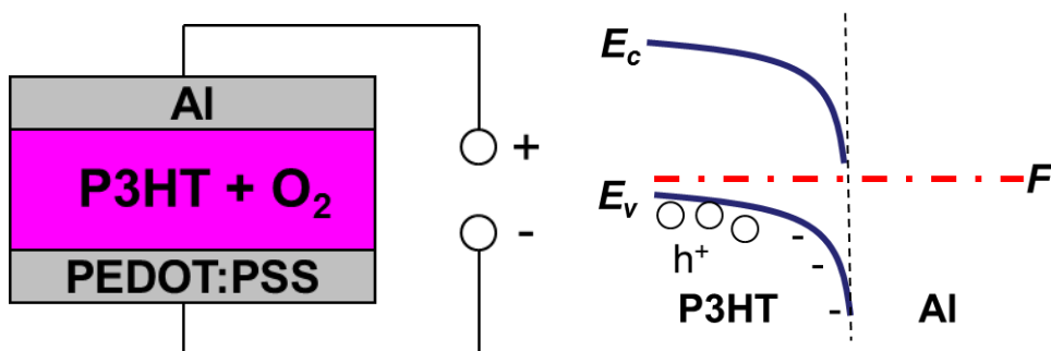
Рис. 62. Схема образца РЗНТ, p -легированного кислородом, между электродами из Al и PEDOT:PSS, используемого в методе импеданс-спектроскопии (слева). Энергетическая диаграмма барьера Шоттки на контакте РЗНТ и Al (схематически).
