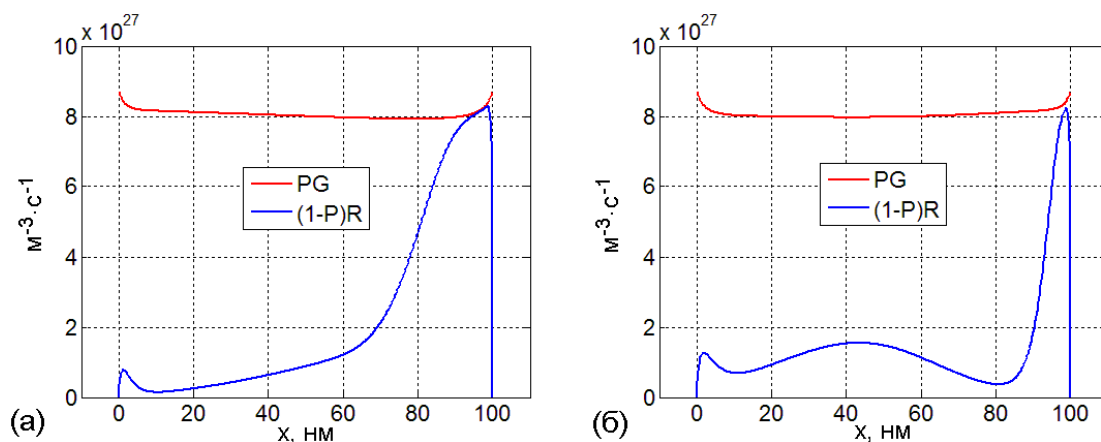
Рис. 41. Скорости генерации PG и рекомбинации (1-P)R свободных носителей заряда при \mu_p/\mu_n=10^{-2} в отсутствии примесей (а) и при концентрации примесей акцепторного типа N_a=6.1 \cdot 10^{22} \text{ м}^{-3} (б).
