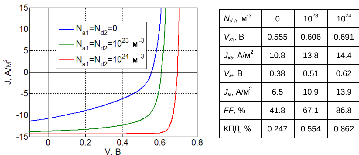
Рис. 47. Рассчитанные вольтамперные характеристики двухслойного фотоэлемента при K=0.1 при различных концентрациях легирующих примесей.
