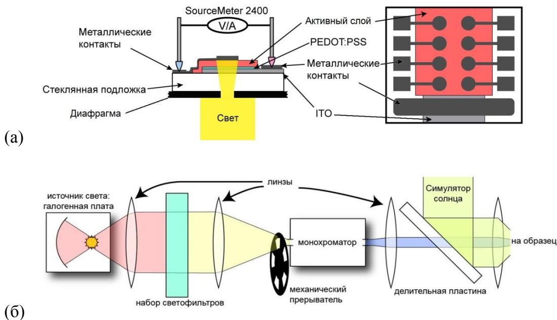
Рис. 21. Схематическое изображение образца солнечного фотоэлемента (а) и экспериментального стенда для измерения ВАХ и спектров ВКЭ (б).
