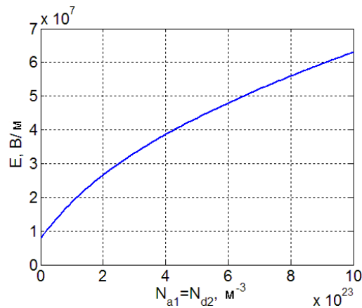
Рис. 49. Зависимость напряжённости поля на границе слоёв от концентрации легирующих примесей.
