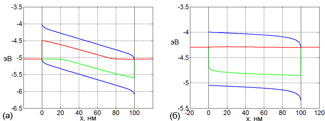
Рис. 42. Энергетические зонные диаграммы органического солнечного фотоэлемента в случае омических контактов \Phi_I=5.05 эВ (а) и при пониженной работе выхода левого электрода \Phi_I=4.3 эВ (б).
