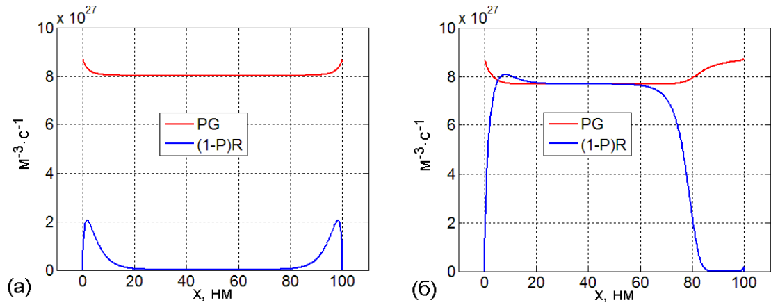
Рис. 29. Скорости генерации PG и рекомбинации (1-P)R свободных носителей заряда в отсутствии легирования (а) и при концентрации легирующих примесей N_a=10^{24} \text{ м}^{-3} (б).
