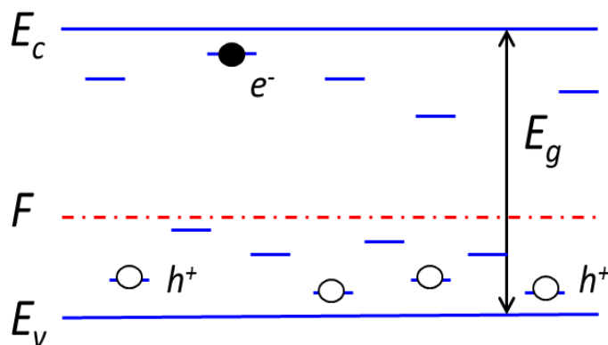
Рис. 14. Энергетическая диаграмма полупроводника с легирующими примесями. E_c – нижний край зоны проводимости, E_v – верхний край валентной зоны, F – уровень Ферми. Показаны энергетические уровни примесей, большинство которых электронейтрально, а небольшая часть ионизована. Примеси p -типа преобладают, примеси n -типа компенсированы.
