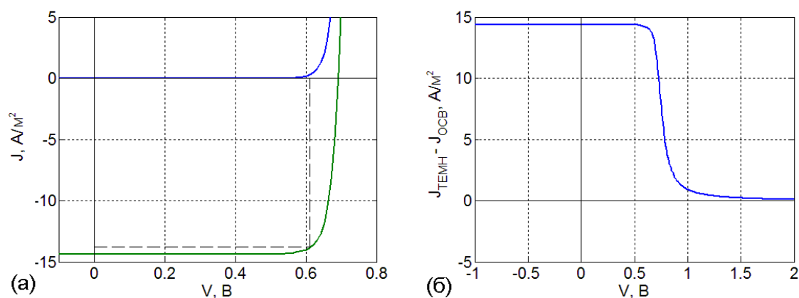
Рис. 46. Рассчитанные вольтамперные характеристики двухслойного органического фотоэлемента в темноте (синяя кривая) и при освещении (зелёная кривая) при отсутствии легирования, штриховыми линиями показана точка максимальной мощности (а). Разность темновой ВАХ и ВАХ при освещении (б).
