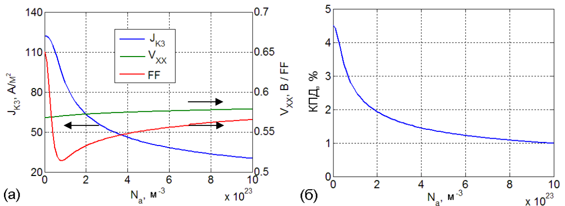
Рис. 31. Зависимости плотности тока короткого замыкания J_{KЗ} , напряжения холостого хода V_{XX} , фактора заполнения FF (а) и КПД (б) от концентрации легирующих примесей акцепторного типа N_a .
