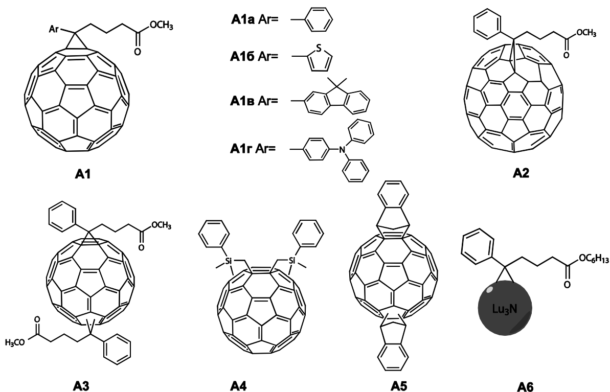
Рис. 17. Структурные формулы производных фуллеренов, используемых в качестве акцепторов в органических солнечных фотоэлементах.
