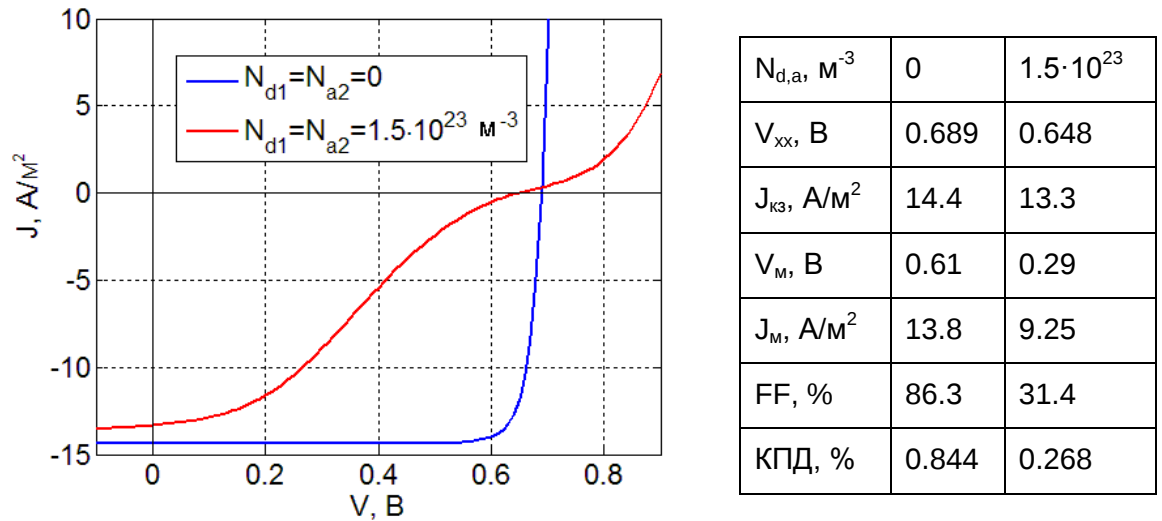
Рис. 52. Вольтамперные характеристики при K=100 в отсутствии легирования (синяя кривая) и при легировании слоёв N_{d1}=1.5 \cdot 10^{23} \text{ м}^{-3} и N_{a2}=1.5 \cdot 10^{23} \text{ м}^{-3} (красная кривая).
