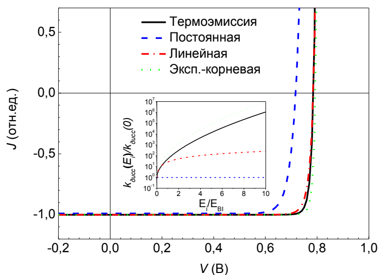
Рис. 61. ВАХ двухслойных органических СФ с различными формами полевой зависимости скорости диссоциации связанных электронно-дырочных пар k_{diss}(E_i) : в случае термоэмиссии по формуле (1.27а), постоянная скорость k_{diss} , линейная по формуле (3.27) и экспоненциально-корневая по формуле (3.28). Сами зависимости показаны на вставке в логарифмическом масштабе.
