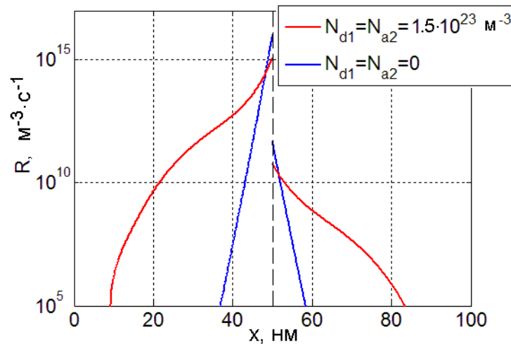
Рис. 54. Скорости бимолекулярной рекомбинации R в отсутствии легирования (синяя кривая) и при легировании слоёв (красная кривая).
