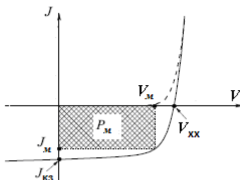
Рис. 9. Типичная вольтамперная характеристика солнечного фотоэлемента в темноте (штриховая линия) и при освещении (сплошная линия). Показаны плотность тока короткого замыкания J_{КЗ} и напряжение холостого хода V_{ХХ} . Максимальная выходная мощность пропорциональна произведению J_М \times V_М .
