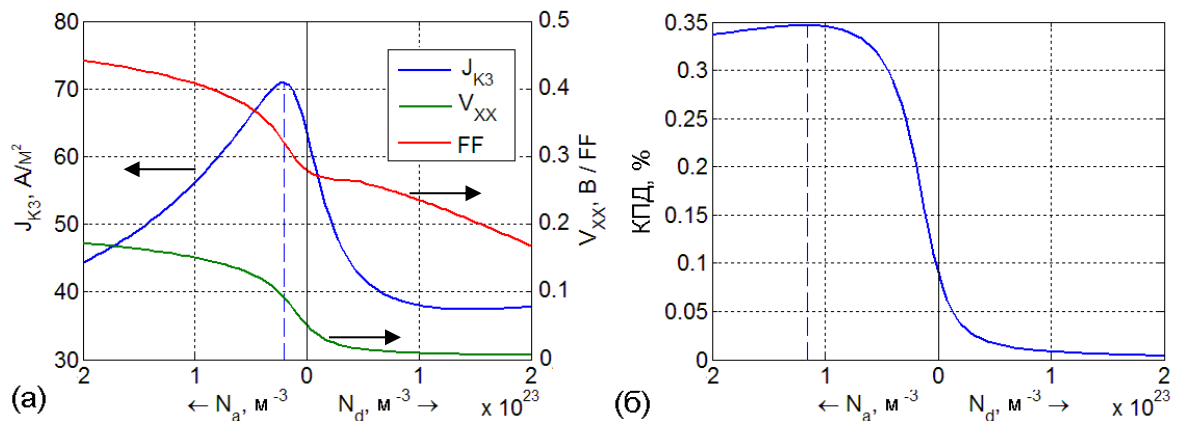
Рис. 44. Зависимости плотности тока короткого замыкания J_{K3} , напряжения холостого хода V_{xx} и фактора заполнения FF (а) и КПД (б) от концентраций легирующих примесей донорного N_d и акцепторного N_a типов при \Phi_I=4.3 эВ.
