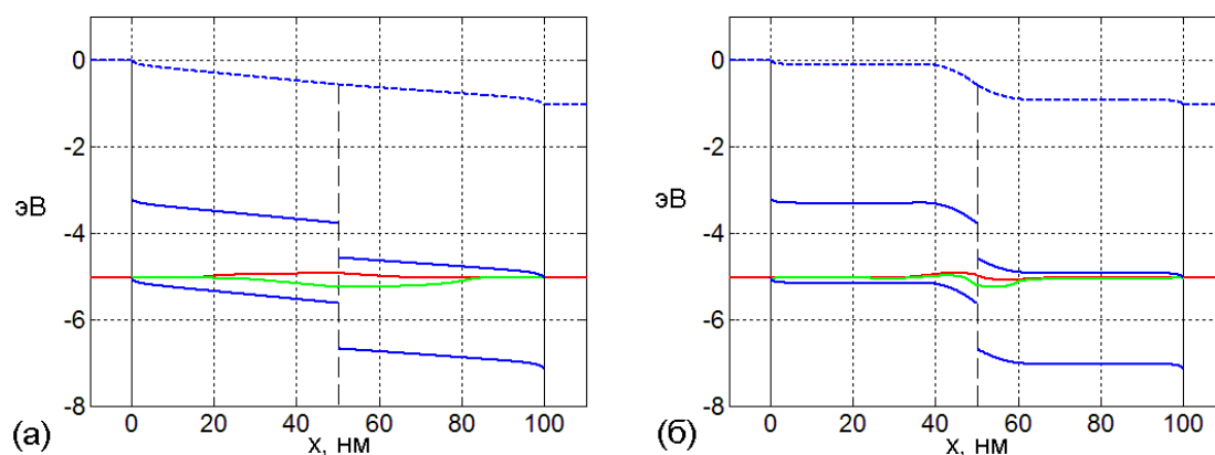
Рис. 48. Энергетические зонные диаграммы двухслойного фотоэлемента в отсутствии легирования (а) и при легировании (б). Левый (донорный) слой легирован примесями акцепторного типа N_{a1}=10^{24} \text{ м}^{-3} , а правый (акцепторный) слой легирован примесями донорного типа N_{d2}=10^{24} \text{ м}^{-3} . Вертикальная черная штриховая линия обозначает границу слоёв ( x=50 \text{ нм} ).
