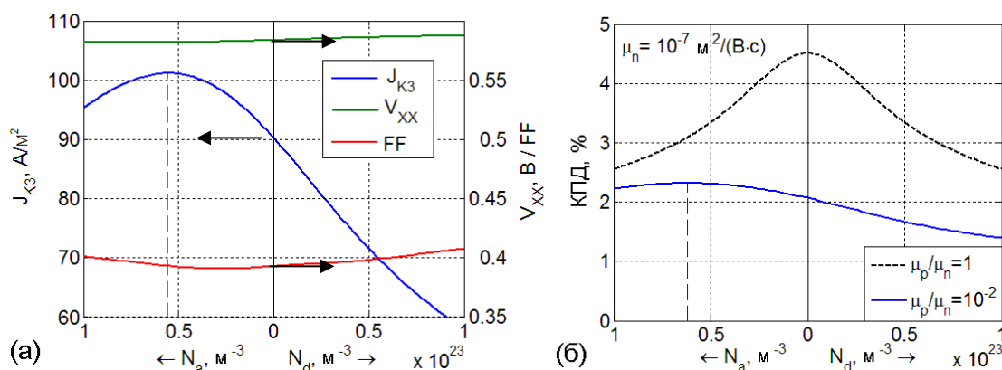
Рис. 39. Рассчитанные зависимости плотности тока короткого замыкания J_{K3} , напряжения холостого хода V_{xx} , фактора заполнения FF (а) и КПД (б) от концентрации легирующих примесей донорного N_d и акцепторного N_a типов при дисбалансе подвижностей электронов и дырок ( \mu_p/\mu_n=10^{-2} ). Чёрной штриховой линией показана зависимость КПД при балансе подвижностей ( \mu_p=\mu_n ).
