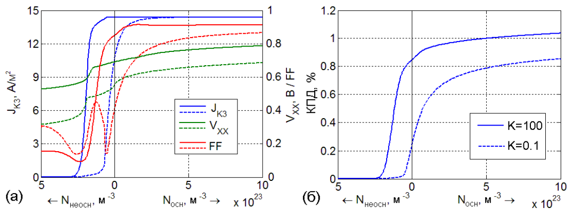
Рис. 51. Зависимости плотности тока короткого замыкания J_{K3} , напряжения холостого хода V_{XX} , фактора заполнения FF (а) и КПД (б) от концентраций легирующих примесей при легировании слоёв основными носителями N_{осн} \equiv N_{a1} = N_{d2} и неосновными носителями N_{неосн} \equiv N_{d1} = N_{a2} . Сплошные линии соответствуют случаю долгоживущих связанных электронно-дырочных пар ( K=100 ), штриховые линии соответствуют случаю K=0.1 .
