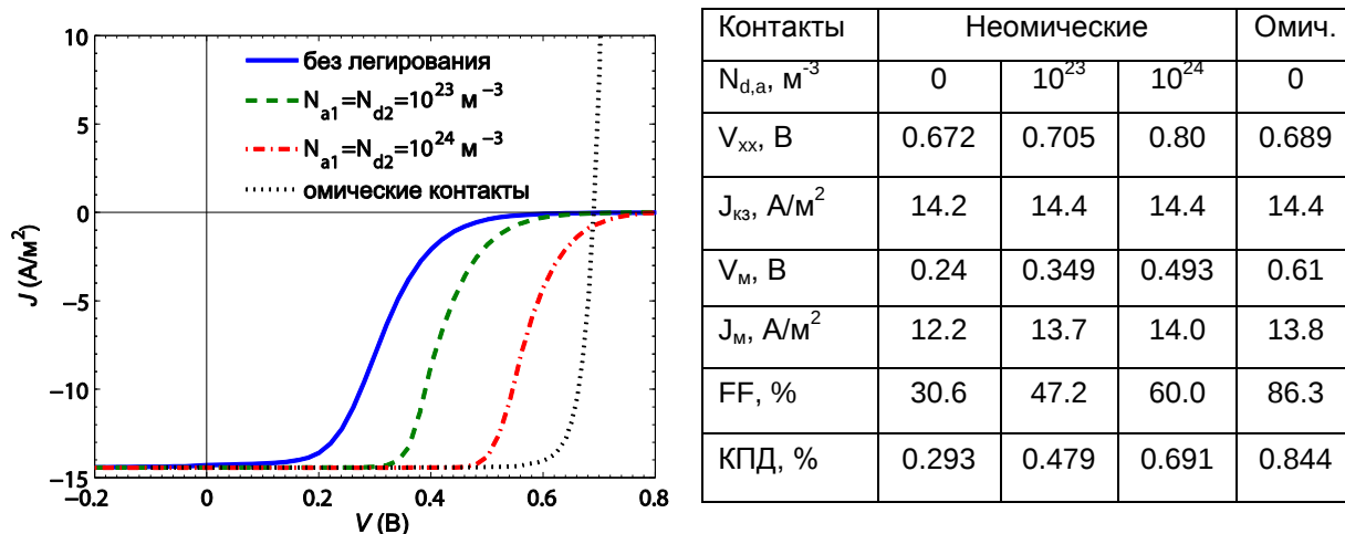
Рис. 56. ВАХ двухслойного органического СФ с неомическими контактами при различных уровнях легирования ( K=100 ). Для сравнения дана ВАХ нелегированного двухслойного органического СФ с омическими контактами (чёрная пунктирная кривая).
