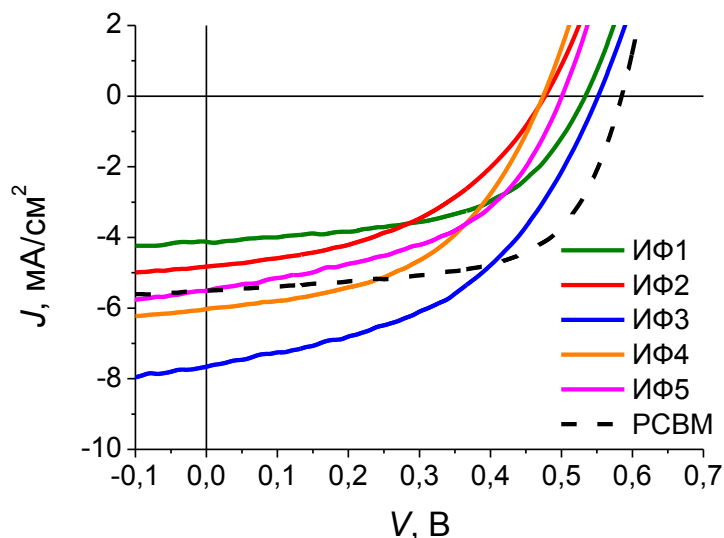
Рис. 69. Вольтамперные характеристики фотоэлементов на основе РЗНТ:ИФ1 – 5 и опорного образца на основе РЗНТ:РСВМ при соотношении полимер : фуллерен 1:1 при отсутствии отжига.
