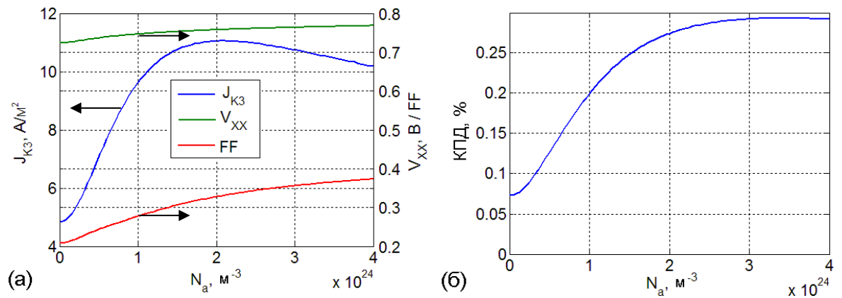
Рис. 37. Зависимости плотности тока короткого замыкания J_{K3} , напряжения холостого хода V_{XX} , фактора заполнения FF (а) и КПД (б) от концентрации легирующих примесей акцепторного типа N_a в случае низких подвижностей \mu_n = \mu_p = 10^{-11} \text{ м}^2/(\text{В} \cdot \text{с}) .
