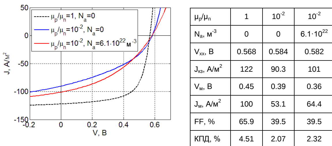
Рис. 38. Вольтамперные характеристики при дисбалансе подвижностей электронов и дырок ( \mu_p/\mu_n=10^{-2} ) в отсутствии легирования (синяя кривая) и при концентрации легирующих примесей N_a=6.1 \cdot 10^{22} \text{ м}^{-3} (красная кривая). Штриховой чёрной линией показана вольтамперная характеристика при балансе подвижностей ( \mu_p=\mu_n ) в отсутствии легирования.
