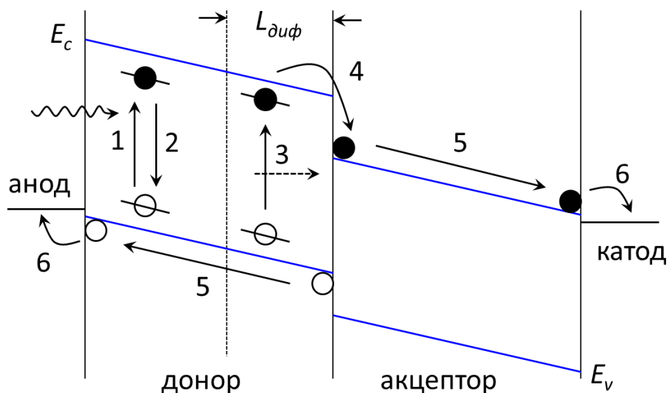
Рис. 5. Энергетическая диаграмма фотоэлемента на основе планарного гетероперехода (схематически). Схематически показаны процессы, происходящие при поглощении света. L_{diff} – длина диффузии экситона.
