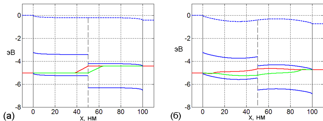
Рис. 53. Энергетические зонные диаграммы двухслойного фотоэлемента в точке максимальной мощности в отсутствии легирования (а) и при легировании слоёв N_{d1}=1.5 \cdot 10^{23} \text{ м}^{-3} и N_{a2}=1.5 \cdot 10^{23} \text{ м}^{-3} (б).
