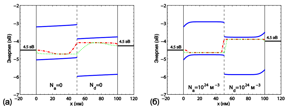
Рис. 55. Энергетические зонные диаграммы двухслойных органических СФ с неомическими контактами при отсутствии легирования (а) и при легировании основными носителями в точке максимальной мощности.
