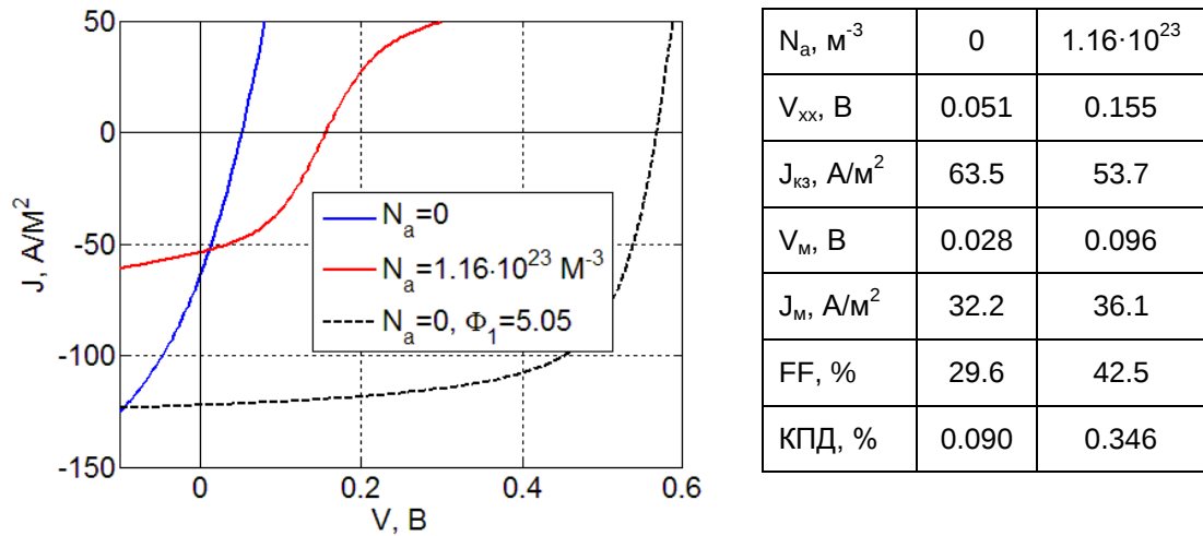
Рис. 43. Рассчитанные вольтамперные характеристики при \Phi_I=4.3 эВ в отсутствии легирования (синяя кривая) и при концентрации легирующих примесей акцепторного типа N_a=1.16 \cdot 10^{23} \text{ м}^{-3} (красная кривая). Для сравнения показана вольтамперная характеристика в случае омических контактов (чёрная штриховая линия).
