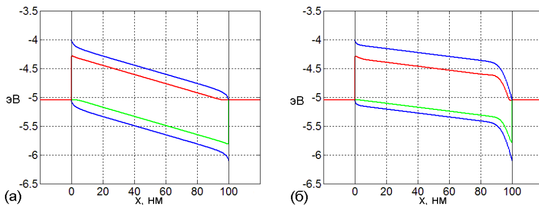
Рис. 33. Энергетические зонные диаграммы в случае низких подвижностей ( \mu_n = \mu_p = 10^{-11} \text{ м}^2/(\text{В} \cdot \text{с}) ) в отсутствии легирования (а) и при концентрации легирующих примесей N_a = 2 \cdot 10^{24} \text{ м}^{-3} (б).
