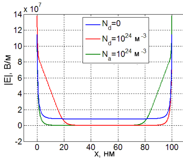
Рис. 28. Абсолютная величина напряжённости электрического поля |E| в активном слое в режиме короткого замыкания в отсутствие легирования и при легировании примесями донорного и акцепторного типов.
