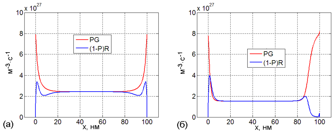
Рис. 35. Скорости генерации PG и рекомбинации (1-P)R свободных носителей заряда в случае \mu_n = \mu_p = 10^{-11} \text{ м}^2/(\text{В} \cdot \text{с}) в отсутствии легирования (а) и при концентрации легирующих примесей N_a = 2 \cdot 10^{24} \text{ м}^{-3} (б).
