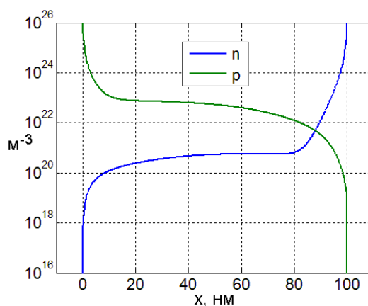
Рис. 40. Концентрации электронов n и дырок p в режиме короткого замыкания в случае дисбаланса подвижностей \mu_p/\mu_n=10^{-2} .
