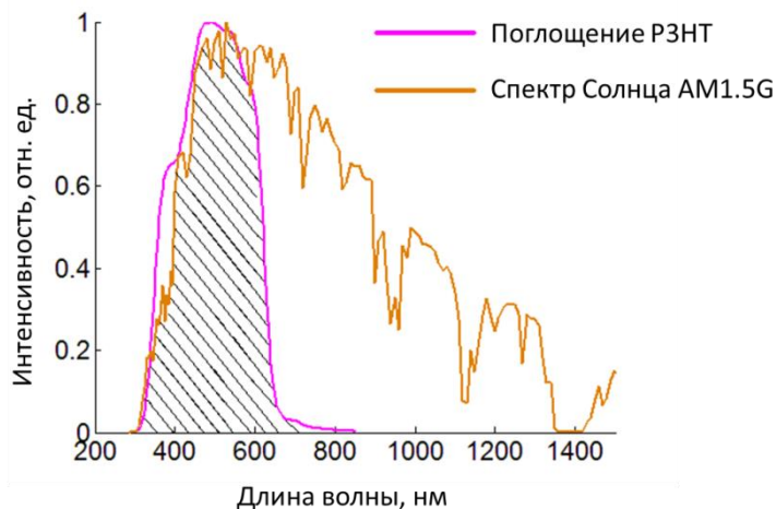
Рис. 15. Спектр солнечного излучения AM1.5G и спектр поглощения полимера РЗНТ (нормированные на максимум). Заштрихована область их перекрытия.
