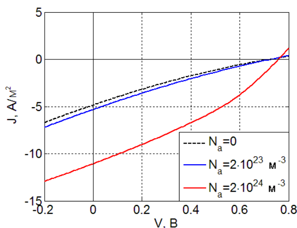
Рис. 32. Вольтамперные характеристики в случае низких подвижностей ( \mu_n=\mu_p=10^{-11} м 2 /(В·с)) при различных концентрациях легирующих примесей акцепторного N_a типа.
