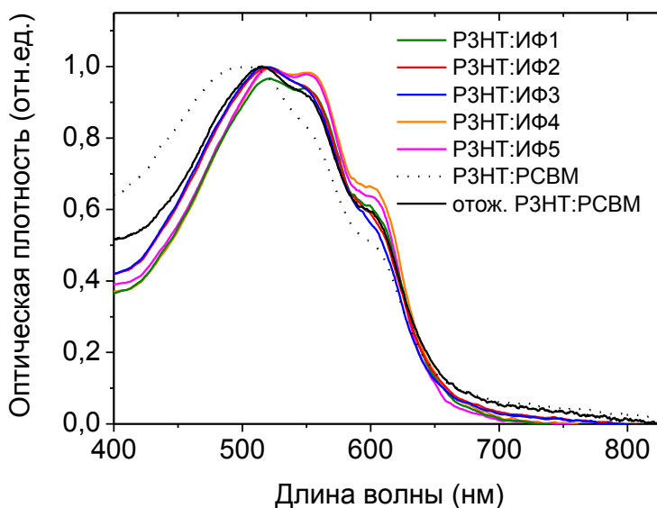
Рис. 70. Спектры поглощения плёнок смесей P3HT:ИФ1 – 5 и P3HT:PCBM. Пунктирная линия обозначает спектр поглощения плёнки P3HT:PCBM, подвергнутой термическому отжигу при 110°C в течение 15 мин.
