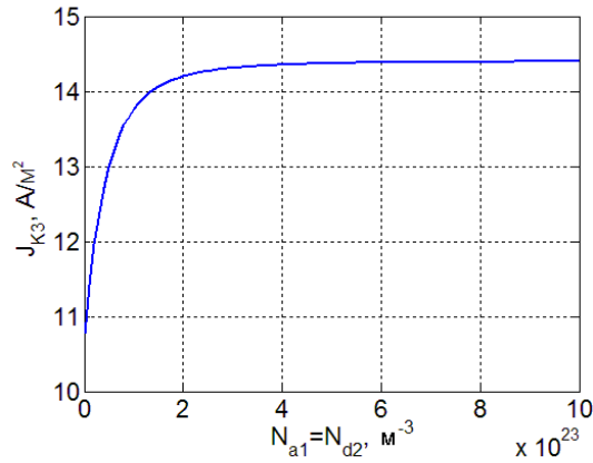
Рис. 50. Зависимость тока короткого замыкания от концентрации легирующих примесей.
