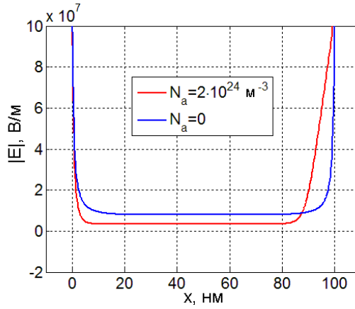
Рис. 34. Напряжённость электрического поля в активном слое в случае \mu_n = \mu_p = 10^{-11} \text{ м}^2/(\text{В} \cdot \text{с}) в отсутствии легирования и при концентрации легирующих примесей N_a = 2 \cdot 10^{24} \text{ м}^{-3} .
