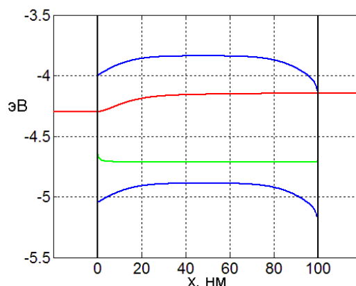
Рис. 45. Энергетическая зонная диаграмма в случае \Phi_1=4.3 эВ при концентрации легирующих примесей N_d=1.16 \cdot 10^{23} \text{ м}^{-3} в точке максимальной мощности.
