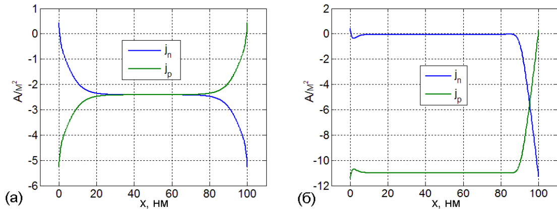
Рис. 36. Плотности токов электронов и дырок в случае \mu_n=\mu_p=10^{-11} \text{ м}^2/(\text{В}\cdot\text{с}) в отсутствии легирования (а) и при концентрации легирующих примесей N_a=2\cdot 10^{24} \text{ м}^{-3} (б).
