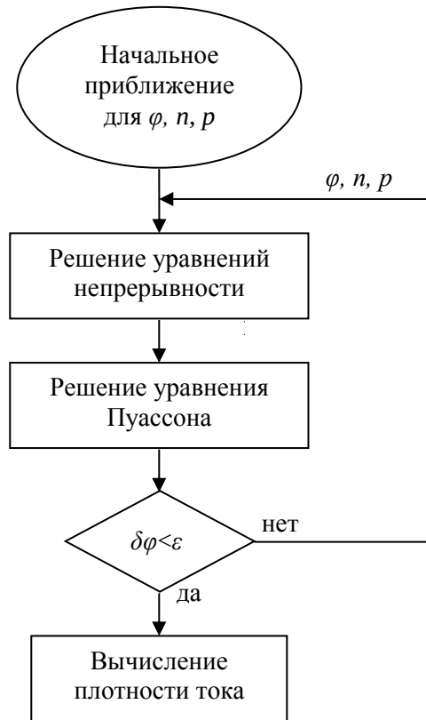
Рис. 24. Блок-диаграмма метода последовательных приближений.
