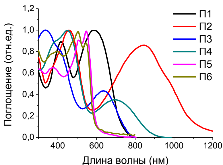
Рис. 64. Спектры поглощения полимеров П1 – П6 в плёнках.
