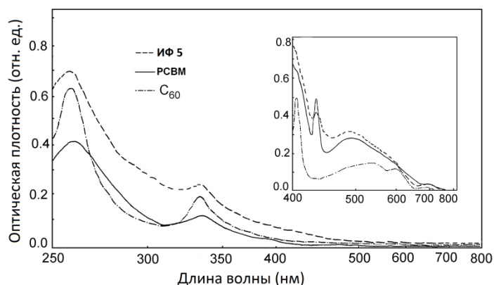
Рис. 68. Спектры поглощения растворов фуллерена C_{60} и его производных ИФ5 и РСВМ в дихлорметане ( 2 \cdot 10^{-5} моль/л, толщина кюветы 2 мм). На вставке показаны спектры при толщине кюветы 10 мм.
