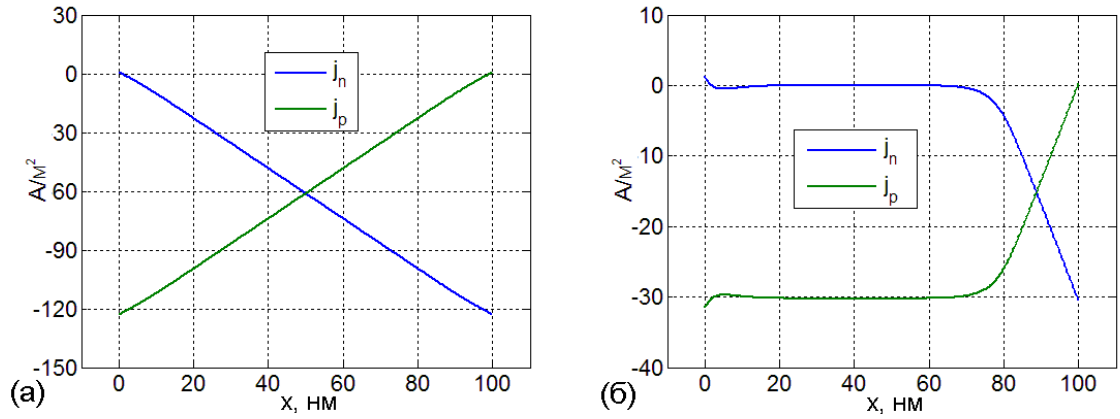
Рис. 30. Плотности токов электронов и дырок в активном слое в отсутствии легирования (а) и при концентрации легирующих примесей N_a=10^{24} \text{ м}^{-3} (б).
