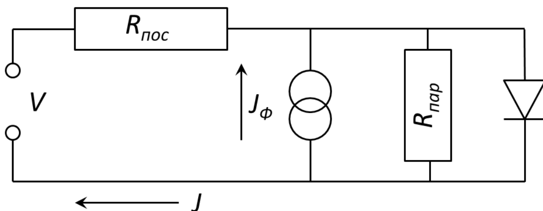
Рис. 10. Эквивалентный контур органического солнечного фотоэлемента.
