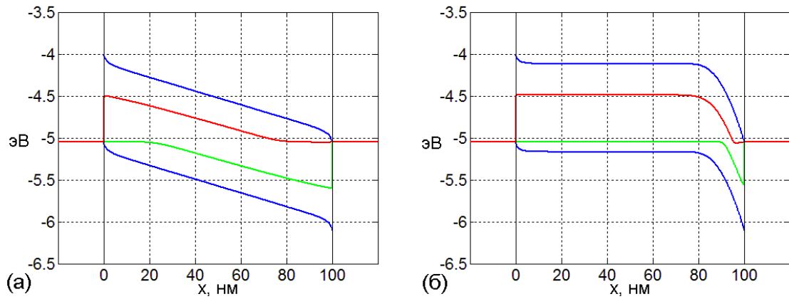
Рис. 27. Энергетические зонные диаграммы в режиме короткого замыкания при отсутствии легирующих примесей (а) и при концентрации примесей акцепторного типа N_a=10^{24} \text{ м}^{-3} (б). Здесь и далее: вертикальные черные линии обозначают границы электродов, синие сплошные линии – уровни E_c и E_v , красная линия – квазиуровень Ферми для электронов, а зелёная линия – для дырок.
