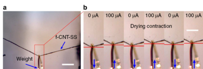
Рис. 8 а – Фотография 35 мг груза на волокне. Шкала 250 мкм. б – Под действием тока 100 мкА волокно сокращается на 1% (1.8 мм), и груз за время < 1 \text{ с} поднимается на 25 мкм (температура среды 23^\circ\text{C} , влажность 55%). Между циклами перерыв 1 ч. Шкала 150 мкм.
