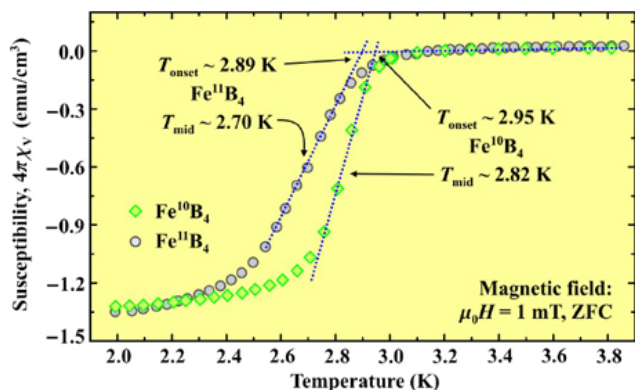
Рис. 1. Температурные зависимости магнитной восприимчивости монокристаллов \text{FeB}_4 с изотопами ^{10}\text{B} и ^{11}\text{B} .
