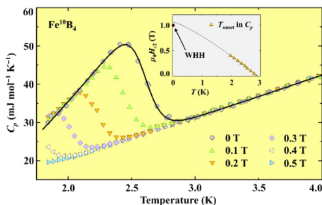
Рис. 2. Температурная зависимость удельной теплоемкости \text{FeB}_4 .
