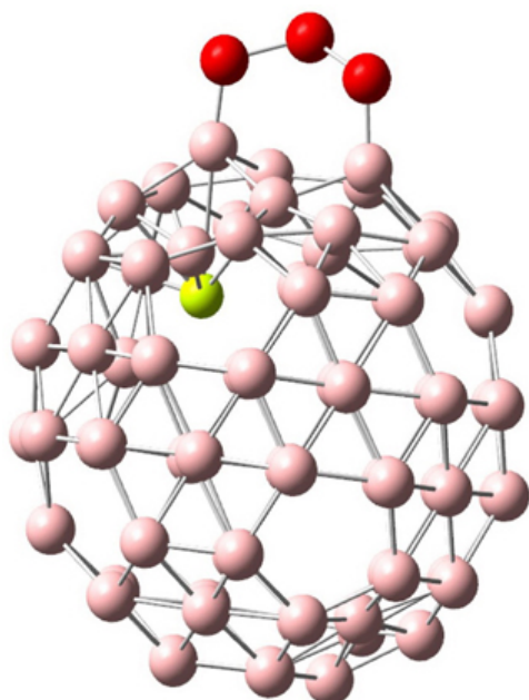
Рис. 2. Эндодраальный комплекс \text{Be@B}_{80} с адсорбированной на поверхности молекулой озона
