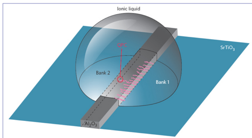
Рис. 1. Полоска \text{Al}_2\text{O}_3 ( 2 \text{ мкм} \times 50 \text{ нм} \times 5 \text{ нм} ) экранирует часть поверхности \text{SrTiO}_3 от ионной жидкости и разделяет ее на сверхпроводящие “берега”. Розовым цветом показаны проводящие каналы, образующиеся при увеличении напряжения на электроде. Красный кружок – квантовый точечный контакт (канал с максимальной проводимостью).
