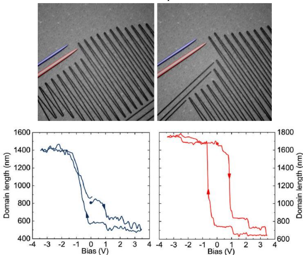
Рис. 1 Шипообразные сегнетоэластические домены в \text{BaTiO}_3 и соответствующие им петли гистерезиса: красная петля соответствует домену, упирающемуся в стенку из ряда перпендикулярных ему доменов, синяя петля соответствует домену, движущемуся в “свободном пространстве”. Размер кадра изображения в просвечивающем электронном микроскопе – 2.5 мкм.
