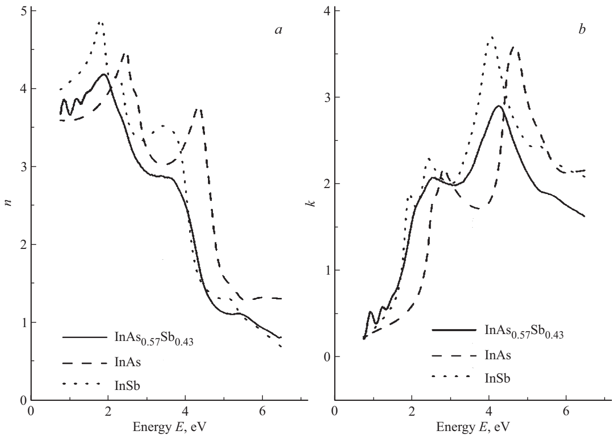
Рис. 5. Спектральные зависимости показателей преломления, n(E) , и экстинкции, k(E) , для гетероэпитаксиальной структуры \text{InAs}_{0.57}\text{Sb}_{0.43} и монокристаллов \text{InAs} , \text{InSb} [5].
