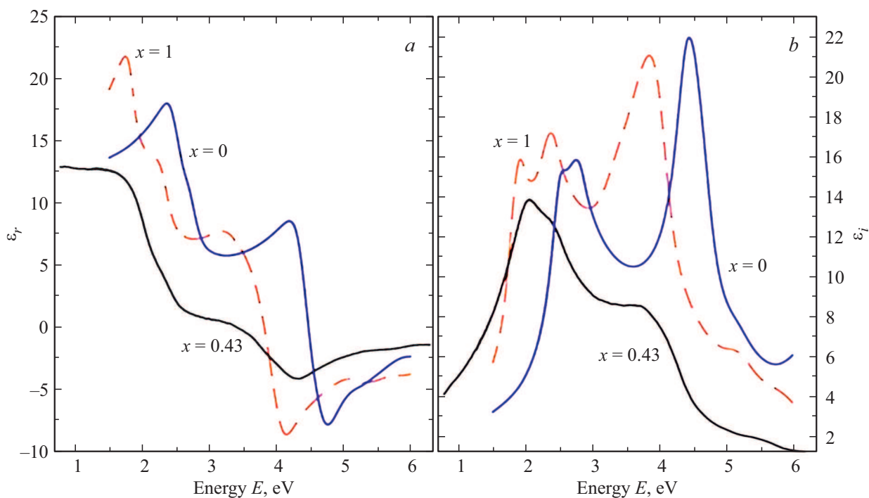
Рис. 4. Спектральные зависимости действительной (a) и мнимой (b) частей диэлектрической функции \text{InAs}_{0.57}\text{Sb}_{0.43} ( x = 0.43 ), \text{InAs} ( x = 0 ), \text{InSb} ( x = 1 ).
