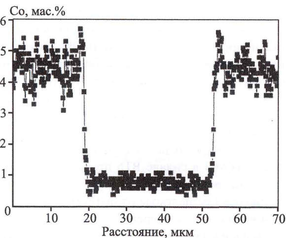
Рис. 3. РЭМ-изображение с линией сканирования поперек границы зерна \beta(\text{Ti,Co})/\beta(\text{Ti,Co}) (а) и концентрационный профиль, снятый вдоль этой линии (б), в сплаве Ti—4 мас.% Co, отожженном при t = 720^\circ\text{C} ( \tau = 720 ч)
