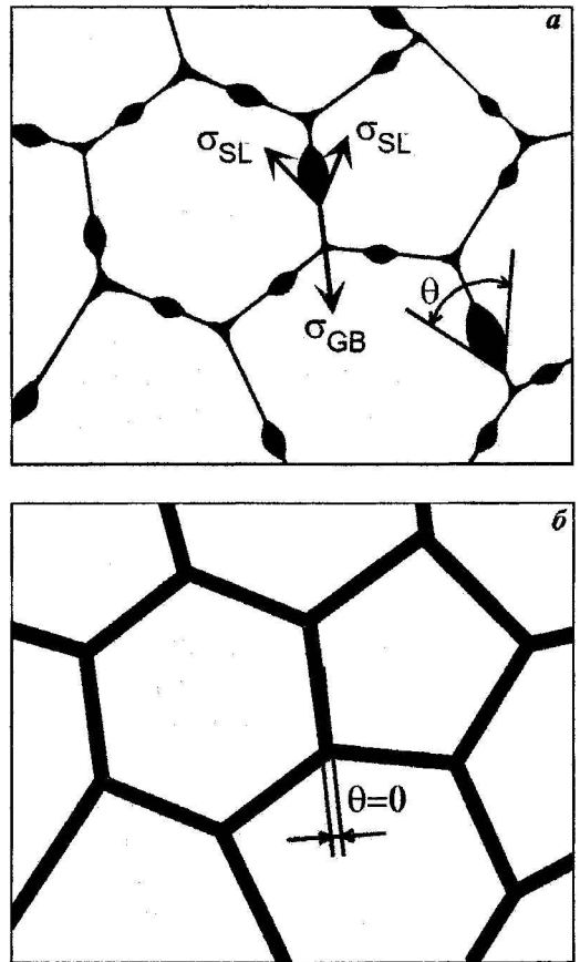
Рис. 1. Схематическое изображение поликристалла с границами зерен, частично (а) и полностью (б) смоченными второй фазой (показана на рисунке черным цветом)
