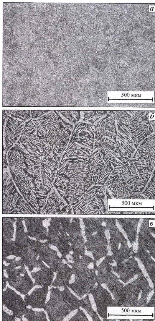
Рис. 2. Оптические микрофотографии сплава Ti—4мас.%Co
