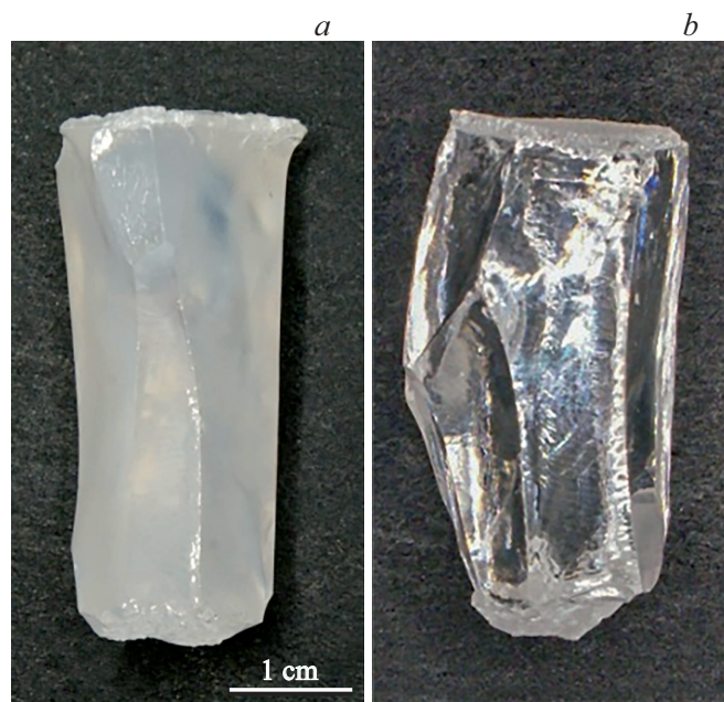
Рис. 1. Внешний вид кристаллов 8Sc1YbSZ (а) и 9Sc1YbSZ (b).
