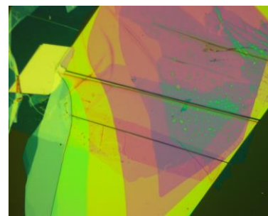
Рис.1. Структура hBN-WSe 2 -hBN на подложке Si/SiO 2 . Размер экрана 240х190 мкм 2 . Толщина нижнего слоя hBN, на который кладётся монослой WSe 2 , меняется ступеньками: 40-200-230-250-260 мкм.
