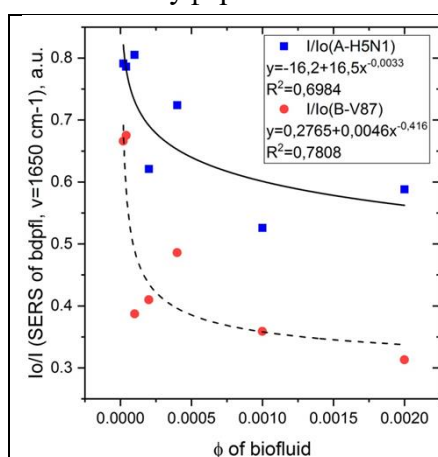
Рис. 1. Изменение относительной интенсивности SERS-сигнала метки BDPFL в зависимости от концентрации вирусных частиц гриппа А и В при агрегации в концентрированном соляном буфере.
