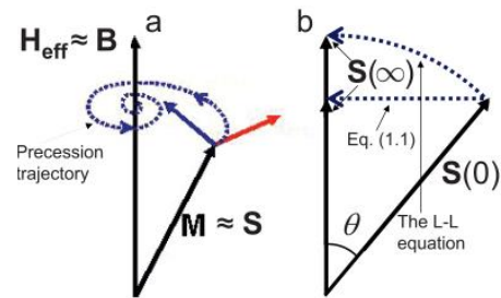
Рис. 1. Иллюстрация к уравнению движения магнитного момента \mathbf{S} в квантово-холловском ферромагнетике: \partial \mathbf{S} / \partial t = -(g\mu_B / \hbar) \mathbf{S} \times \mathbf{B} - \lambda_{QH} \mathbf{B} \times (\mathbf{S} \times \mathbf{B}) (а) Красная стрелка соответствует «прецессионному» члену в уравнении движения, синяя – затуханию. (б) Затухание (пунктирные линии) в системе отсчета, прецессирующей вместе с \mathbf{S} . Дуга – траектория, описывающая \mathbf{S}(t) согласно уравнению Ландау-Лифшица (L-L). Горизонтальная стрелка – направление движения момента в КХФ.
