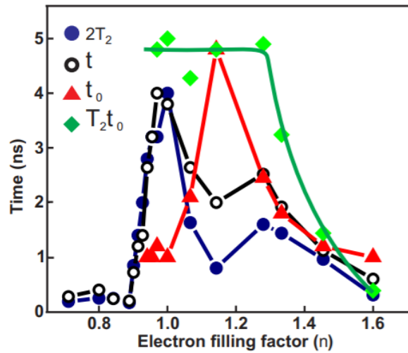
Рис.1. Качественный вид зависимости характеристических времен T_2 и t_0 от фактора заполнения 2ДЭС. Для сравнения показано эмпирическое время, при котором амплитуда ларморовских осцилляций уменьшается в e раз (точки).
