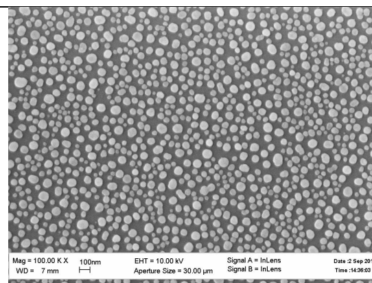
Рис.2. Изображение поверхности Si/SiO 2 , полученное на электронном микроскопе. Толщина напыленного серебра – 15 нм, температура отжига на твердотельной плитке – 360 °С, время отжига – 6 минут.
