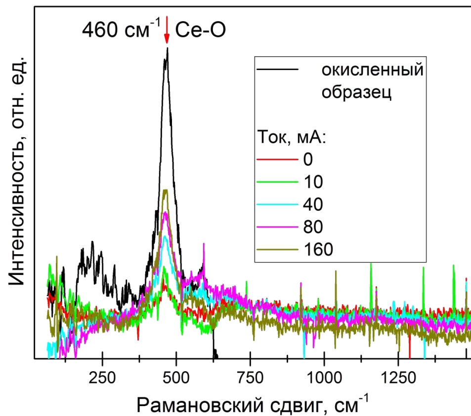
Изменения спектра КРС
