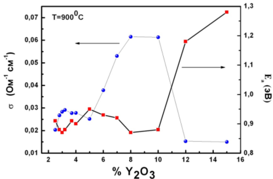
Зависимость проводимости ZrO_2-Y_2O_3 от концентрации Y_2O_3
