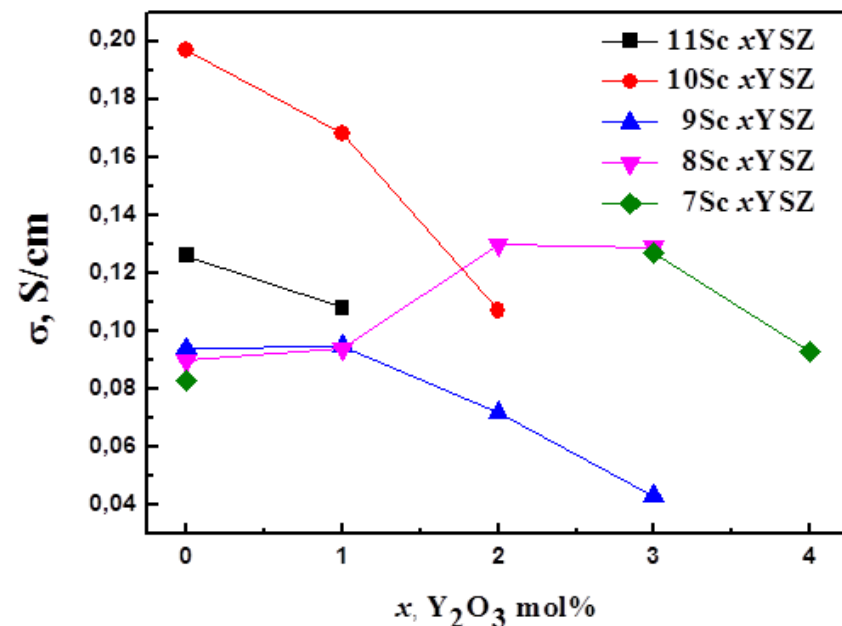
Зависимость проводимости твердых растворов (ZrO_2)_{1-x-y}(Sc_2O_3)_x(Y_2O_3)_y при температуре 900^\circ C от содержания Y_2O_3
