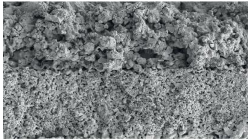
Изображение анодного электрода 5000x
